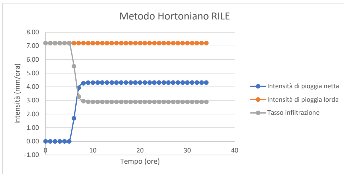
Figura 9. Intensità di pioggia e tasso di infiltrazione per il torrente Rile per T=200 anni e durata pari a 34 ore.
