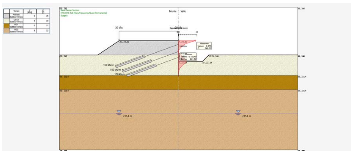
FIGURA 8.16: FASE 8: COMBINAZIONE RARA – DEFORMATA (MAX 8.07 MM)
