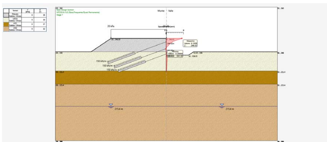
FIGURA 8.15: FASE 7: COMBINAZIONE RARA – DEFORMATA (MAX 8.13 MM)
