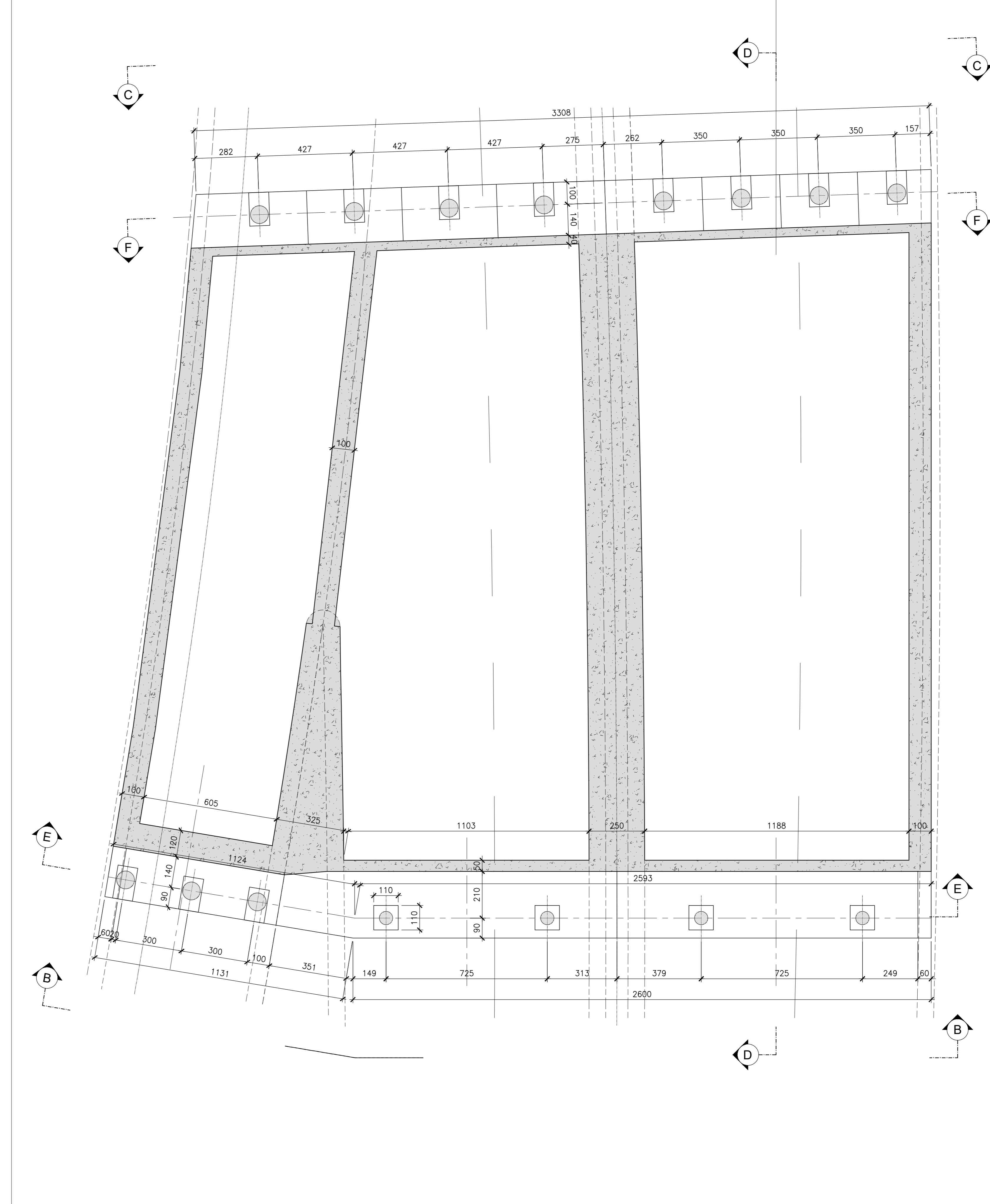
SEZIONE ORIZZONTALE SUL PARAGHIAIA SCALA 1:100
