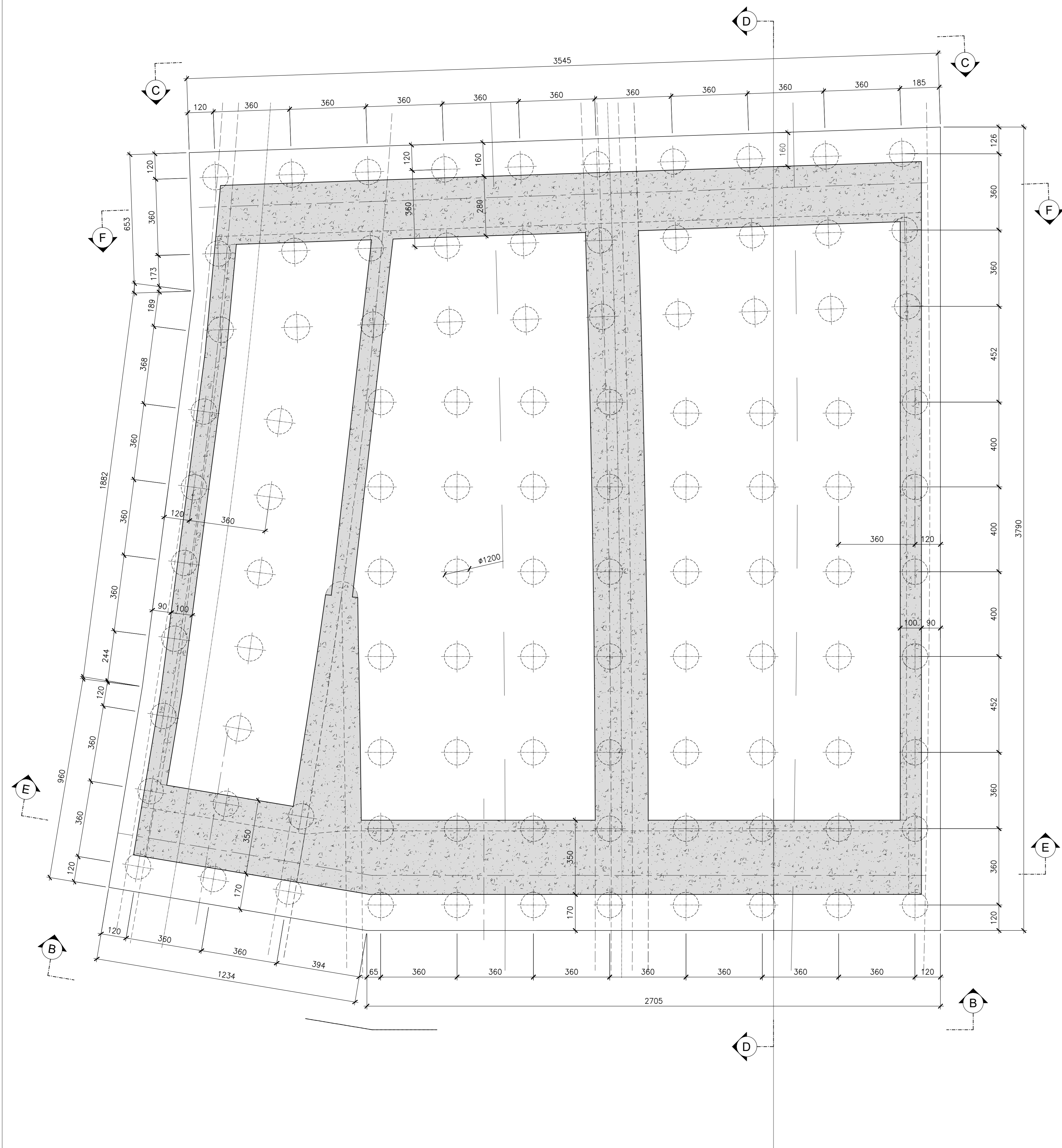
SEZIONE ORIZZONTALE A-A SCALA 1:100
