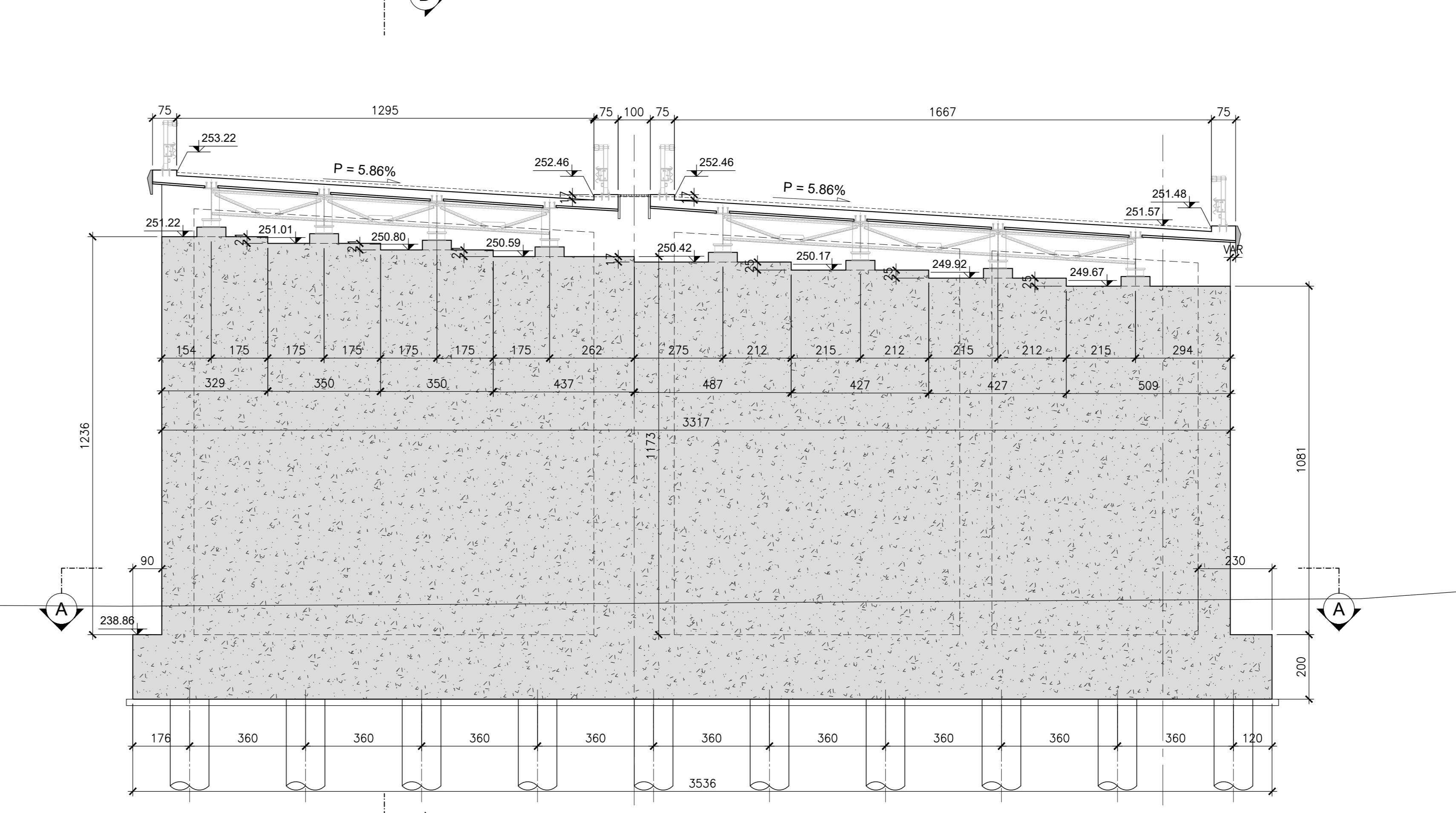
SEZIONE TRASVERSALE F-F (ASSE APPOGGIO) SCALA 1:100
