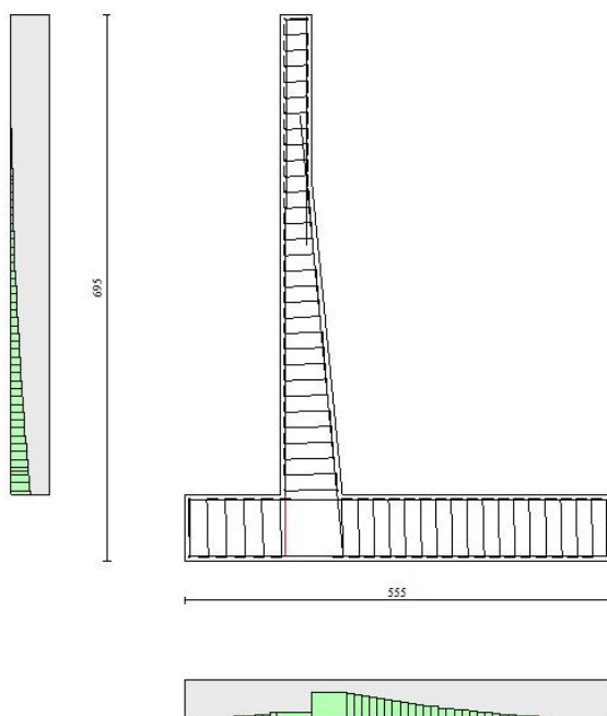
Fig. 17 - Paramento (Inviluppo)
