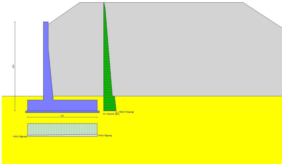
Fig. 4 - Diagramma delle pressioni (combinazione statica) (Combinazione n° 1)
