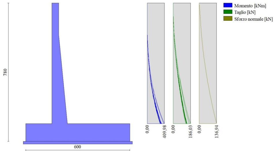
Fig. 15 - Paramento
