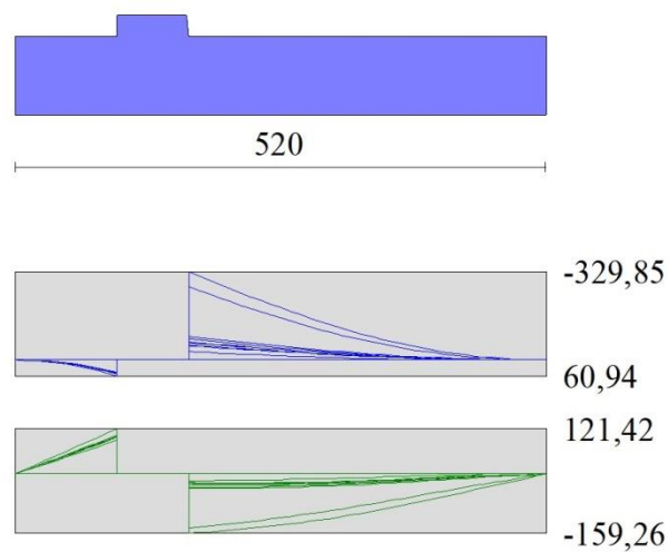
Fig. 16 - Fondazione
