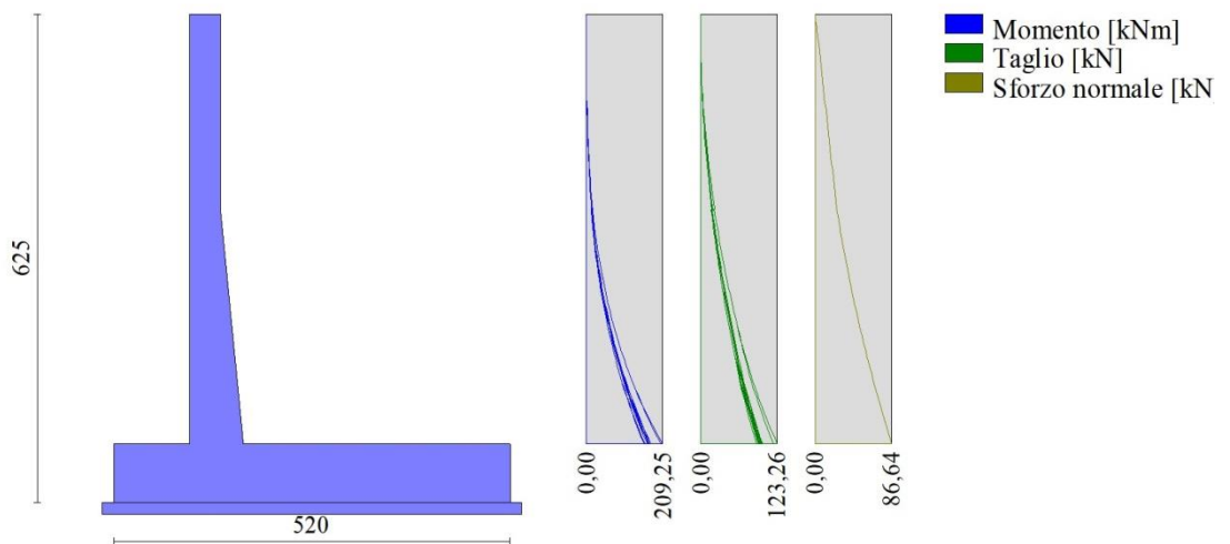
Fig. 15 - Paramento
