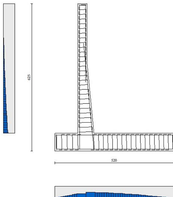
Fig. 18 - Paramento (Inviluppo)
