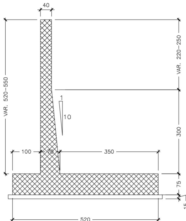
I.8 Sezione trasversale CONCIO C
