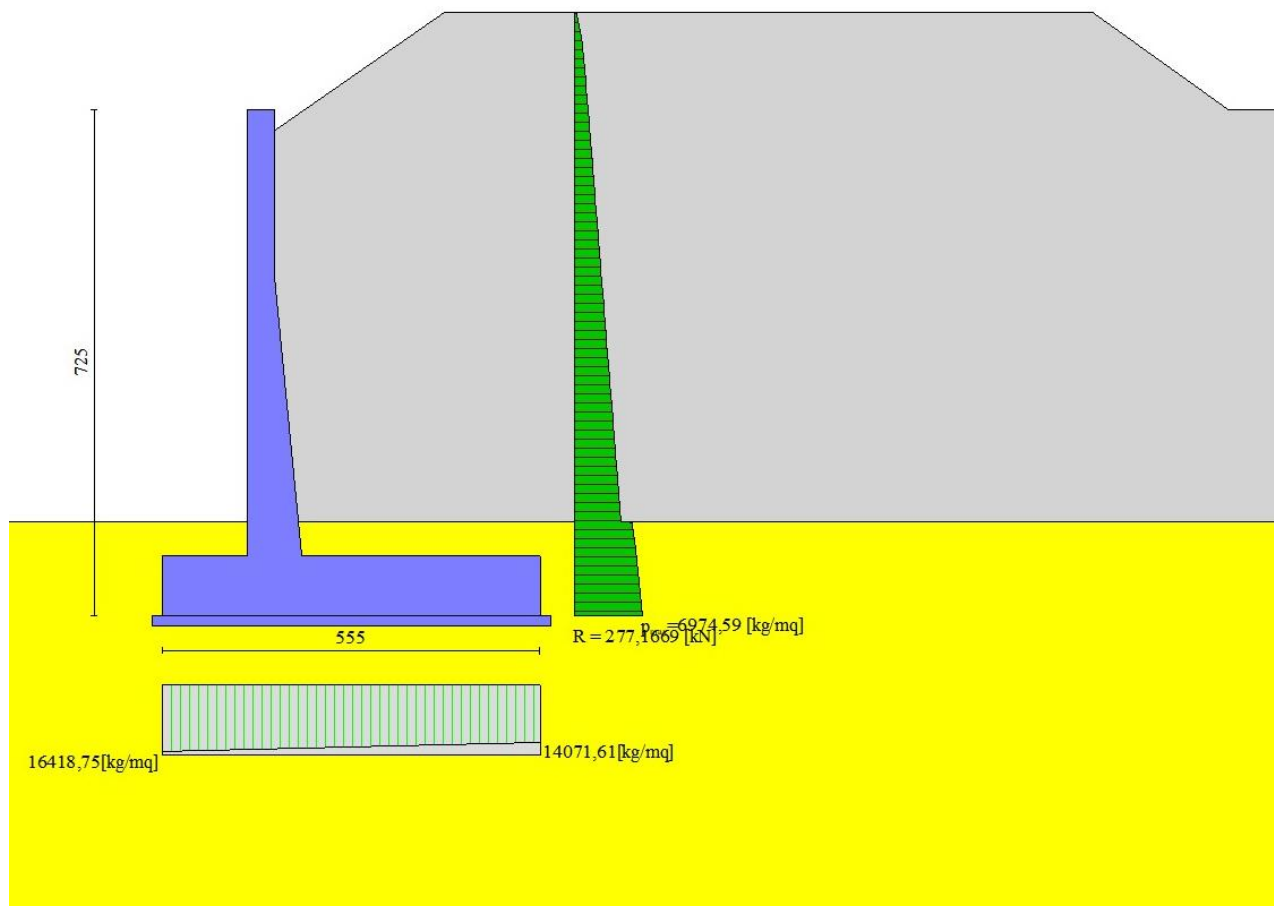
Fig. 4 - Diagramma delle pressioni (combinazione statica) (Combinazione n° 1)
