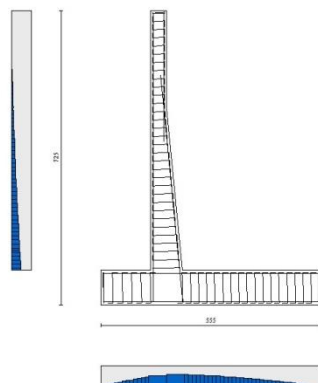
Fig. 18 - Paramento (Inviluppo)
