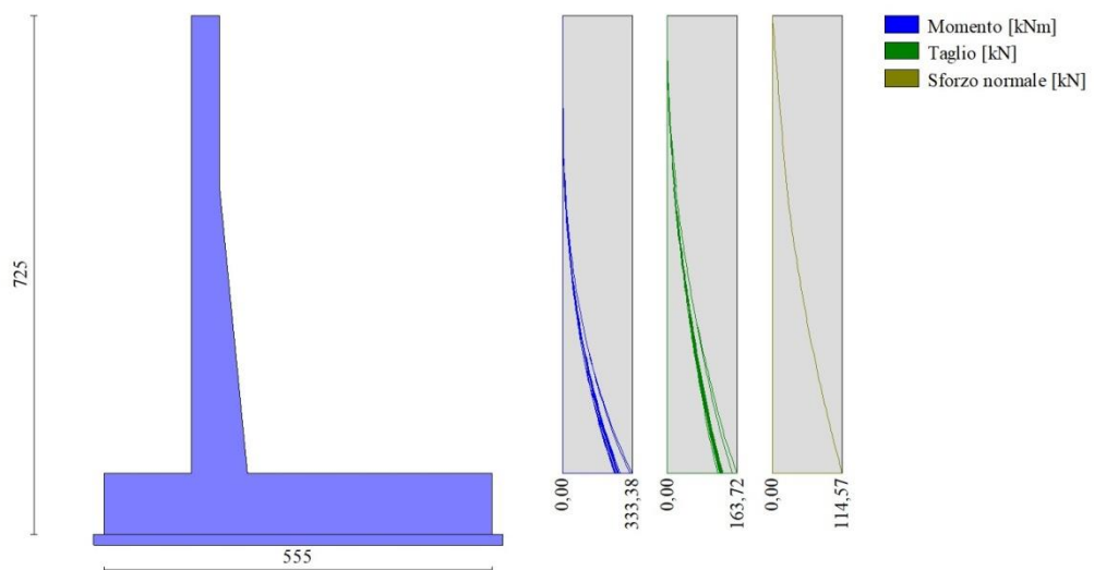
Fig. 15 - Paramento
