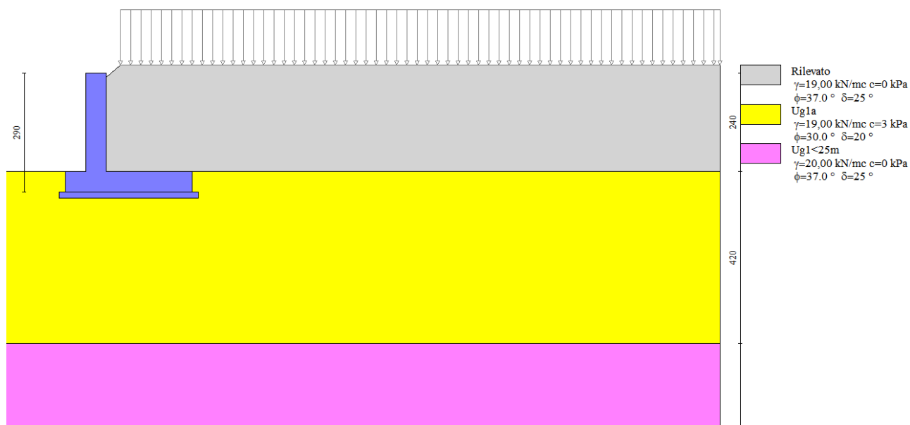
Fig. 2 - Stratigrafia
