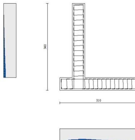
Fig. 18 - Paramento (Inviluppo)
