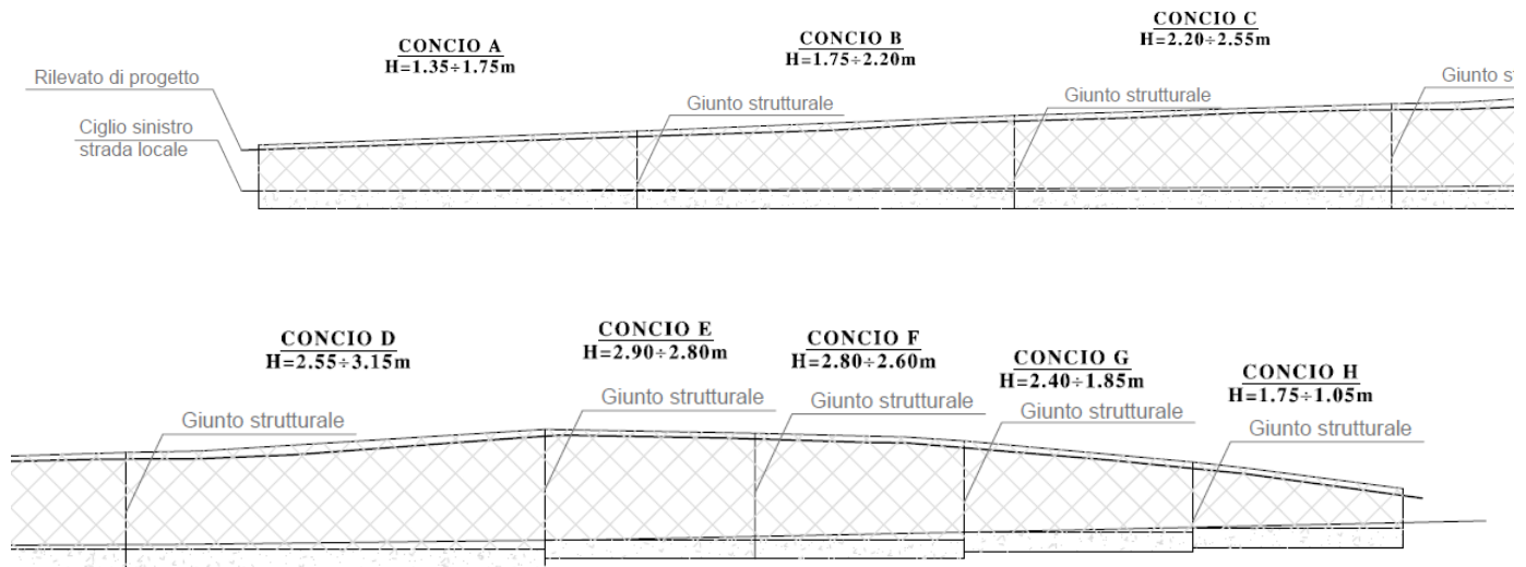
1.2 Sezione longitudinale muro di sostegno OS72
