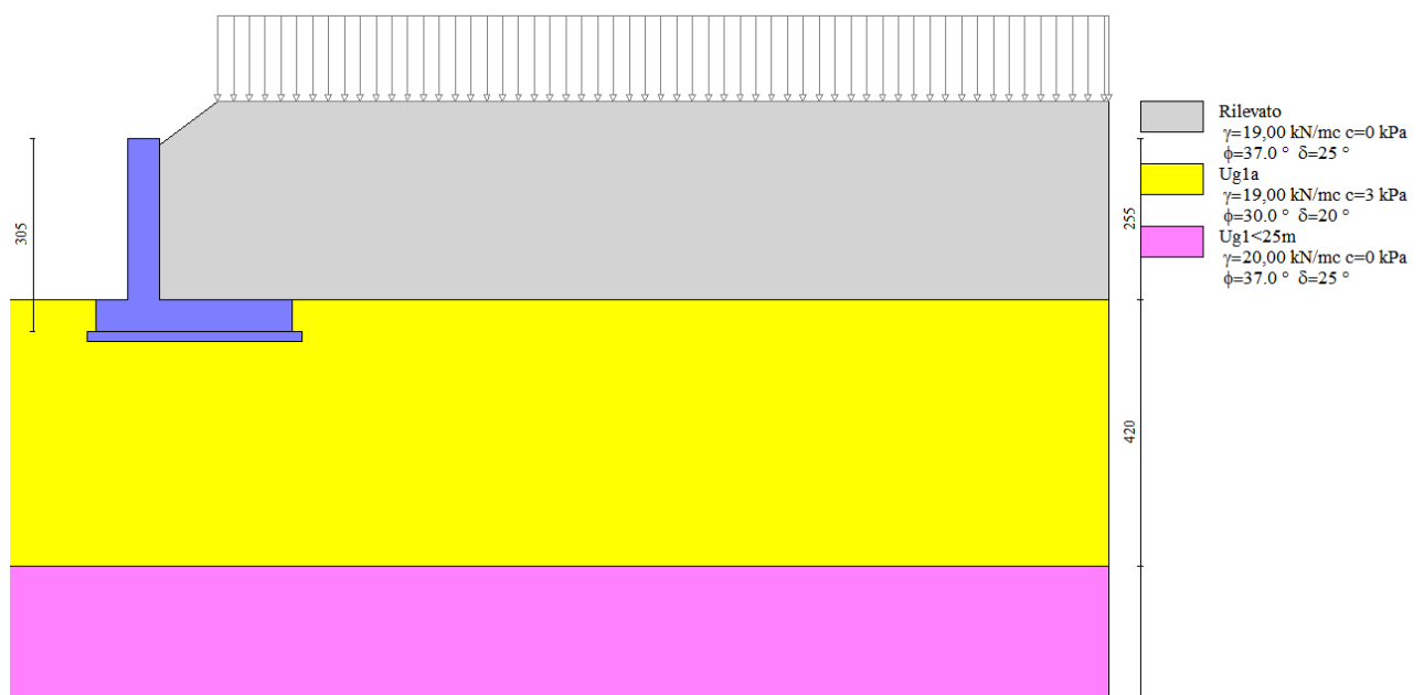
Fig. 2 - Stratigrafia
