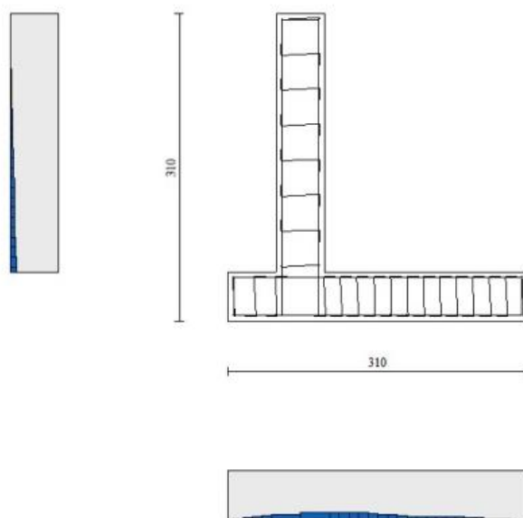
Fig. 18 - Paramento (Inviluppo)
