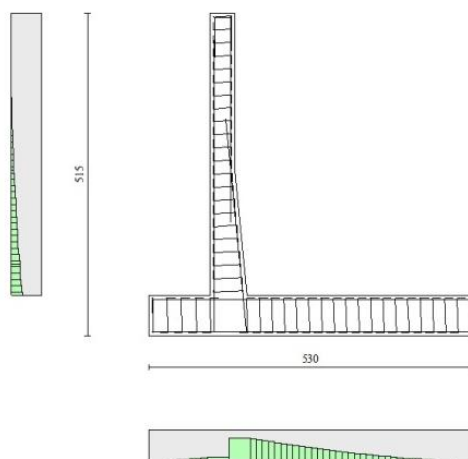
Fig. 17 - Paramento (Inviluppo)
