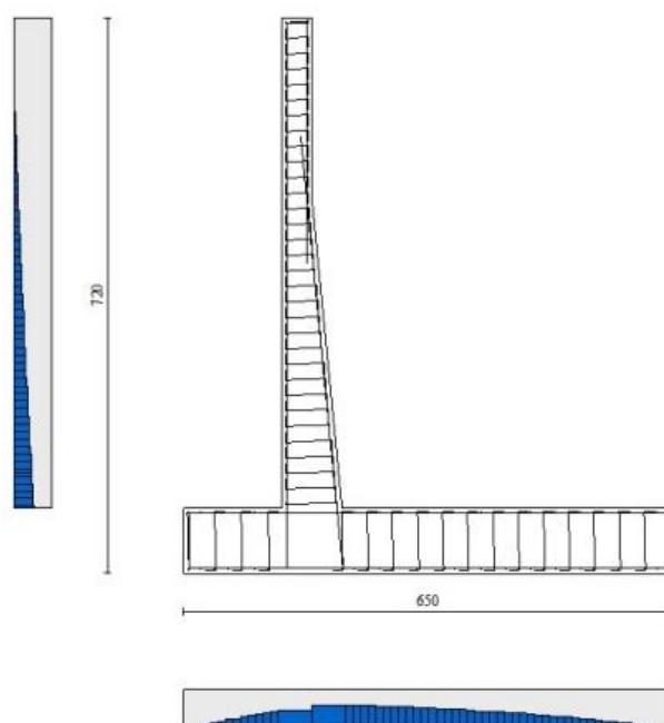
Fig. 18 - Paramento (Inviluppo)
