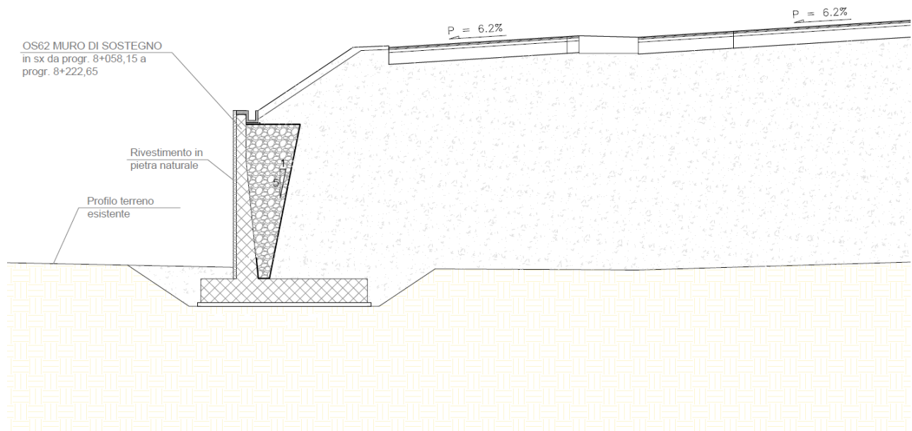
I.3 Sezione trasversale - muro di sostegno OS62
