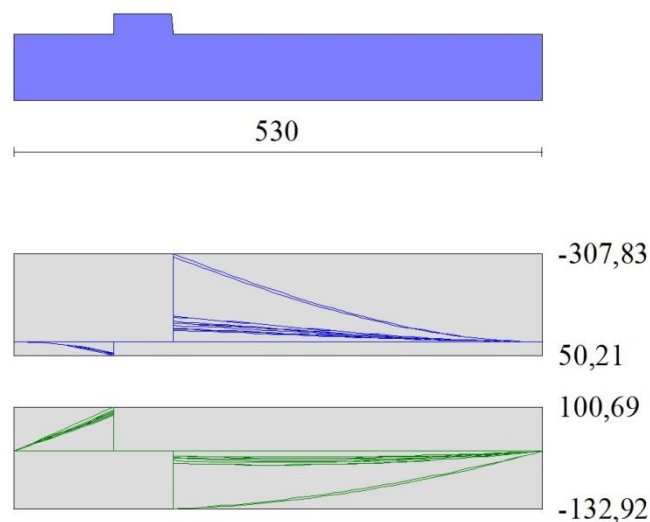
Fig. 16 - Fondazione
