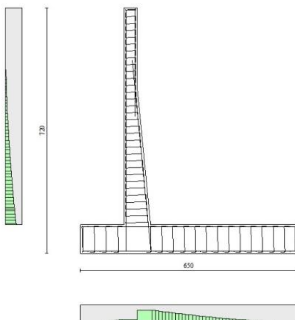
Fig. 17 - Paramento (Inviluppo)
