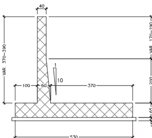
I.10 Sezione trasversale CONCIO E
