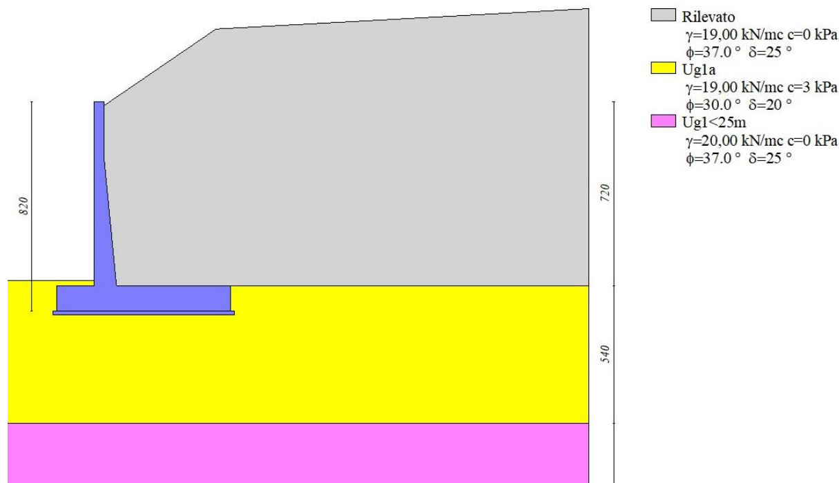
Fig. 2 - Stratigrafia
