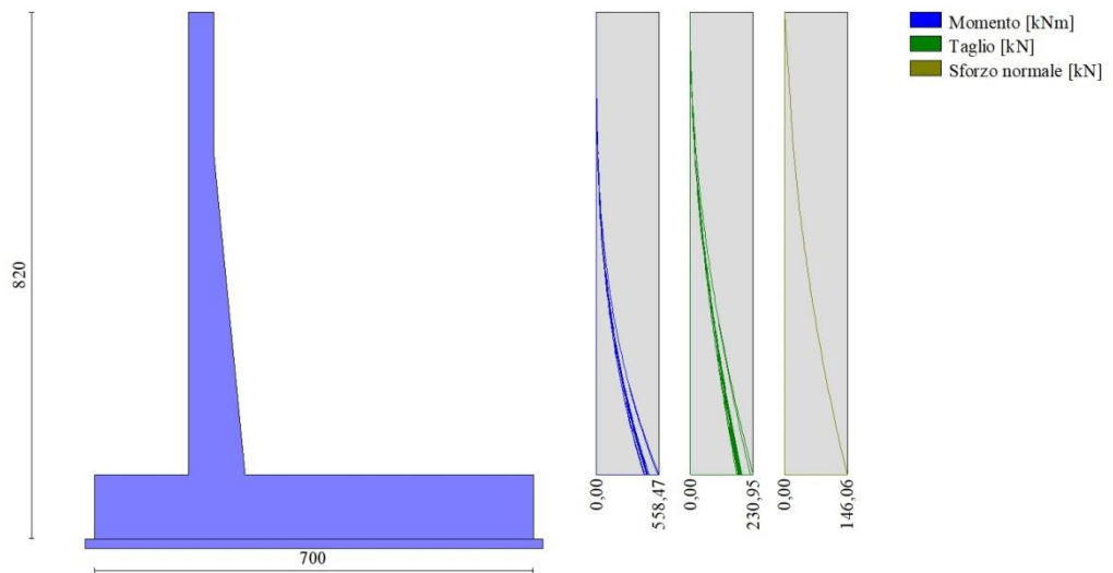
Fig. 15 - Paramento
