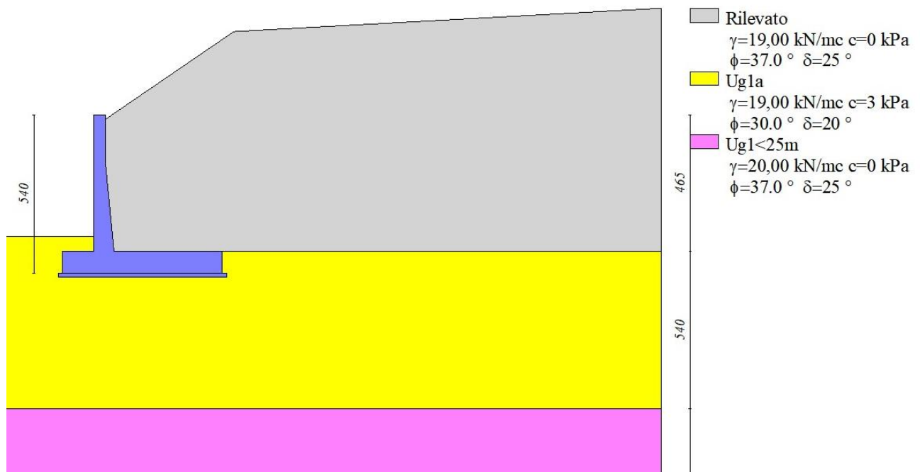
Fig. 2 - Stratigrafia
