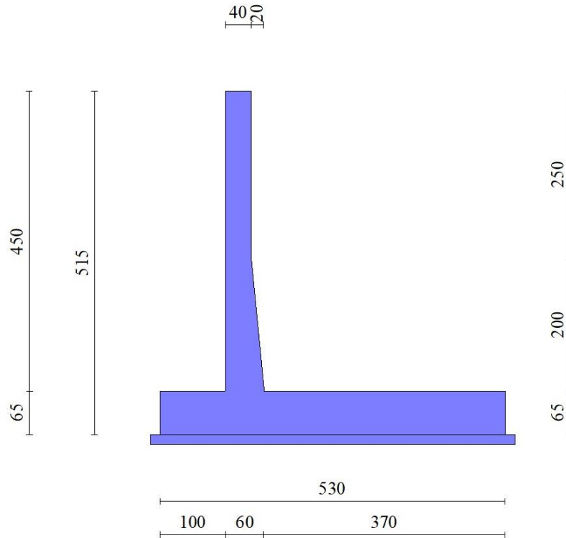
Fig. 1 - Sezione quotata del muro
