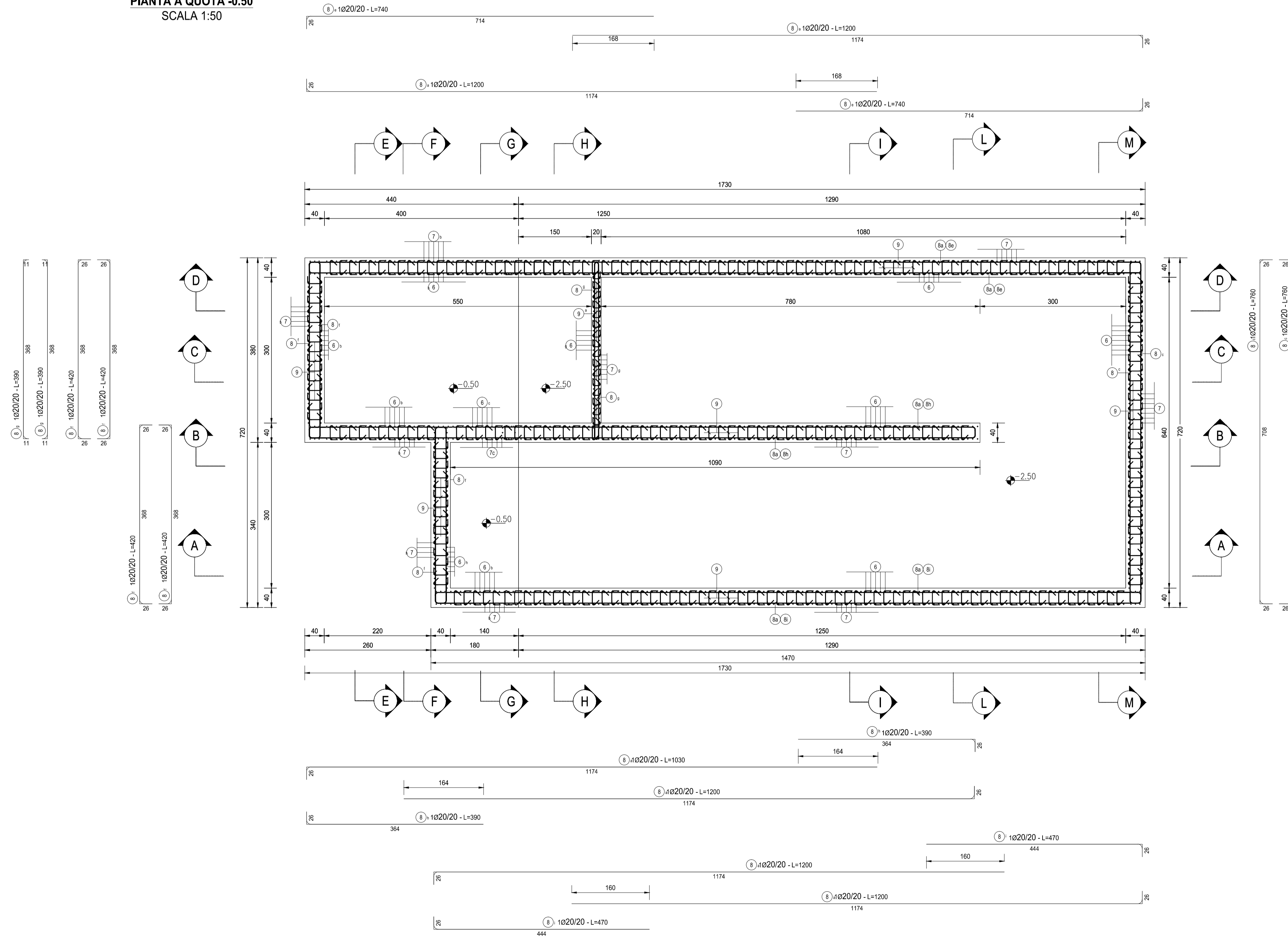
PIANTA A QUOTA -0.50 SCALA 1:50
