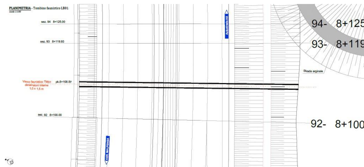
I.1 Inquadramento planimetrico – Sottopasso faunistico
