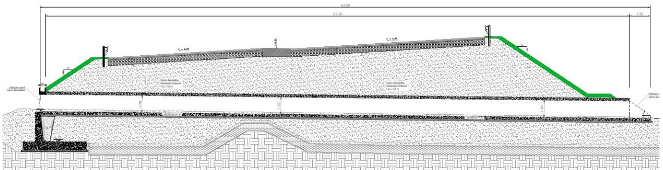
1.2 Sezione longitudinale - Sottopasso faunistico
