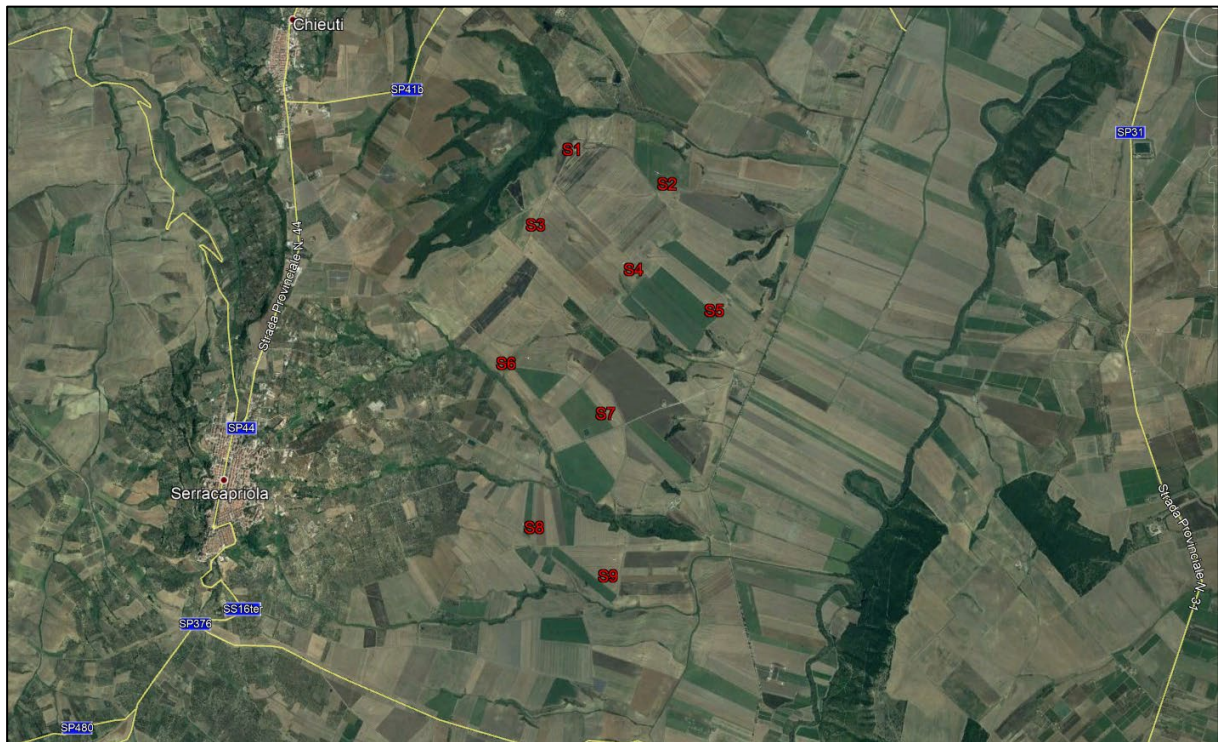
Figura 1: inquadramento territoriale generale dell'area di progetto su orto foto piana estratta da Google Earth.
