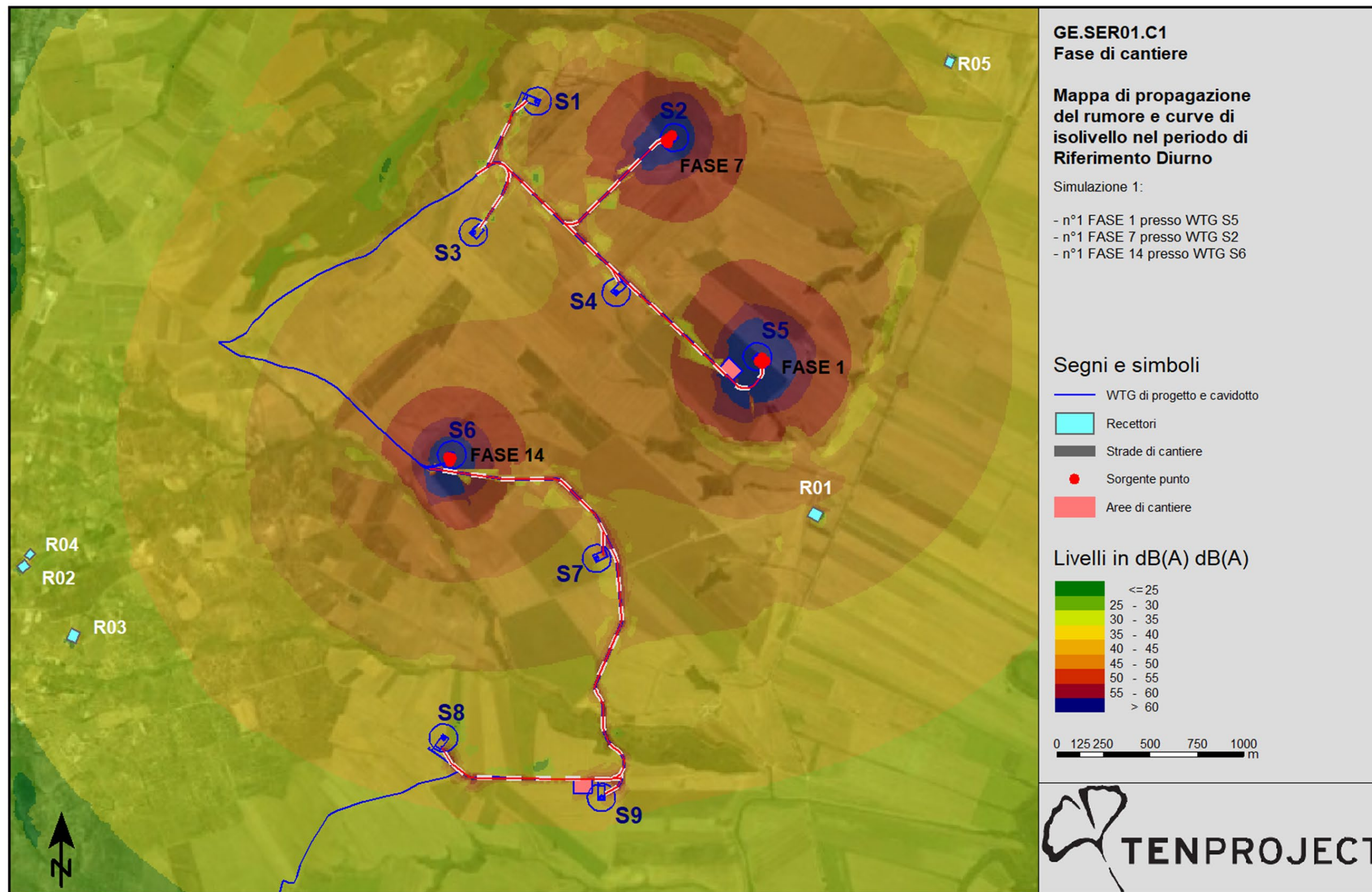
MAPPA DI PROPAGAZIONE DEL RUMORE – SIMULAZIONE 1
