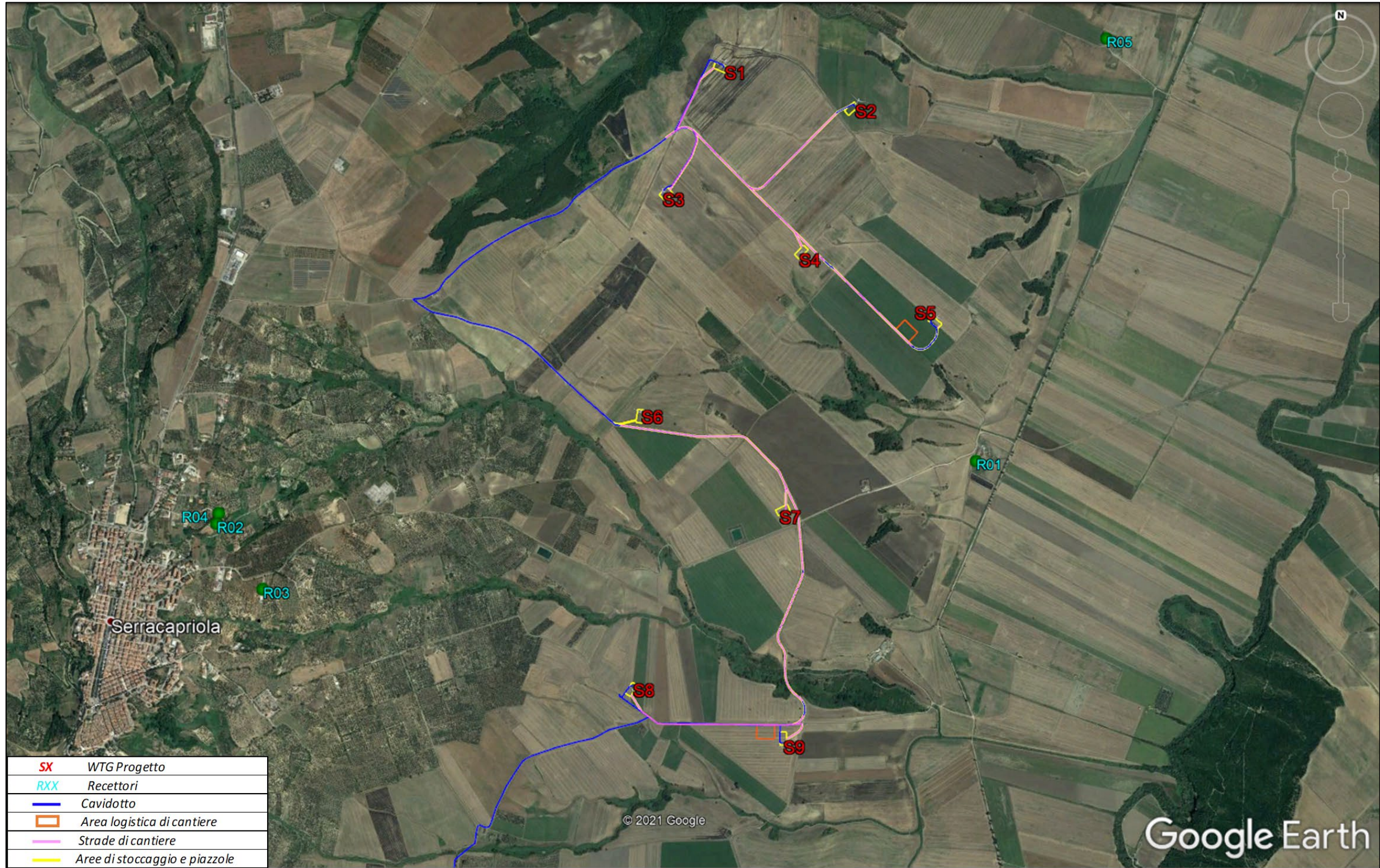
Figura 5: Caratterizzazione dell'area di sviluppo futuro dell'impianto su ortofoto estratta da Google Earth.
