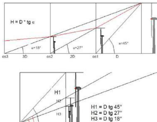
Figura 51: Sensibilità visiva in funzione della distanza
