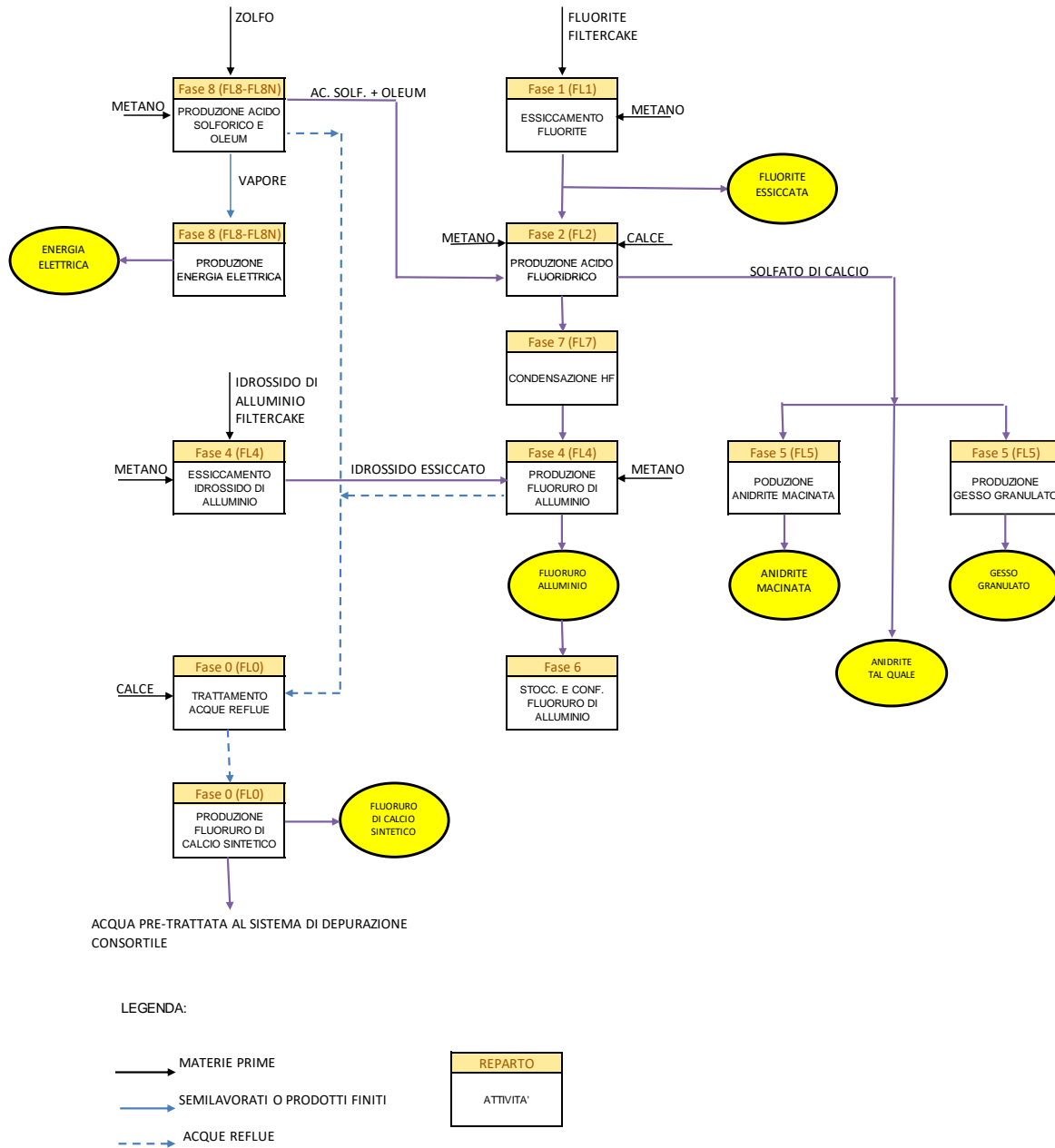
Figura 1: Diagramma di flusso delle attività Fluorsid
