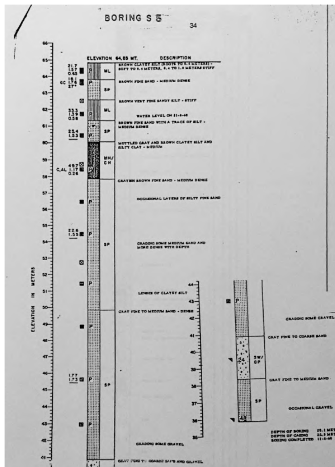
Figura 4-41: Stratigrafia del sondaggio n. 5 (Boer, 1993)
