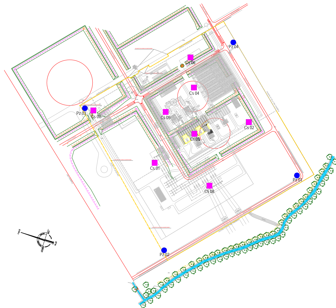
Fig.2 – Pianta dell'area destinata alla costruzione della Centrale a Ciclo Combinato a Turano Lodigiano con l'ubicazione dei punti di campionamento dei terreni e delle acque sotterranee
