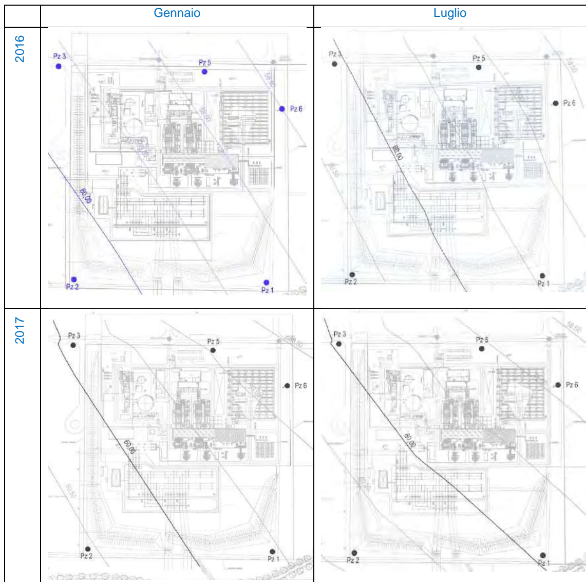
Figura 4-43: Carta delle isofreatiche (2016-2018) –Sorgenia Power
