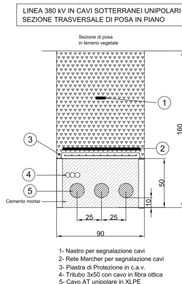
Figura 3-7: Schema tipico di posa dei cavi interrati della linea 380 kV di collegamento alla stazione Terna
