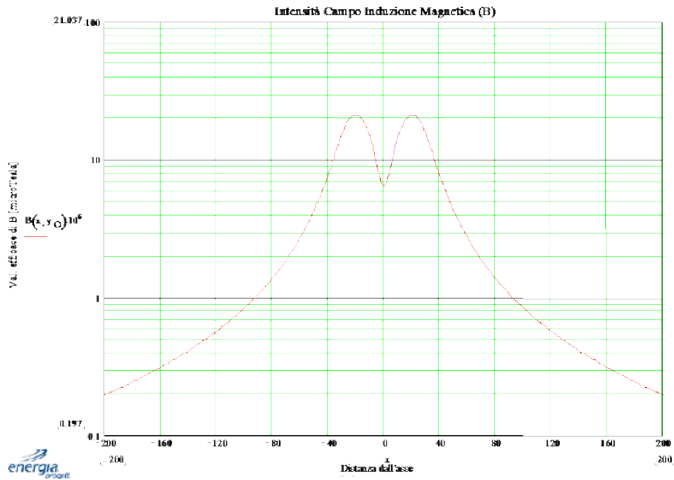
Figura 4-76: – Campo magnetico a 1 m dal suolo per linea entra esce – Centrale fuori produzione e massimo transito di corrente sulle linee (1500 A)
