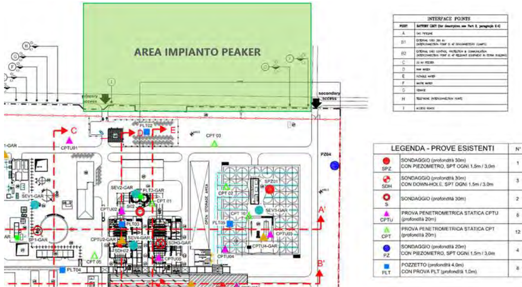
Figura 4-45: Ubicazione dei sondaggi campagna di indagine 2008
