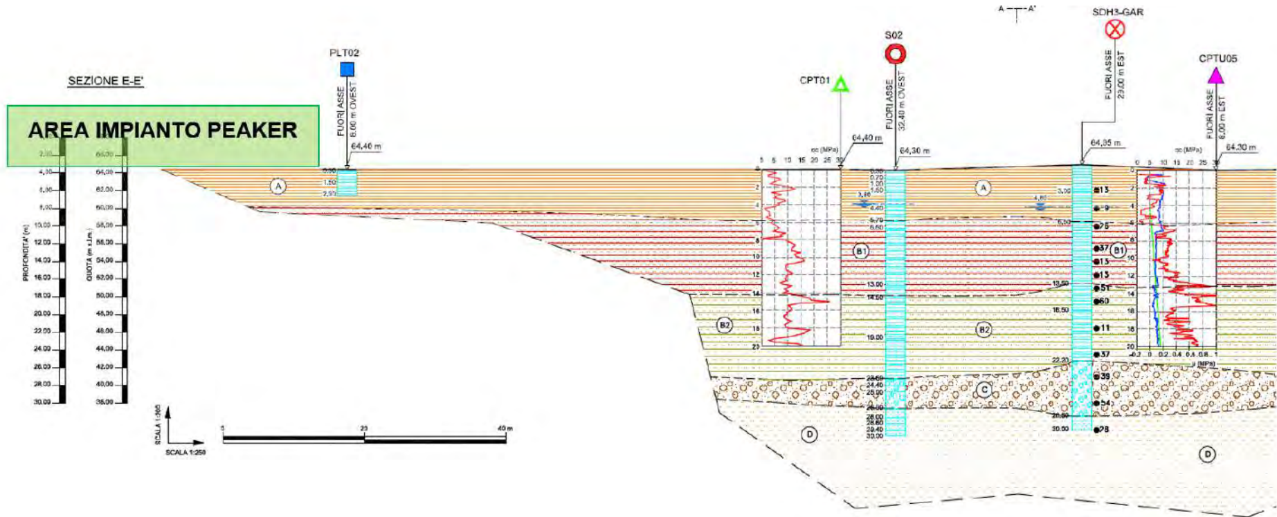
Figura 4-46: dettaglio stratigrafico Sezione E-E'
