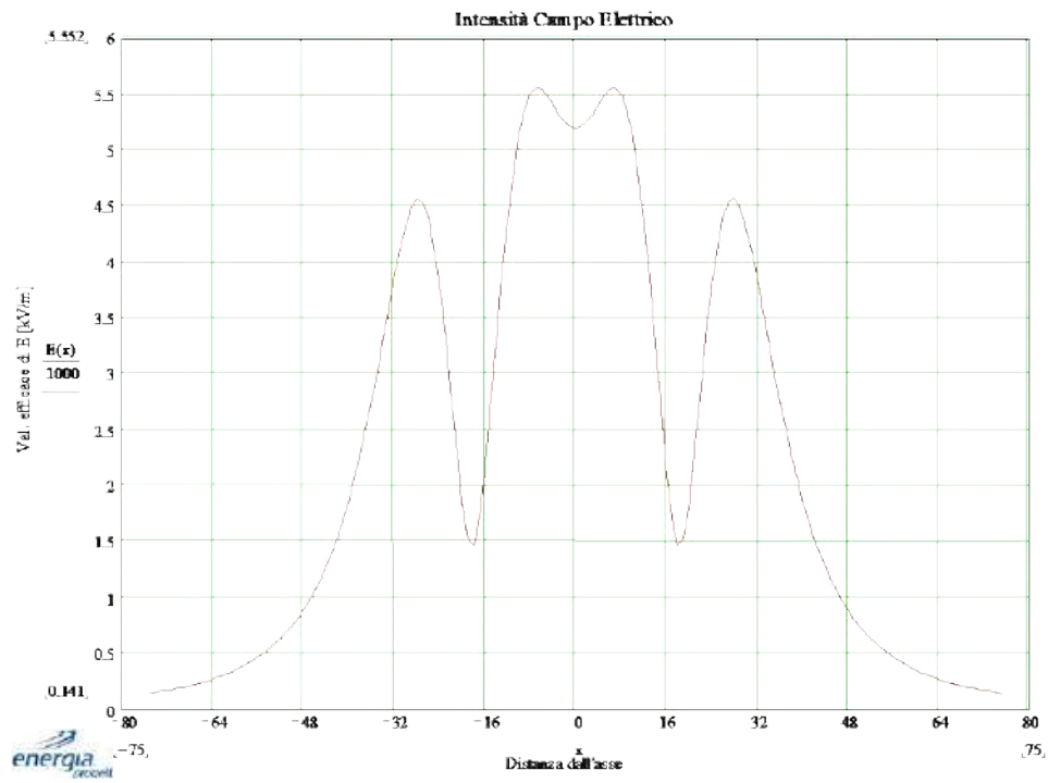
Figura 4-77: – Campo elettrico a 1 m dal suolo per linea entra esce
