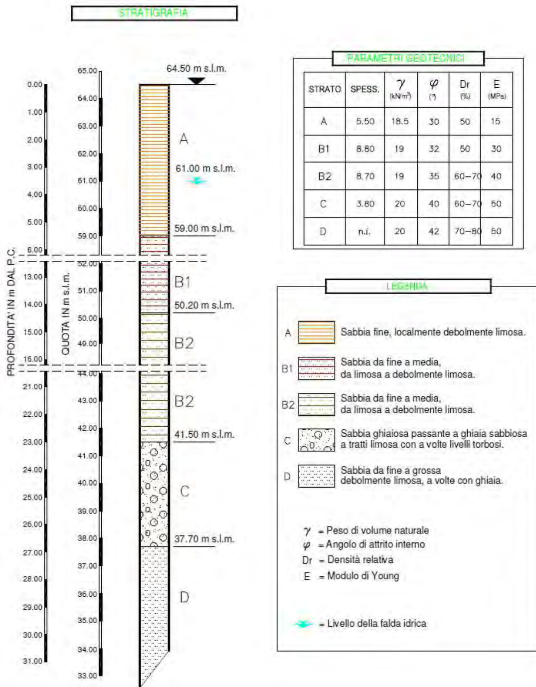
Figura 4-42: Stratigrafia di progetto per l'area (Ansaldo Energia, 2008)
