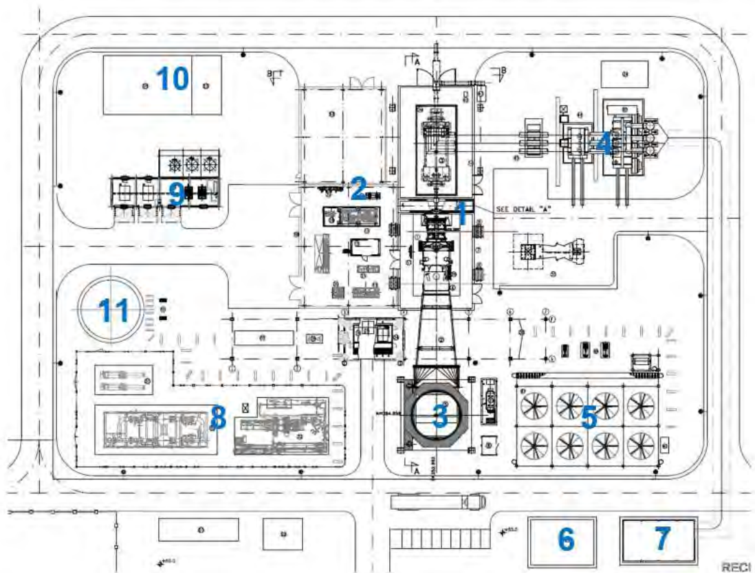
Figura 3-4: Planimetria generale dell'impianto in progetto
