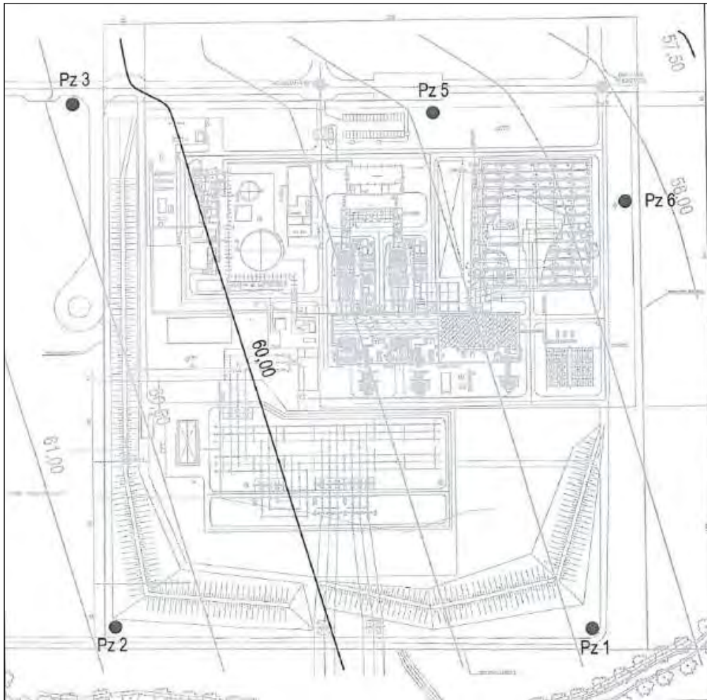
Figura 4-49: Localizzazione dei punti di monitoraggio delle acque (PMC Centrale di Lodi)
