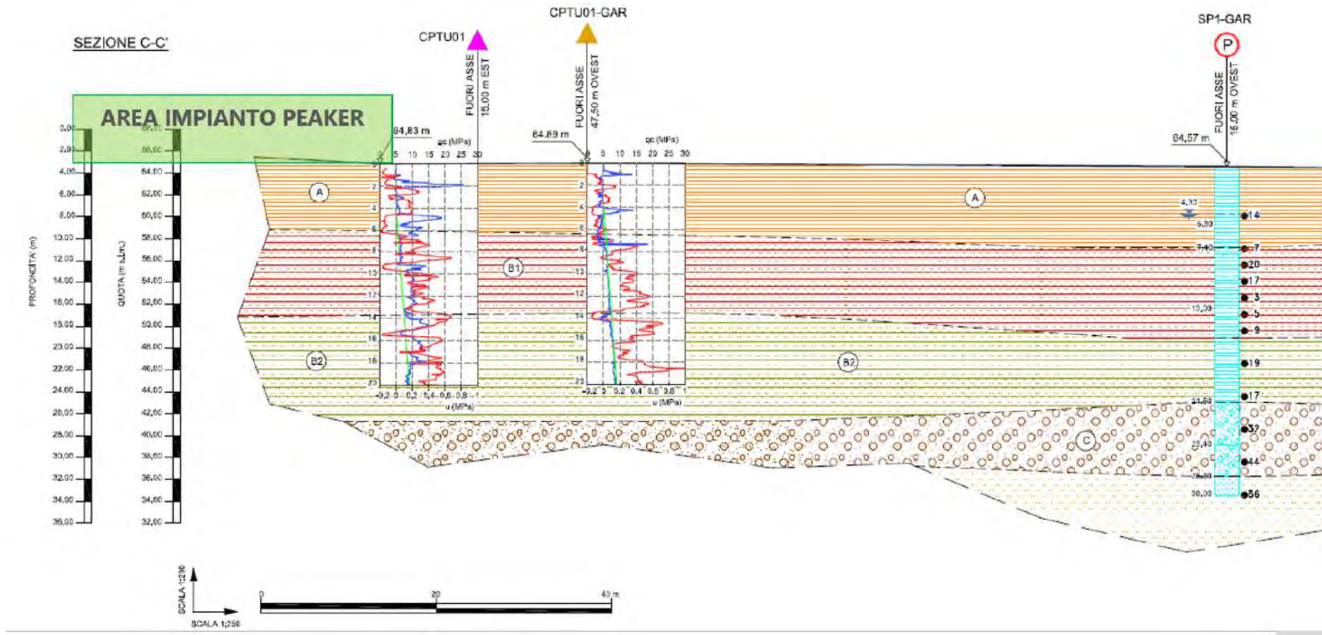
Figura 4-47: dettaglio stratigrafico Sezione C-C'
