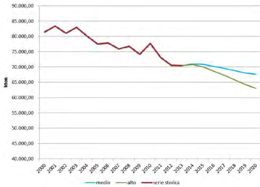
Figura 2-9: Scenari PEAR di riduzione delle emissioni di CO2
