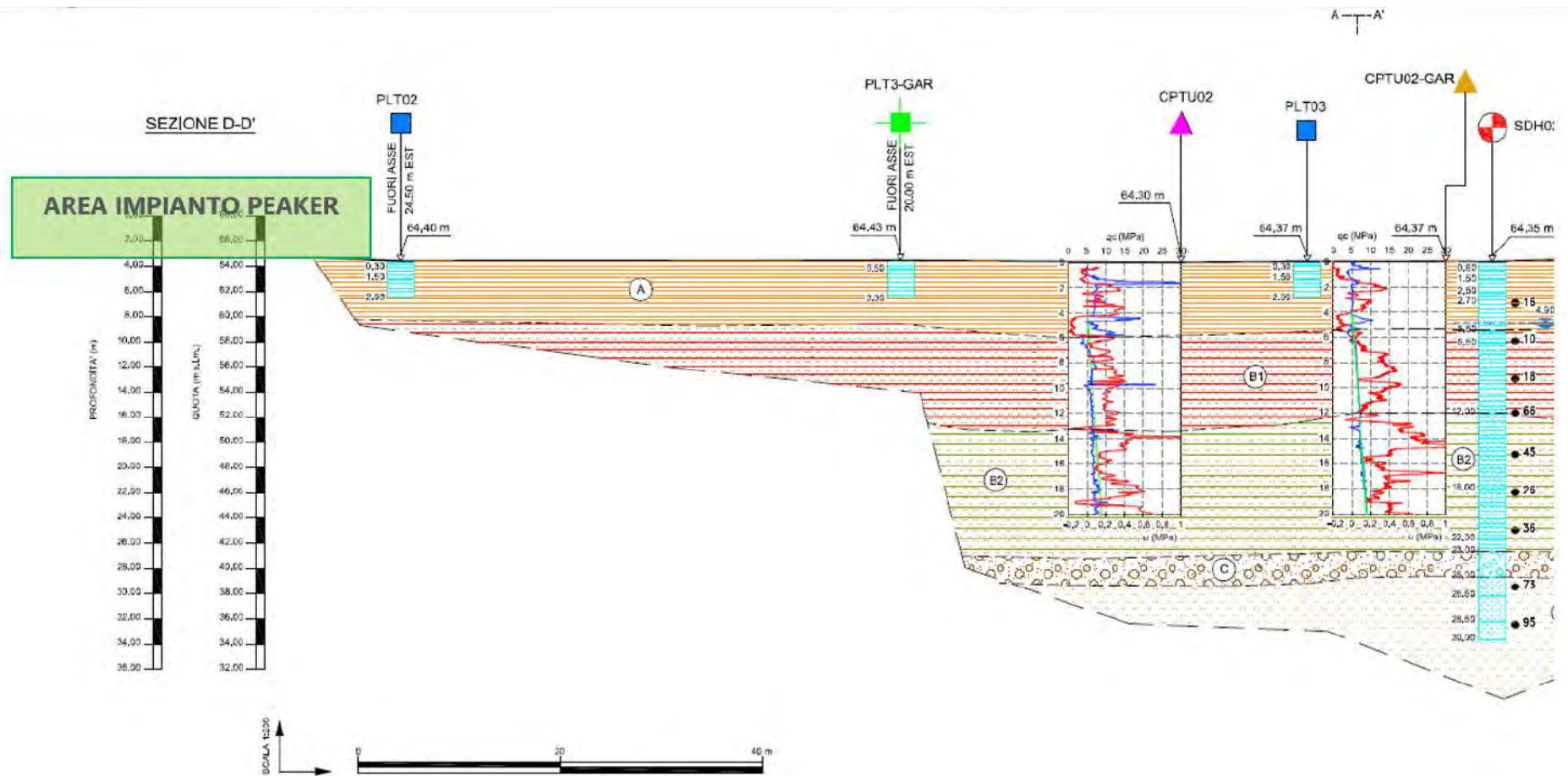
Figura 4-48: dettaglio stratigrafico Sezione D-D'
