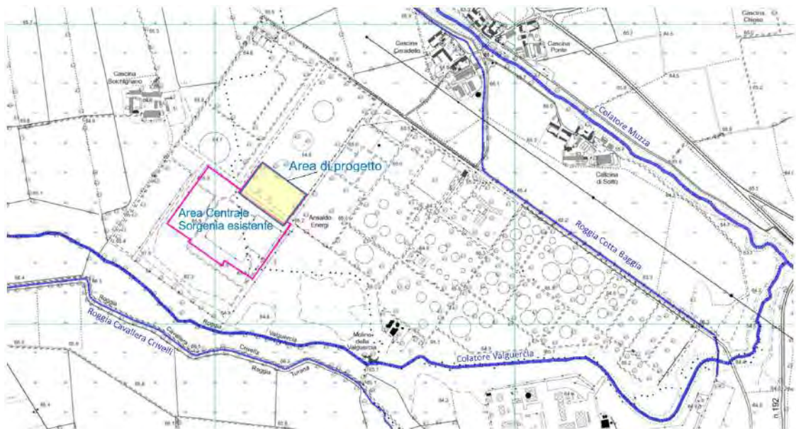
Figura 4-56. Estratto CTR dell'area del nuovo Impianto Peaker in progetto, con evidenziato il reticolo idrico
