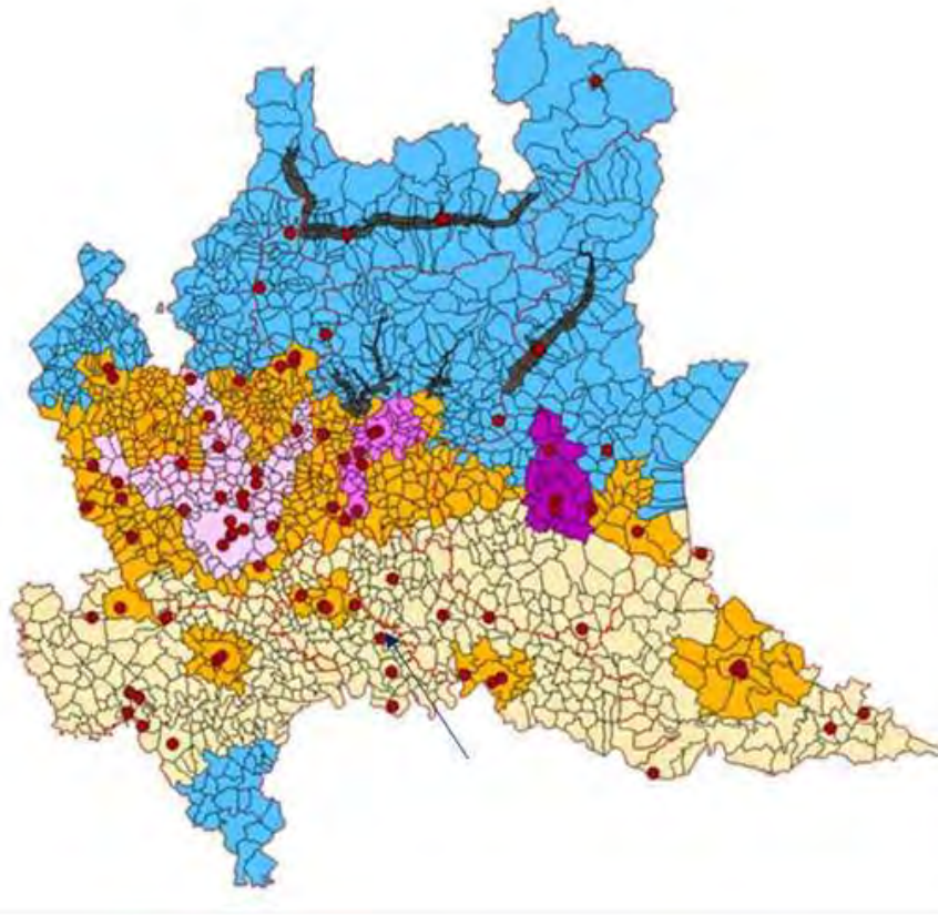
Figura 2-39: Rete regionale di monitoraggio della qualità dell'aria
