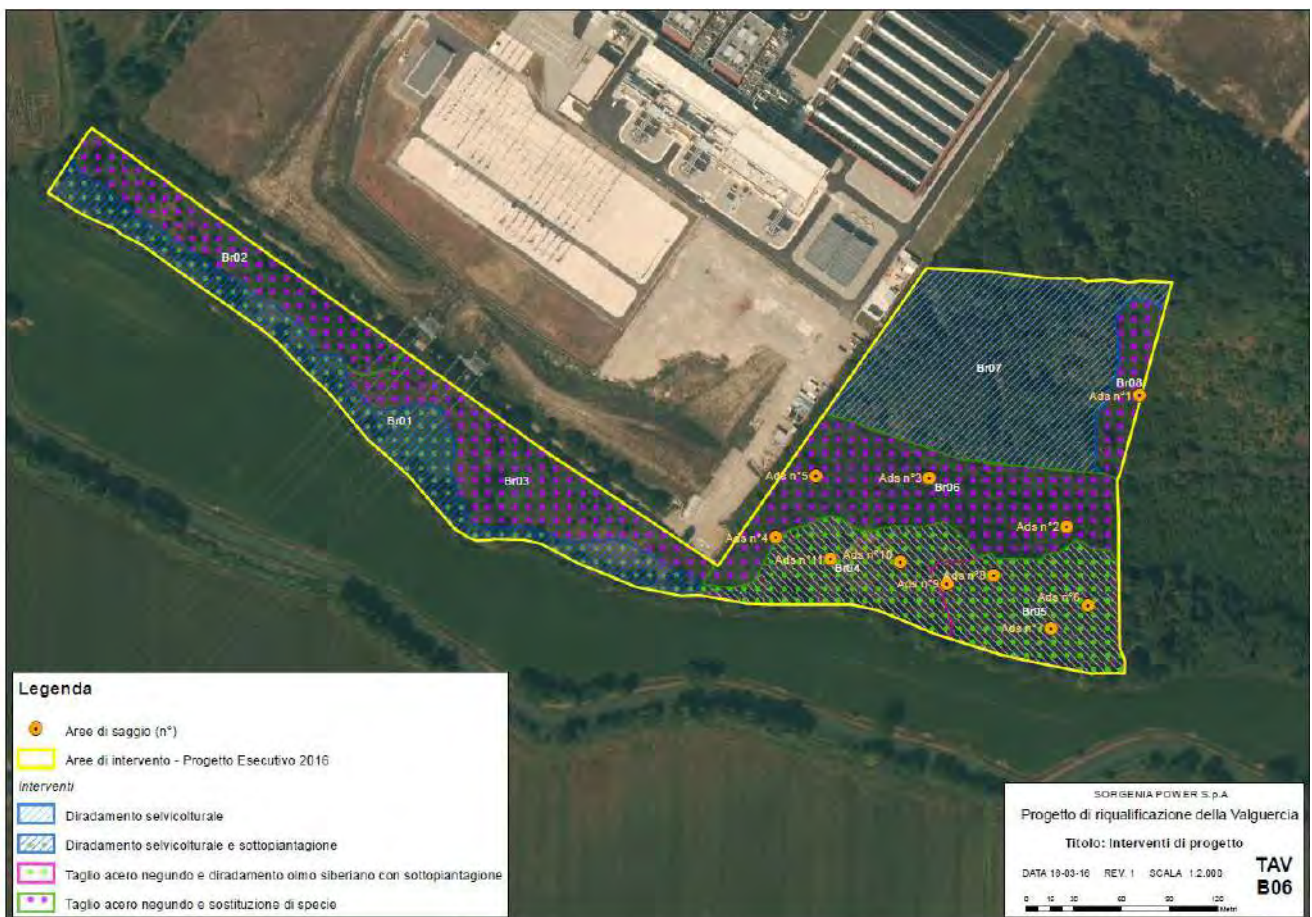
Figura 2-25: Estratto tavola di progetto di riqualificazione della Valguercia (dott. For. R. Musmeci)
