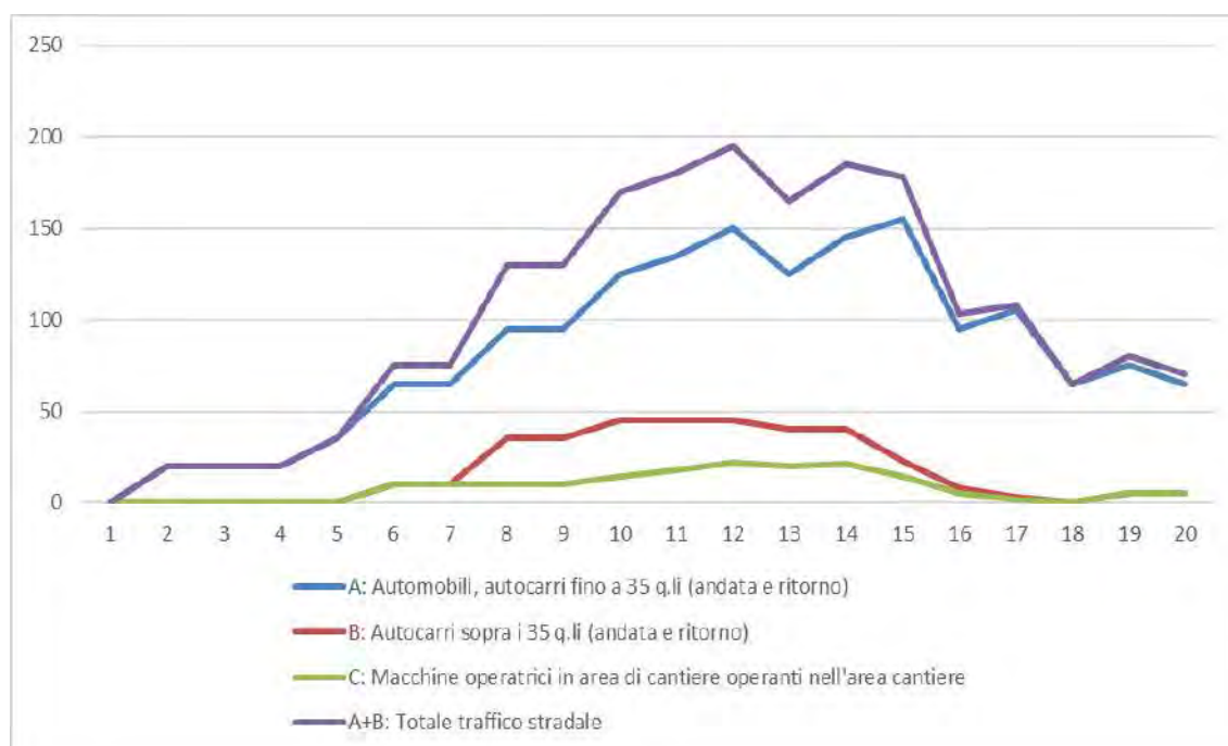
Figura 3-13: Grafico del traffico medio giornaliero atteso in fase di cantiere
