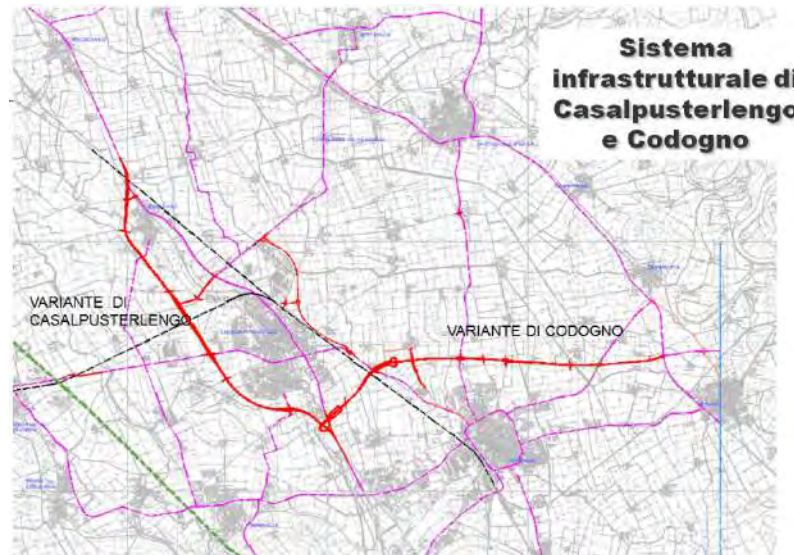
Figura 4-79: Schema progettuale delle tangenziali di Casalpusterlengo e Codogno (Fonte Provincia di Lodi) attualmente in fase di autorizzazione
