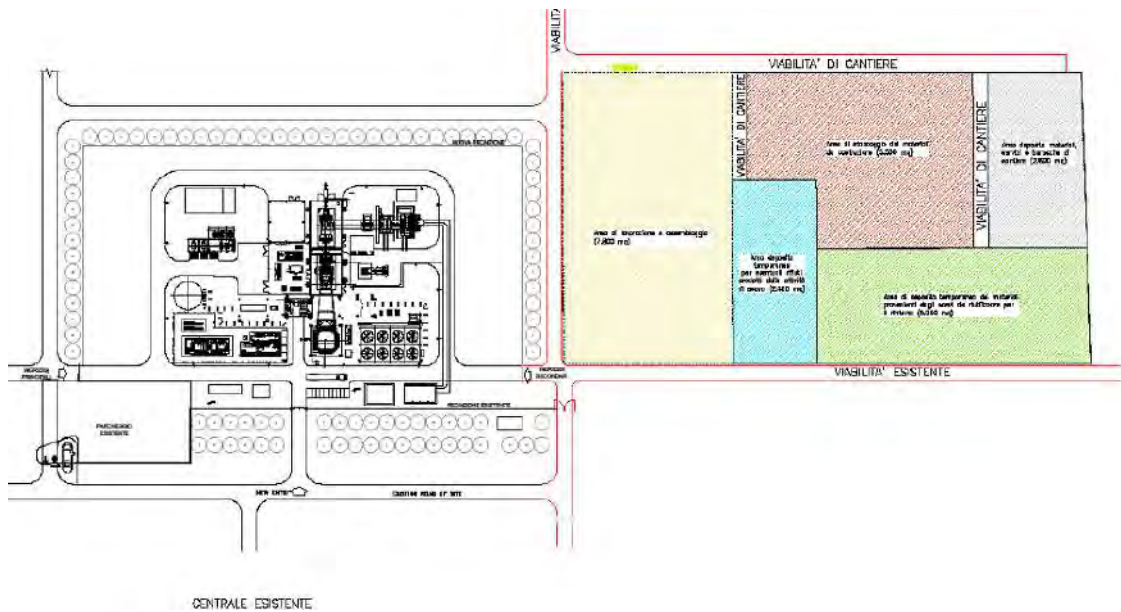
Figura 3-12: Localizzazione dell'area di cantiere temporaneo adiacente al sito di progetto
