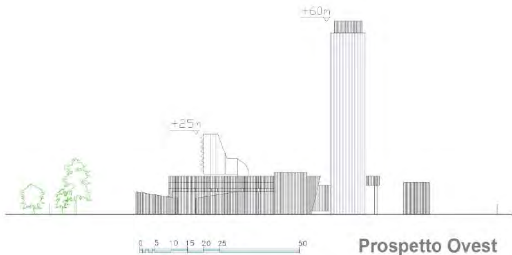
Figura 3-9: Sistemazione architettonica – prospetto ovest
