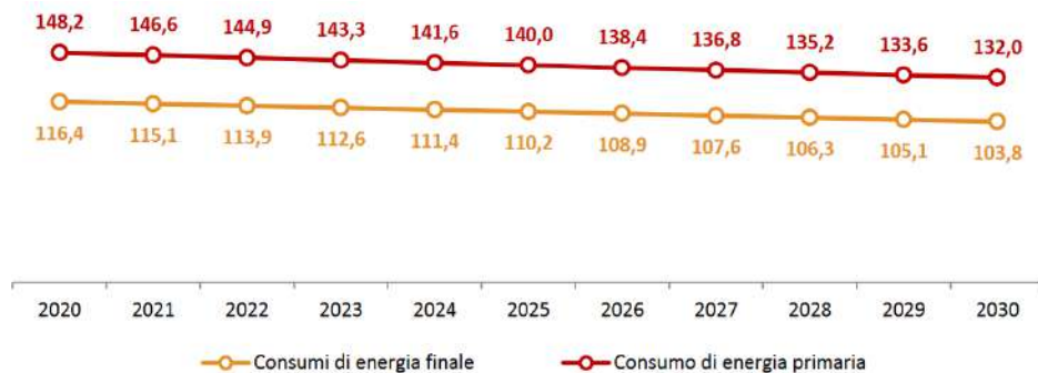
Figura 2-4: Traiettorie dei consumi di energia primaria e finale (Mtep) nel periodo 2020-2030
