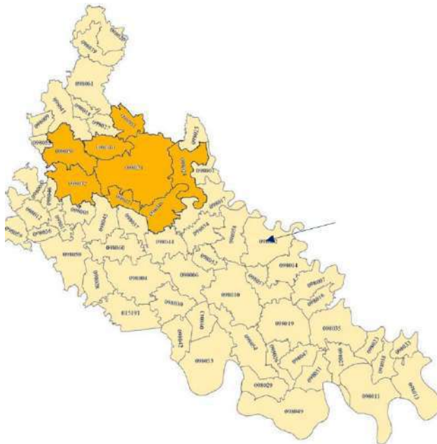
Figura 2-38: Zonizzazione del territorio regionale (estratto provincia di Lodi)
