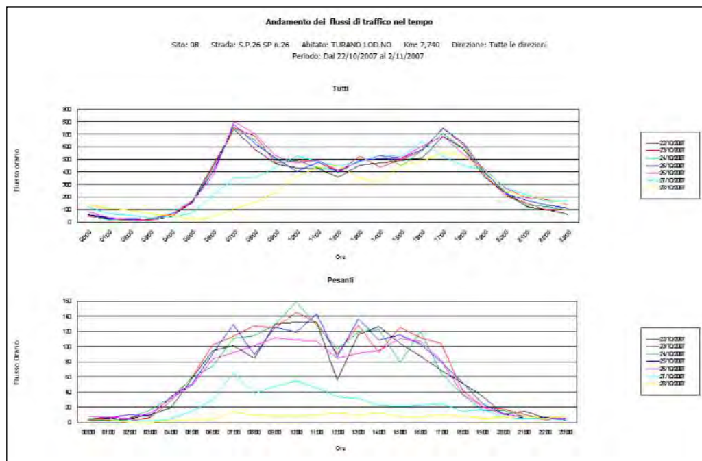
Figura 4-81: Flussi di traffico presso la postazione SP 26 Turano lodigiano km 7,74 – entrambe le direzioni (fonte Provincia di Lodi)
