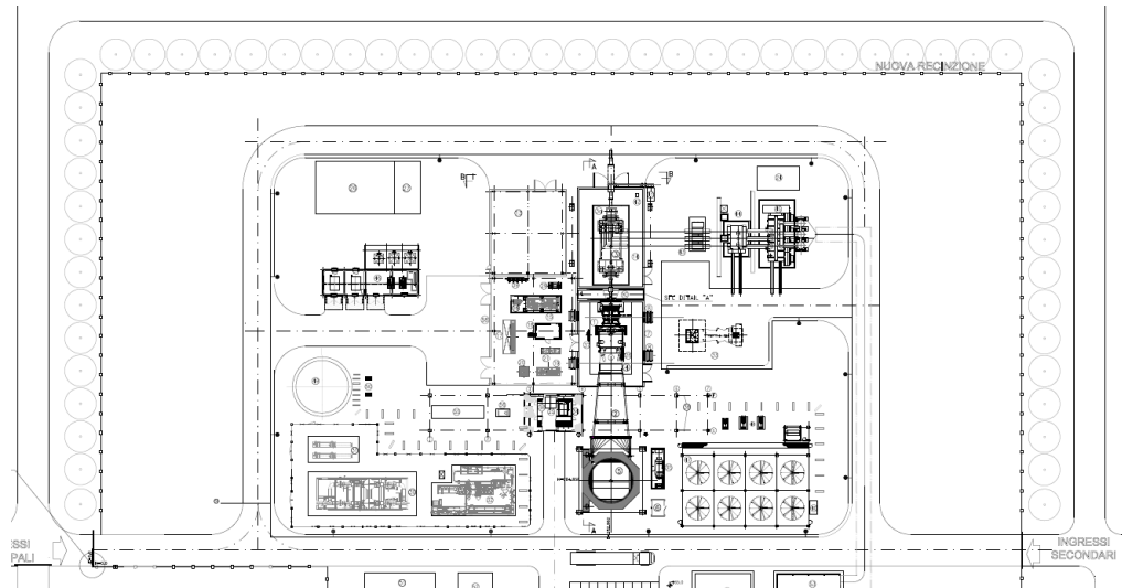
Figura 5. planimetria generale dell'impianto.
