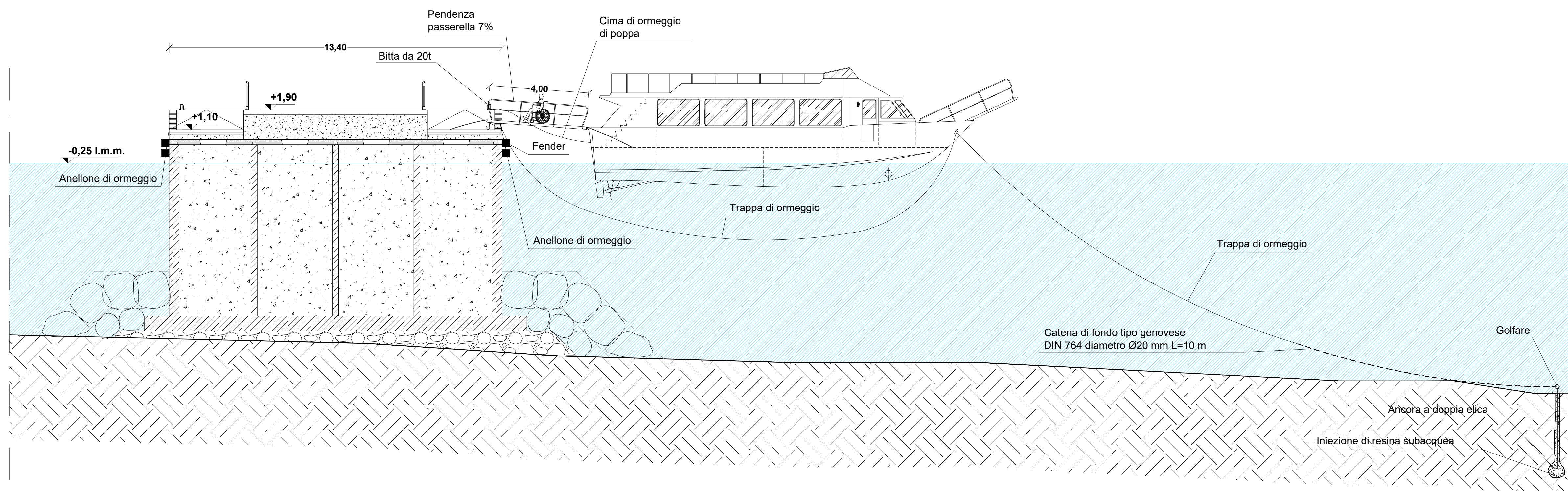
SEZIONE B2-B2 A LIVELLO MINIMO -0,25 m (Scala 1:100)
