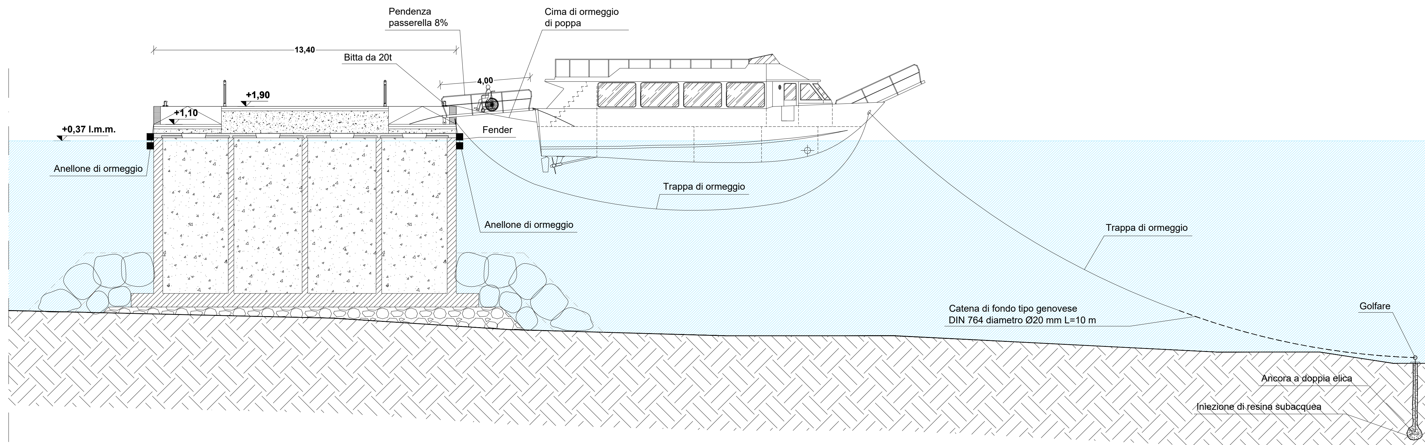
SEZIONE B2-B2 A LIVELLO MASSIMO +0,37 m (Scala 1:100)
