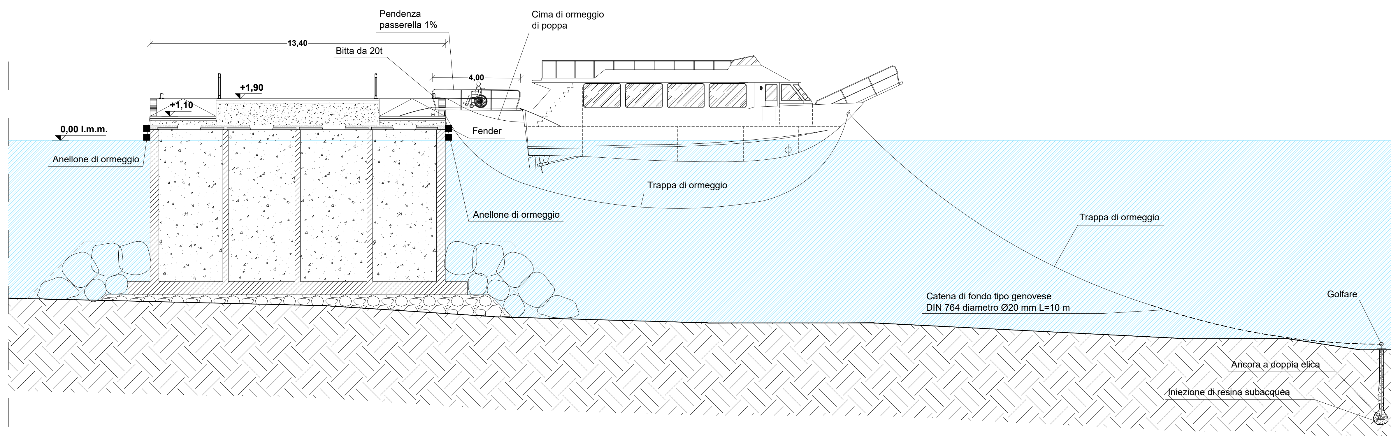
SEZIONE B2-B2 A LIVELLO MEDIO MARE (Scala 1:100)
