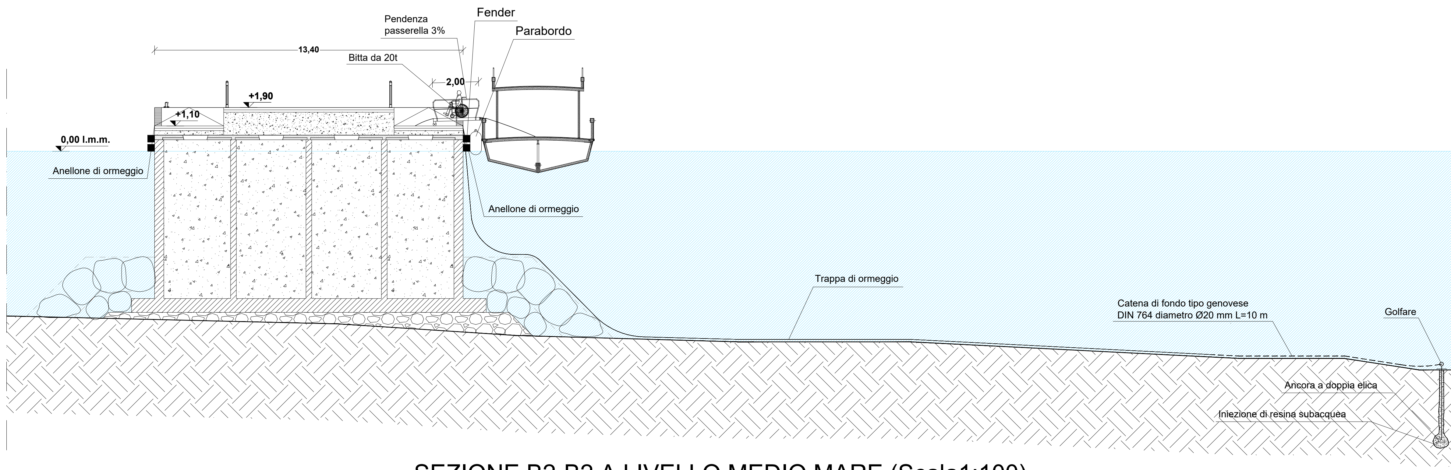
SEZIONE B2-B2 A LIVELLO MEDIO MARE (Scala1:100)
