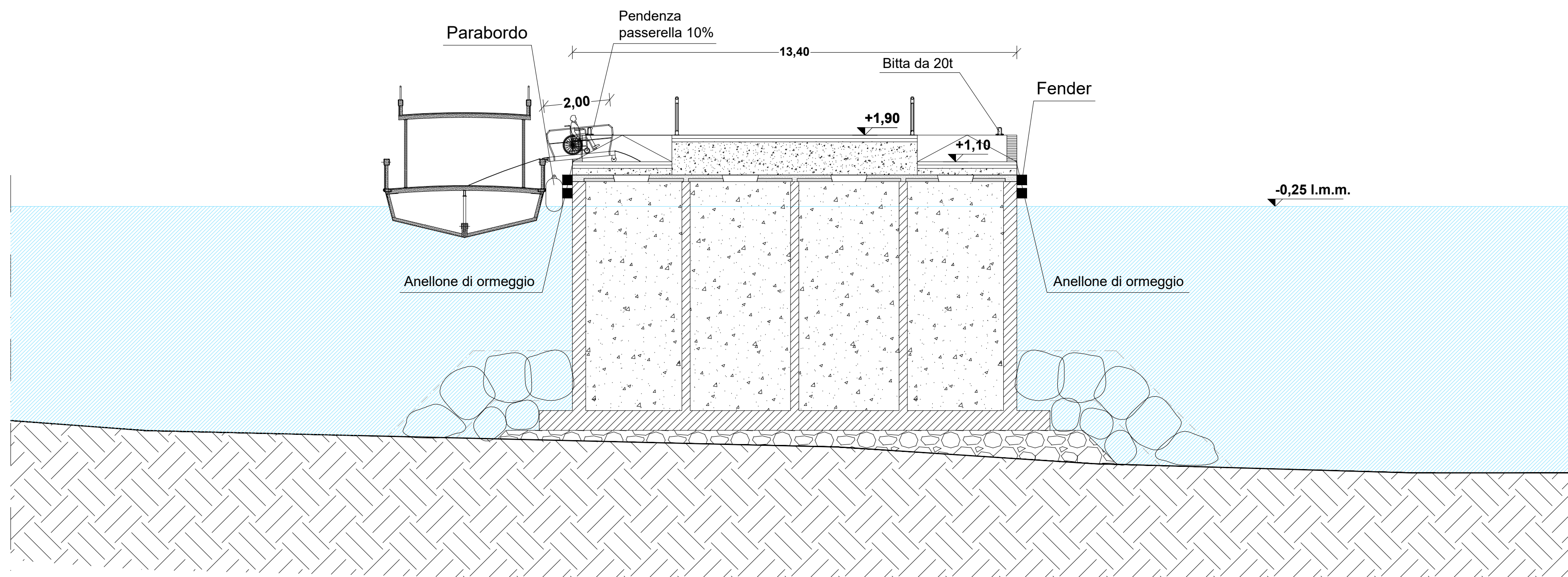
SEZIONE B2-B2 A LIVELLO MINIMO -0,25 m (Scala1:100)
