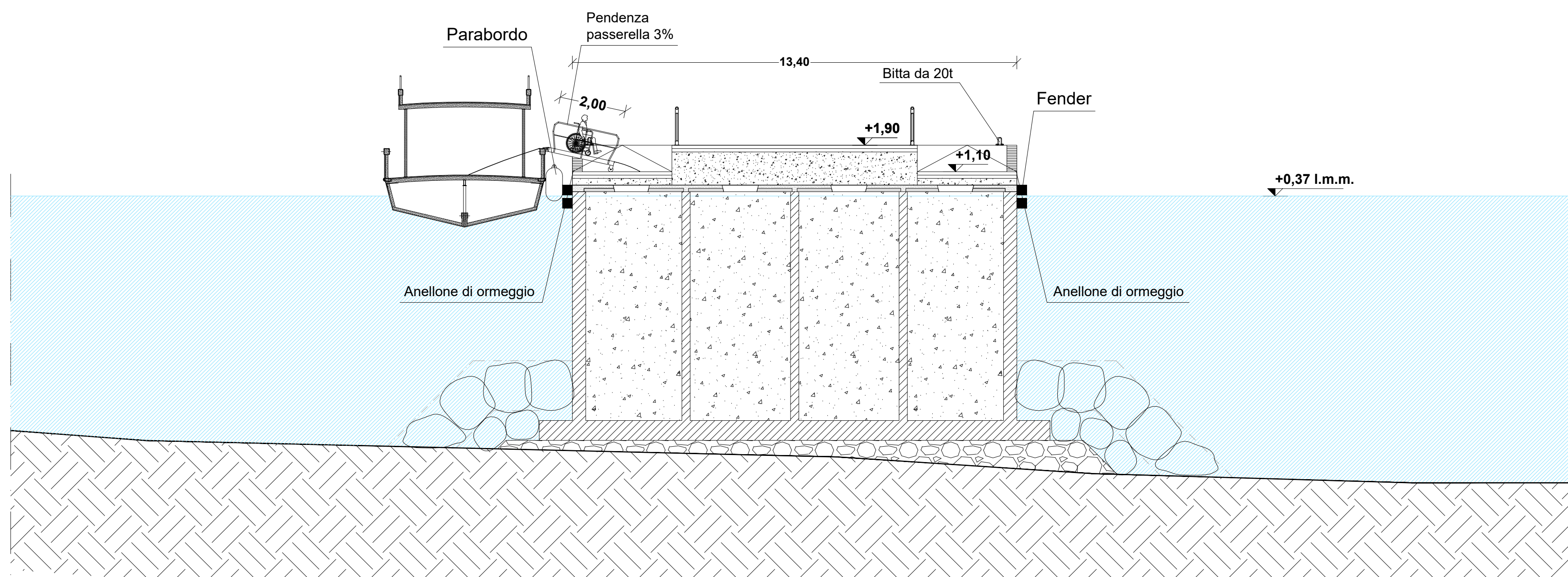
SEZIONE B2-B2 A LIVELLO MASSIMO +0,37 m (Scala1:100)
