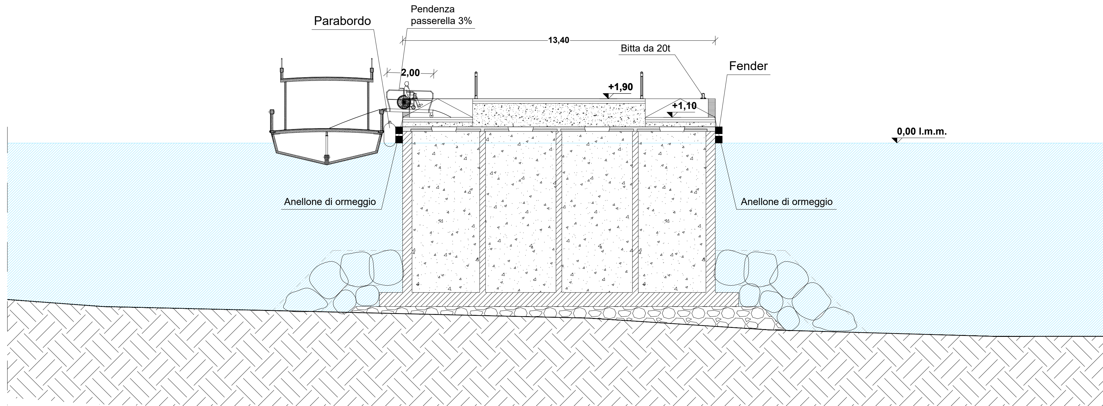
SEZIONE B2-B2 A LIVELLO MEDIO MARE (Scala1:100)
