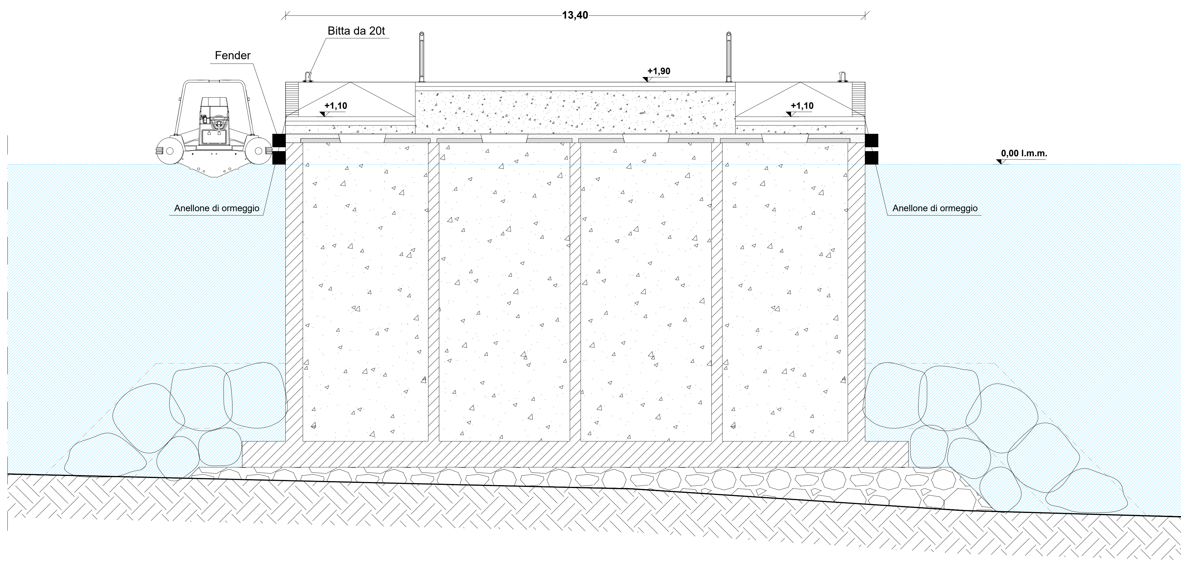
SEZIONE B2-B2 A LIVELLO MEDIO MARE (Scala1:50)
