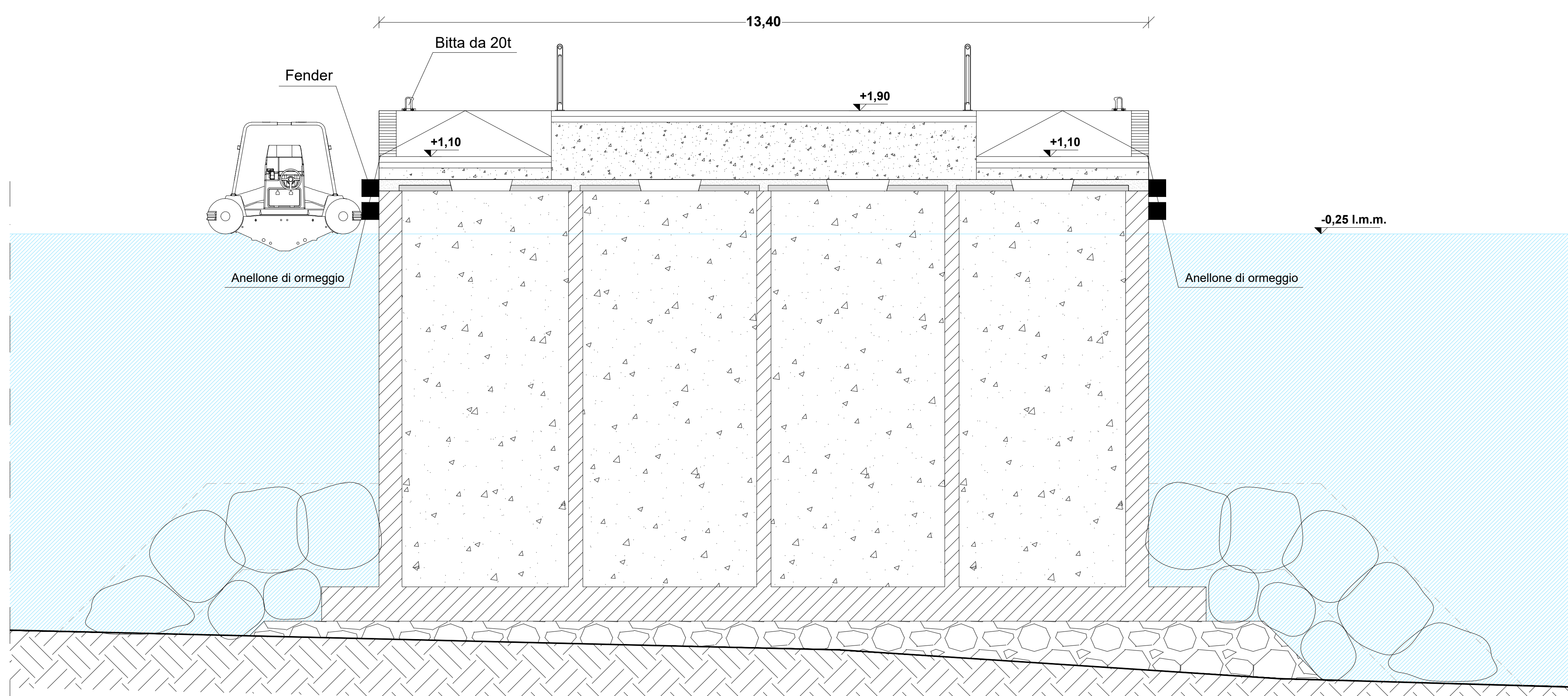
SEZIONE B2-B2 A LIVELLO MINIMO -0,25 m (Scala1:50)
