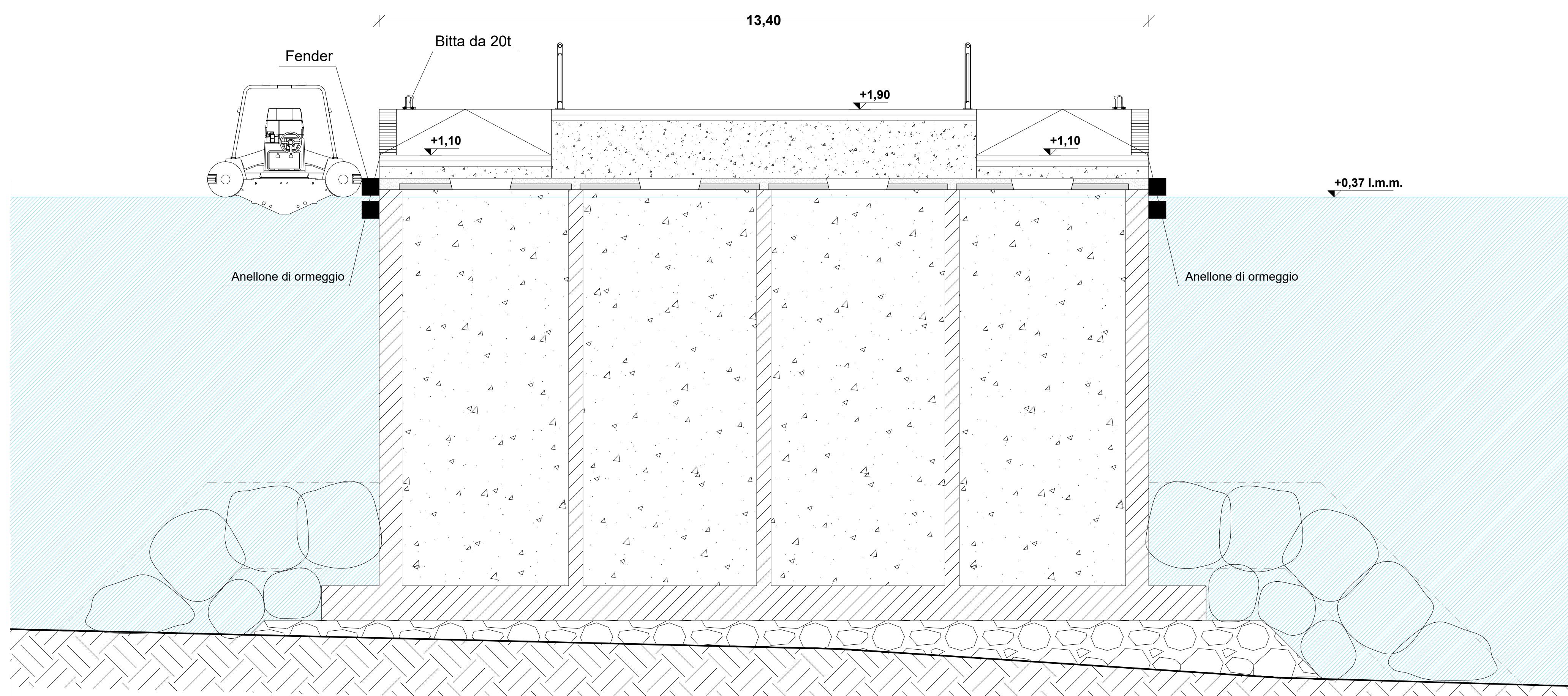
SEZIONE B2-B2 A LIVELLO MASSIMO +0,37 m (Scala1:50)
