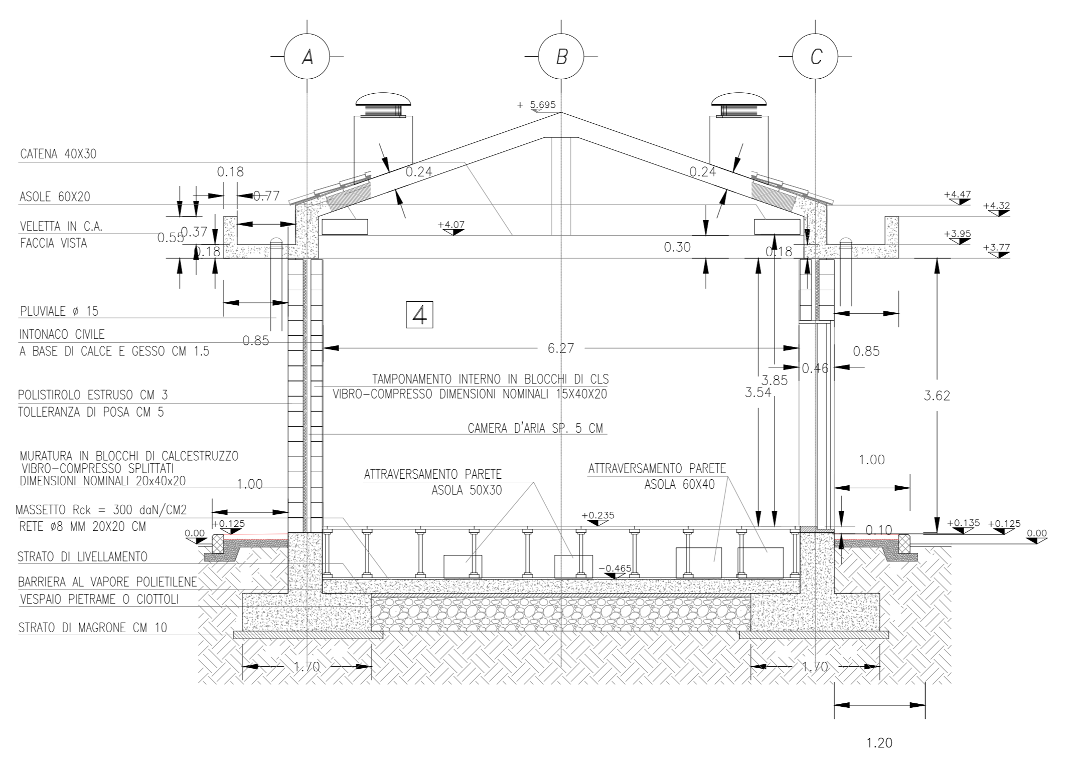
SEZIONE TRASVERSALE 3-3
