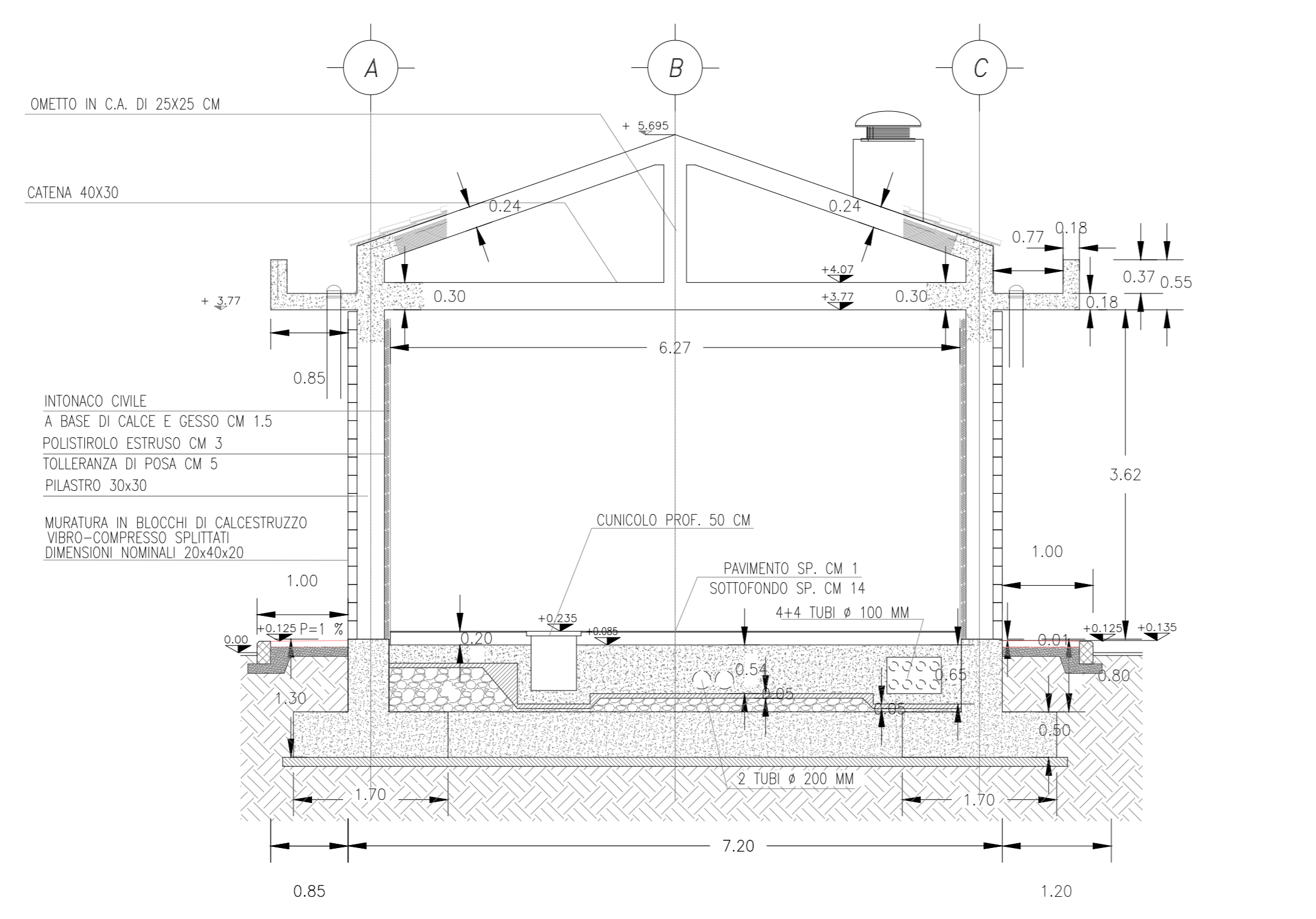
SEZIONE TRASVERSALE 2-2
