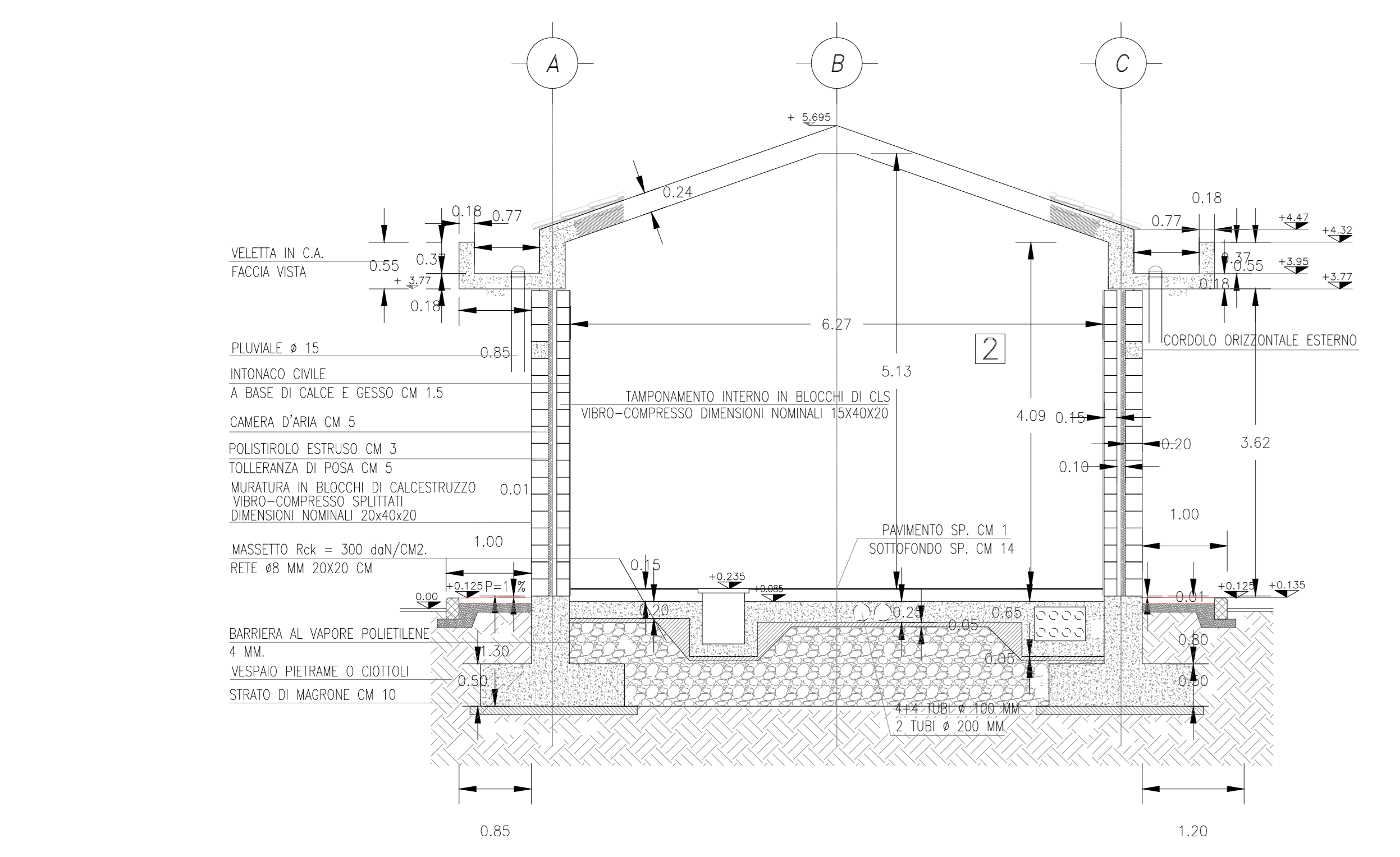
SEZIONE TRASVERSALE 1-1
