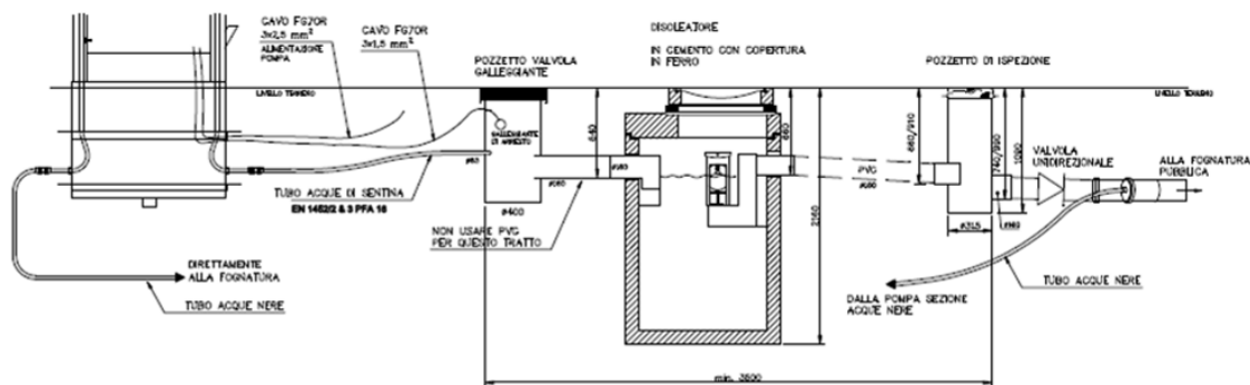
Figura 9 -Schema funzionale disoleatore
