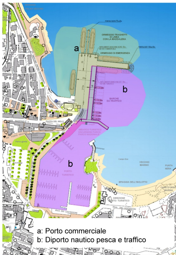
Figura 15 - schema di principio delle differenti aree funzionali dell'organismo portuale nell'assetto di progetto
