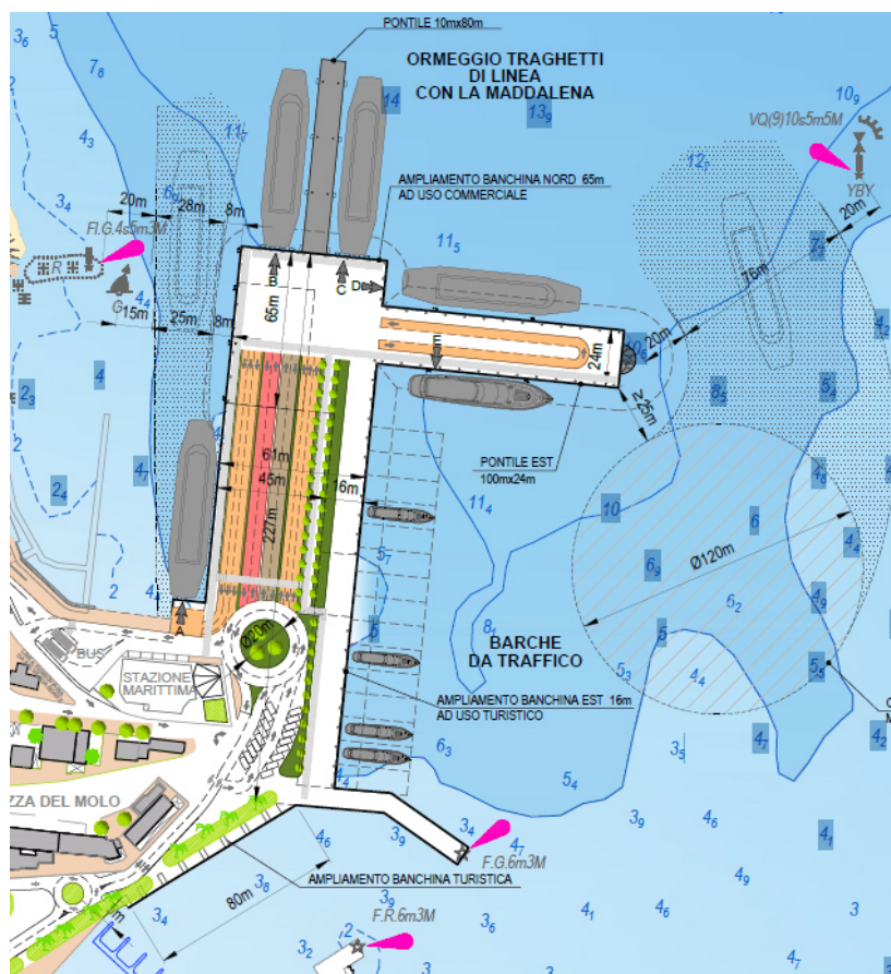
Figura 7 - Schema complessivo dell'impianto portuale
