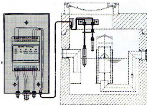
Esempio di installazione su Oleopator K
