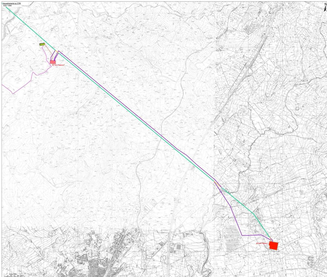
Figura 3-4: Inquadramento su CTR n.618060, 618070, 618110, cavidotto AT, SSE condivisione, SE "Partanna 3", elettrodotto aereo esistente e nuovo elettrodotto aereo 220 kV
