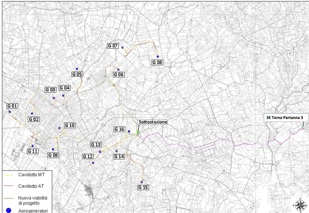
Figura 3-3: Inquadramento su CTR n.618040, 617010, 617080, 618050, impianto, sottostazione di trasformazione, cavidotto AT
