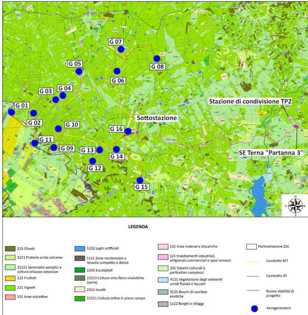
Figura 6-2: Carta dell'uso del suolo relativa all'impianto eolico (Fonte SITR Sicilia)
