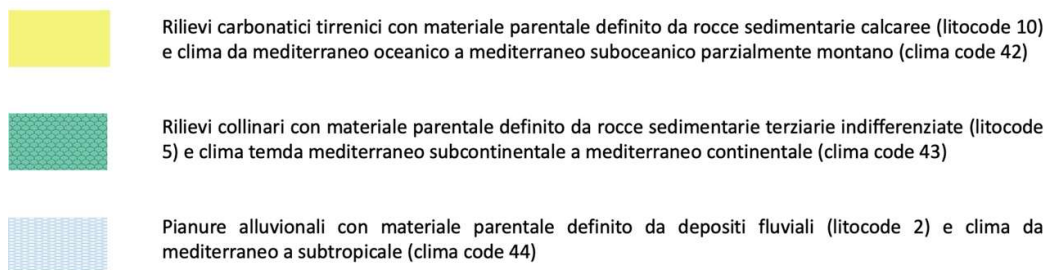
Figura 6-1: Carta ecopedologica dell'area in esame.
