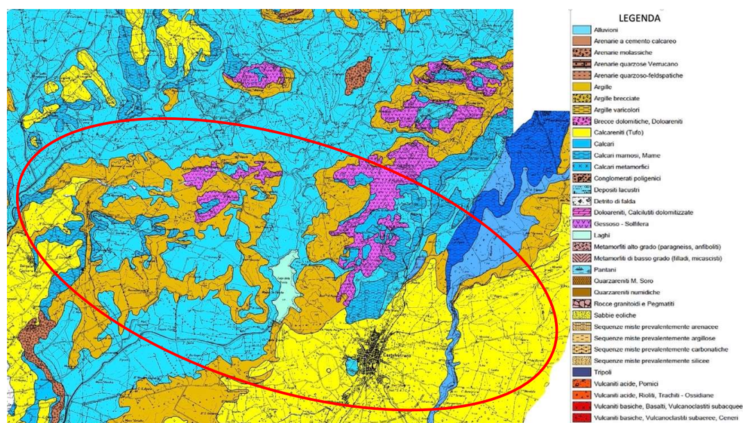
Figura 5-1: Carta litologica dell'area in esame
