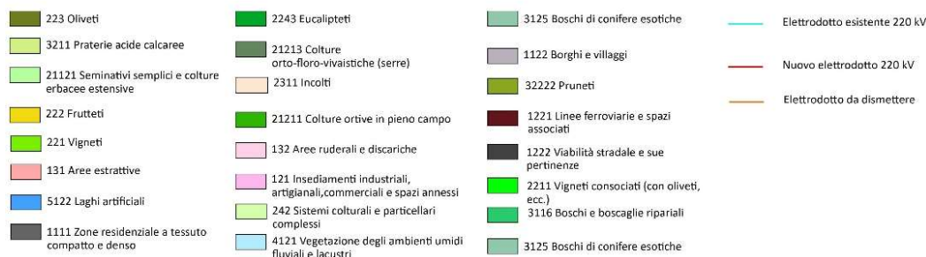
Figura 6-3: Carta dell'uso del suolo relativa alle opere di rete (Fonte SITR Sicilia).
