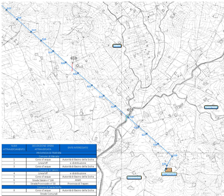
Figura 2-4: Inquadramento su CTR relativo al cavidotto AT, SSE di trasformazione condivisa, SE "Partanna 2" SE "Partanna 3", elettrodotto aereo esistente "Fulgatore Partanna" e nuovo elettrodotto aereo 220 kV
