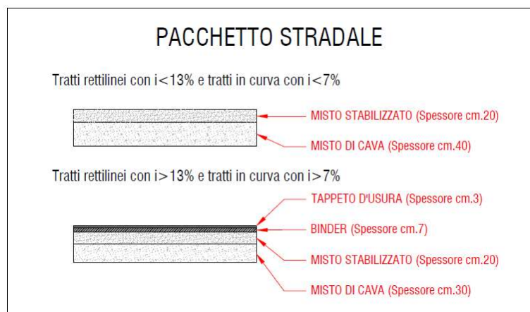
Figura 2-9: Pacchetti stradali
