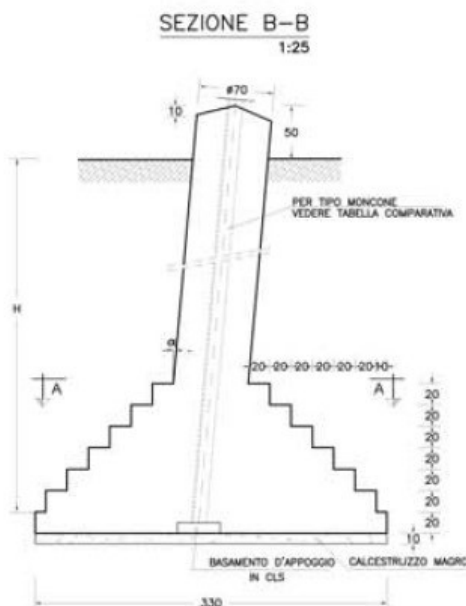
Figura 2-15: Schema tipo di fondazione per sostegni
