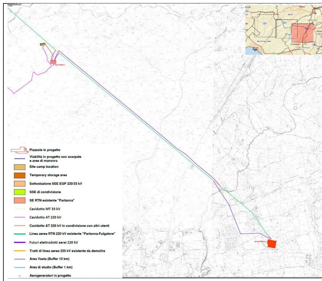
Figura 2-5: Carta di Inquadramento su CTR nuovo elettrodotto aereo 220 KV
