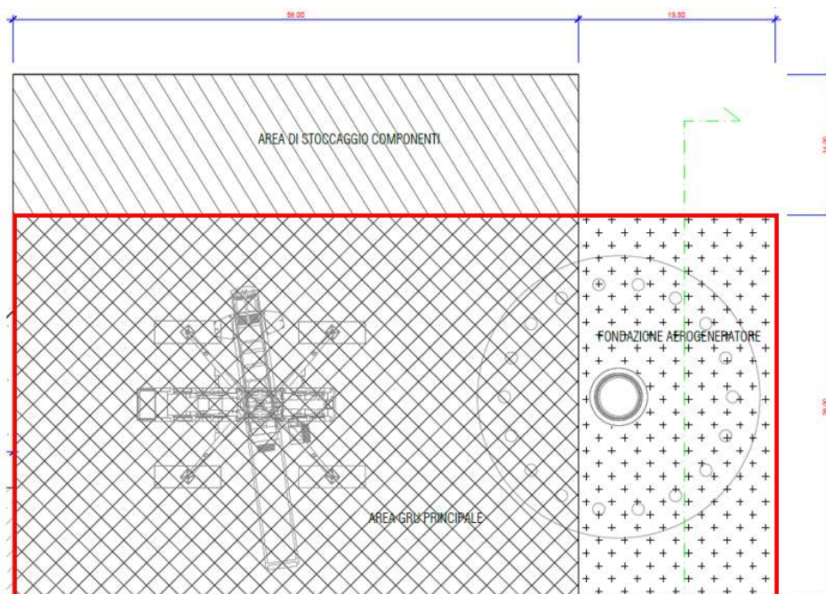
Figura 2-8: Piazzola – parte definitiva
