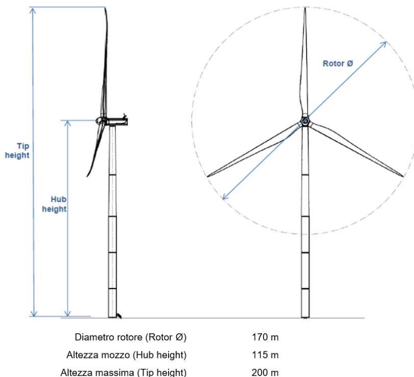
Figura 2-6: Vista e caratteristiche di un aerogeneratore da 4,2 MW
