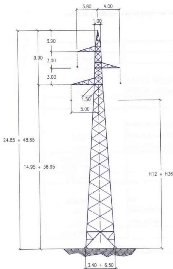
Figura 2-14: Sostegno tipo in semplice terna
