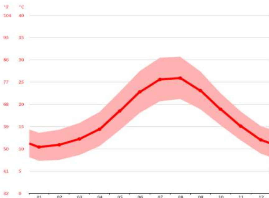
Grafico temperature medie annue
