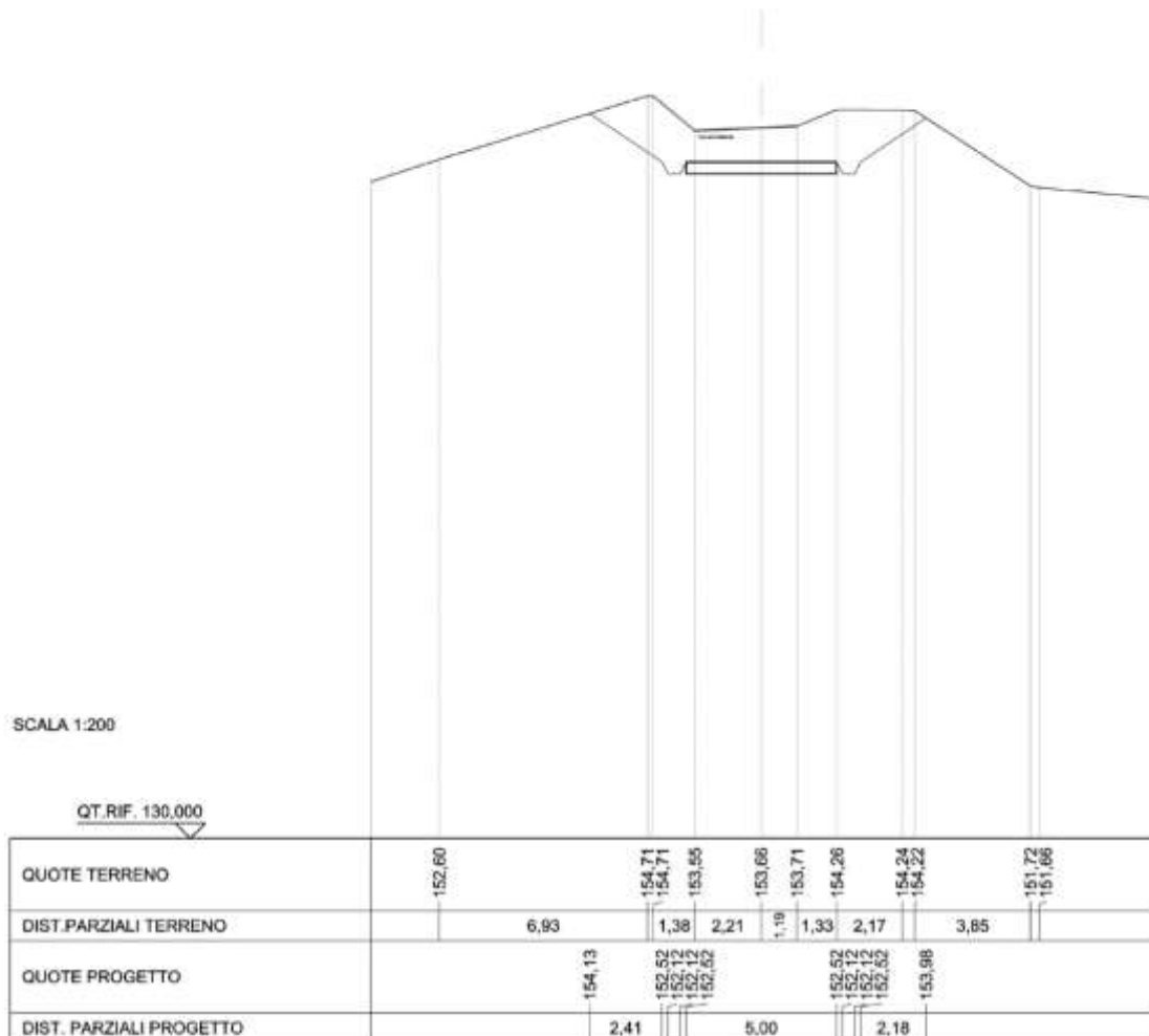
Fig. 10 - Sezioni stradali più significative
