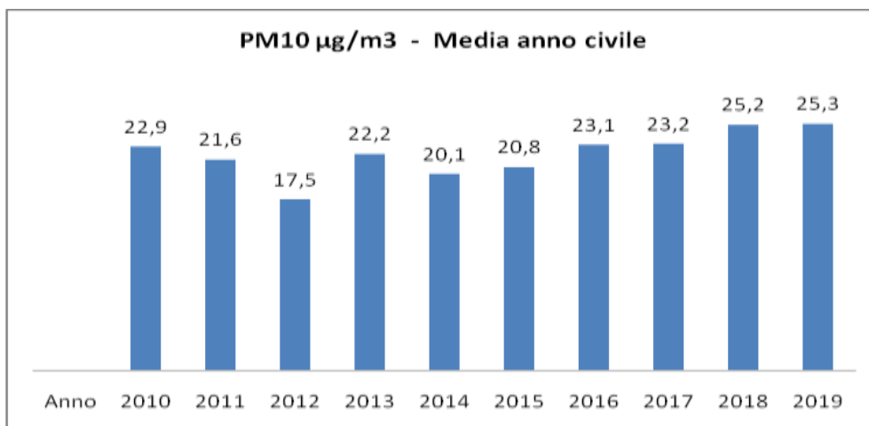
Andamento del PM 10 come media anno civile (40 µg/m 3 )” nel periodo 2010 – 2019
