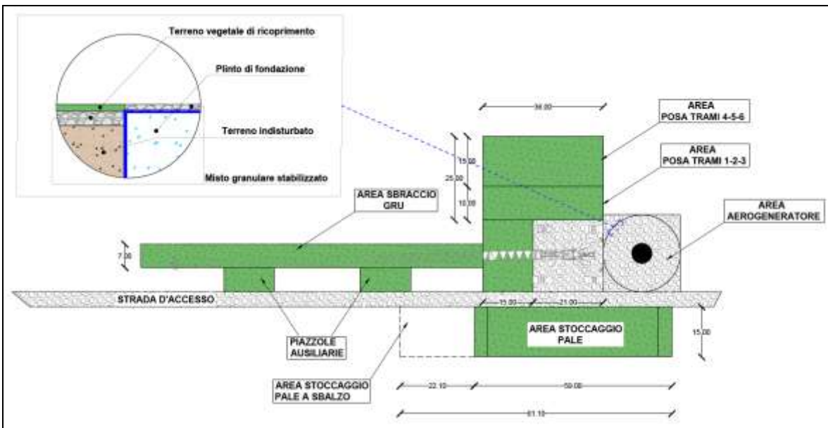
Planimetria piazzola tipo in fase di esercizio
