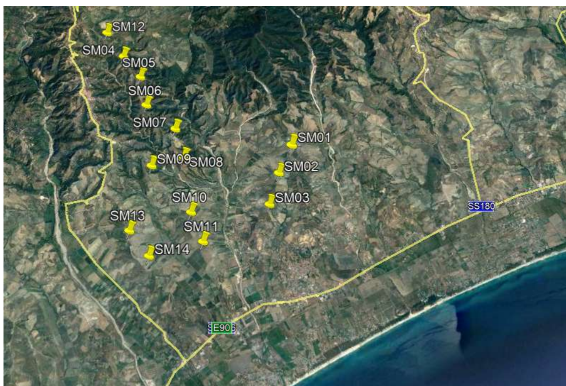
Fig 8 Vie di accesso Parco Eolico
