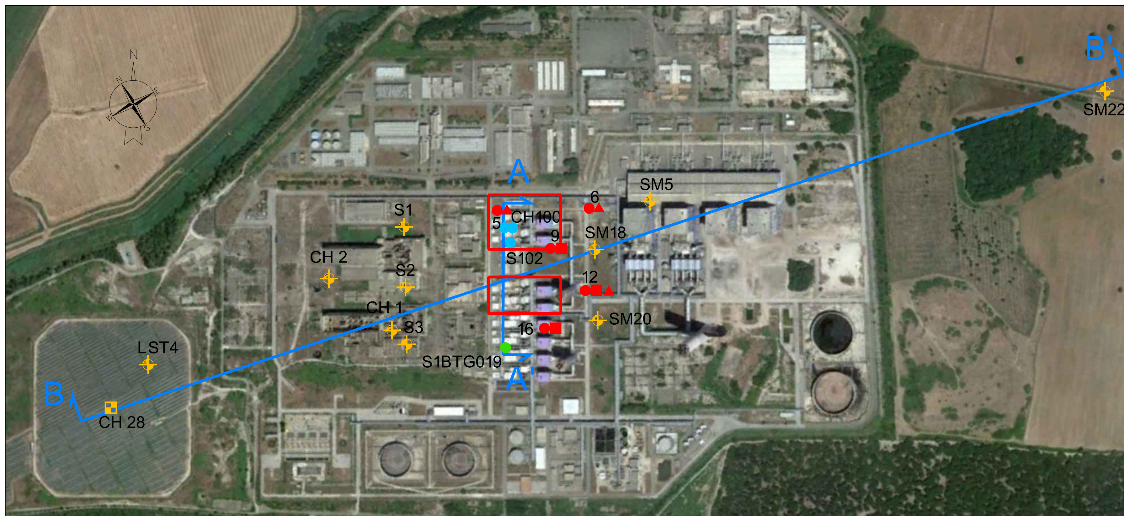
PLANIMETRIA GENERALE SCALA 1:2.500
