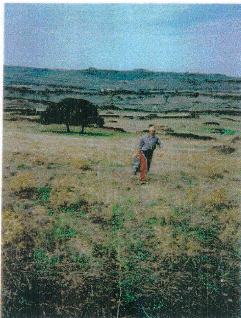
FOTO n° 7 - Panoramica Linea 3. Fase di acquisizione dati (spostamento del connoncino sismico sull'esterno della linea)
