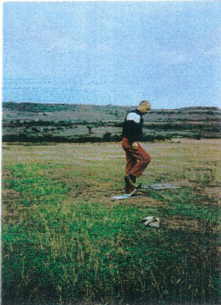
FOTO n° 8 - Particolare sull'esterno della linea 2 - Fase di energizzazione (visibile il cannonecino carico, inserito nel foro di energizzazione)
