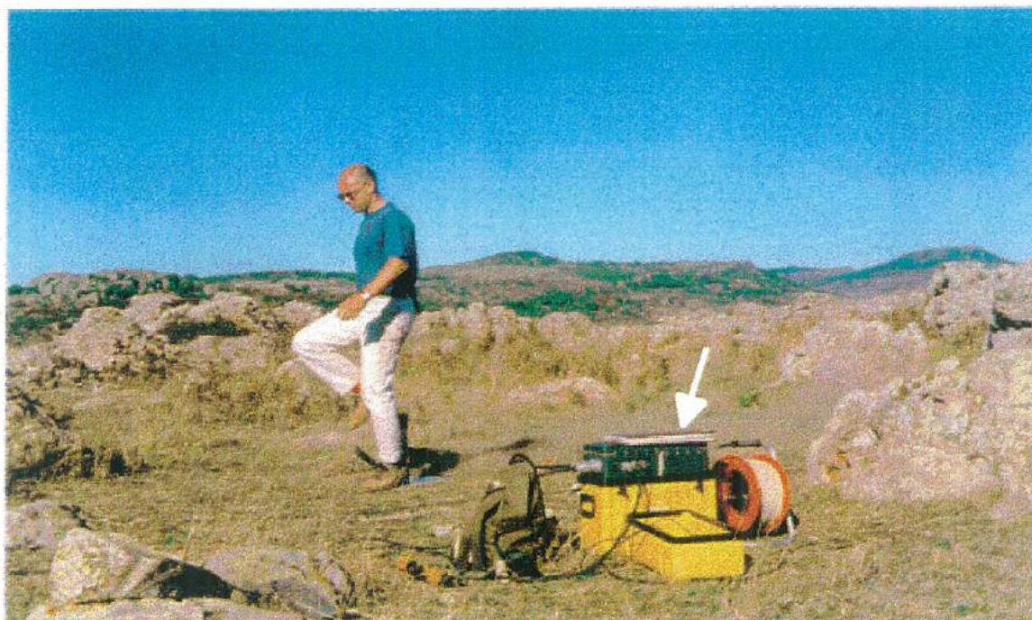
FOTO n° 11 - Linea a riflessione. Fase di energizzazione mediante cannoncino sismico (visibile il sismografo Smartseis a 24 canali)
