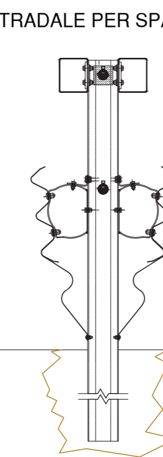
BARRIERA DI SICUREZZA STRADALE PER SPARTITRAFFICO MONOFILARE CLASSE H4
