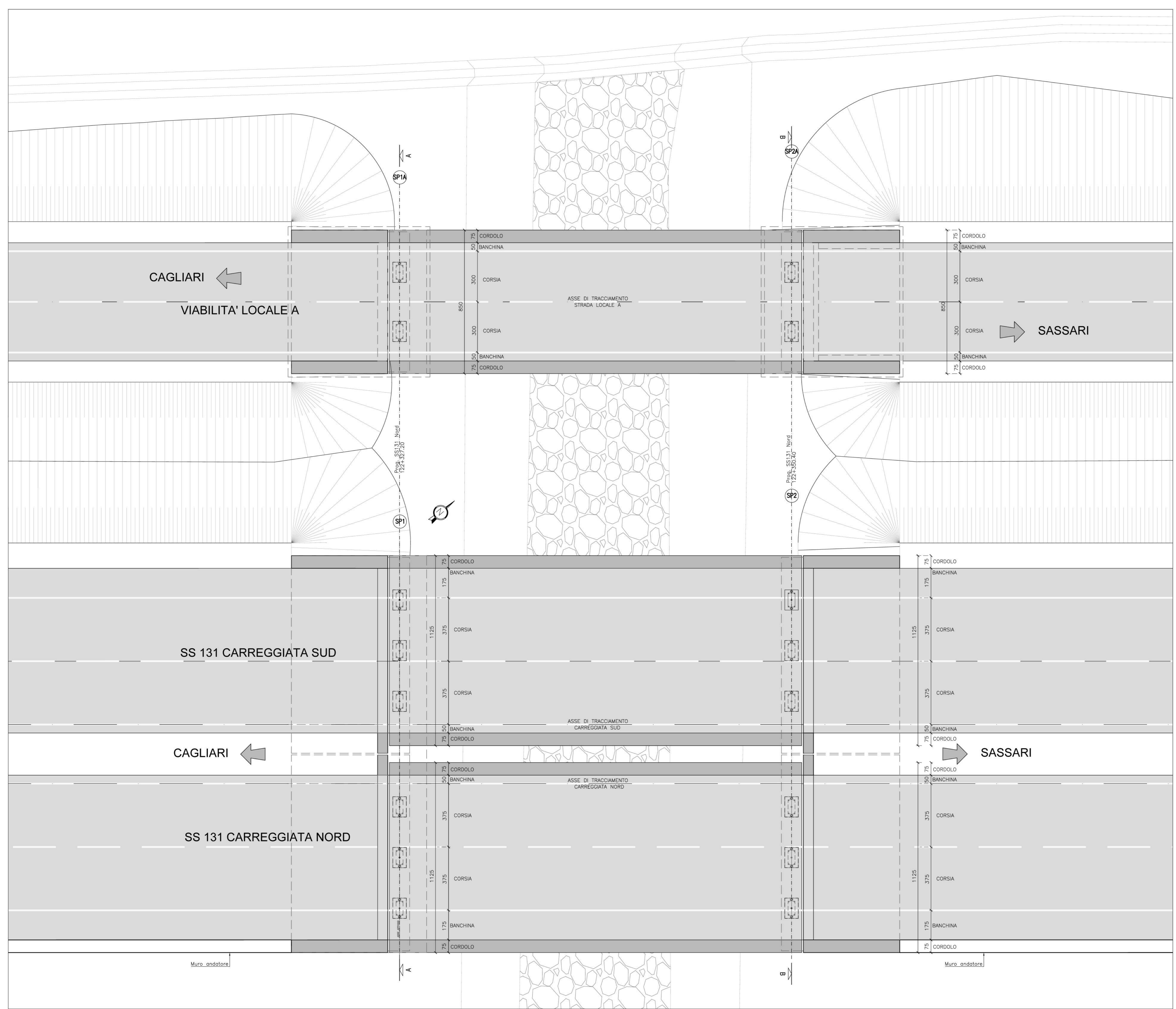
PIANTA Scala 1:100
