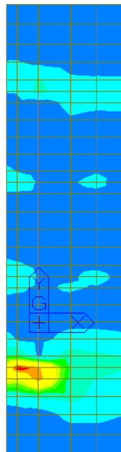
Figura 13-18: Tensioni nel cls dovute al momento flettente M_y (+)
