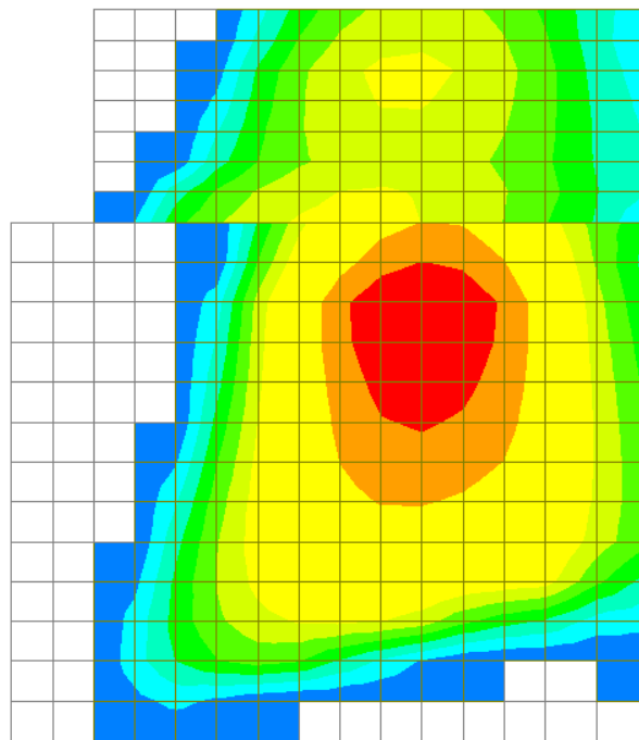
Figura 15-65: Apertura fessure dovuta al momento orizzontale (+)
