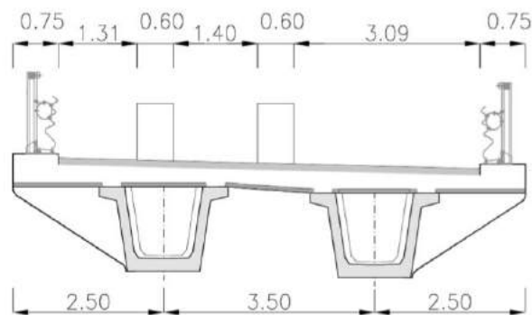
Figura 7-9 Disposizione carichi da traffico – Schema di carico 2 – caso 4
