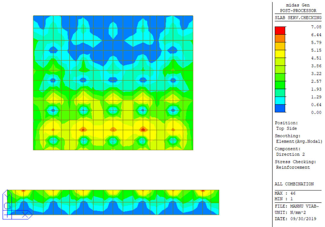
Figura 15-18: Tensioni nell'acciaio dovute al momento flettente M_y (-)
