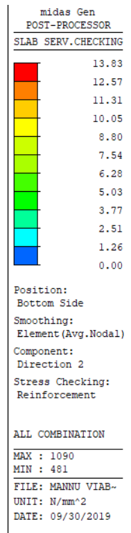
Figura 15-37: Tensioni nell'acciaio dovute al momento flettente orizzontale (+)
