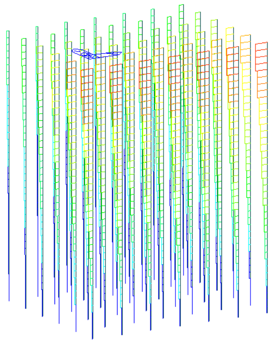
Figura 15-10: Massima sollecitazione sui micropali: combinazione ENV-SLU
