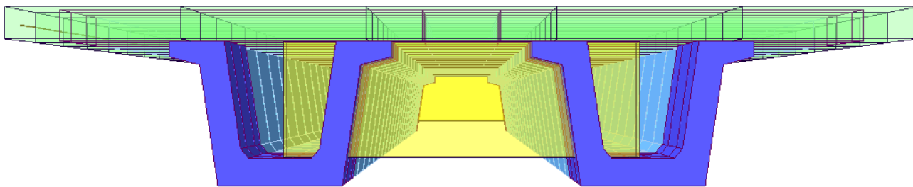
Figura 10-5 Modello FEM – Schematizzazione sezione trasversale tipo
