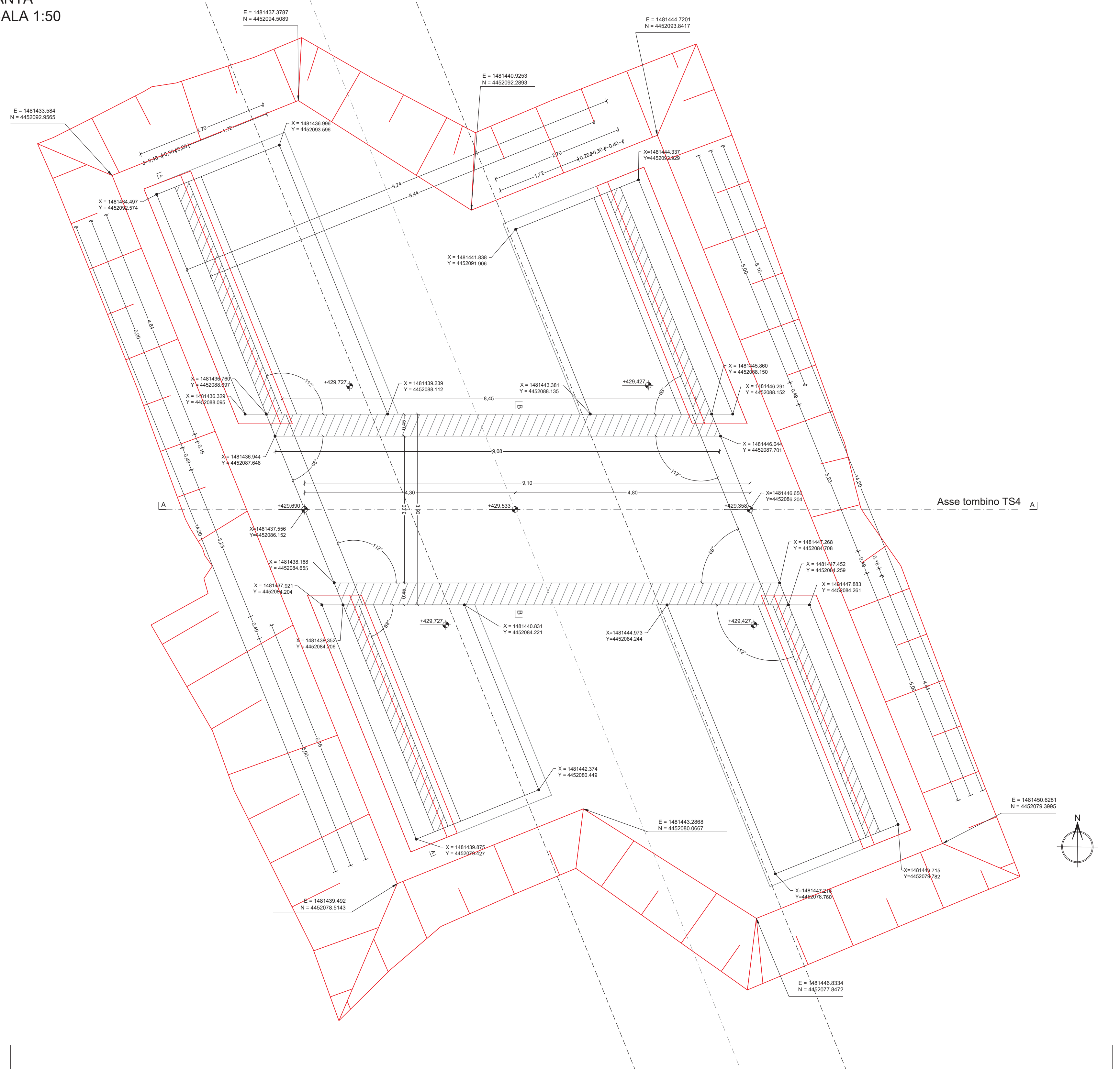
PIANTA SCALA 1:50
