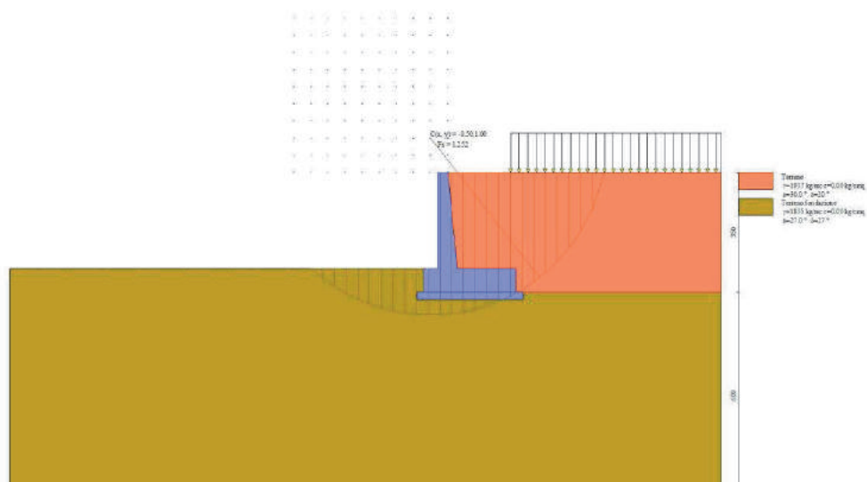
Figura 28 – Stabilità fronte di scavo - Cerchio critico (Combinazione n° 7)
