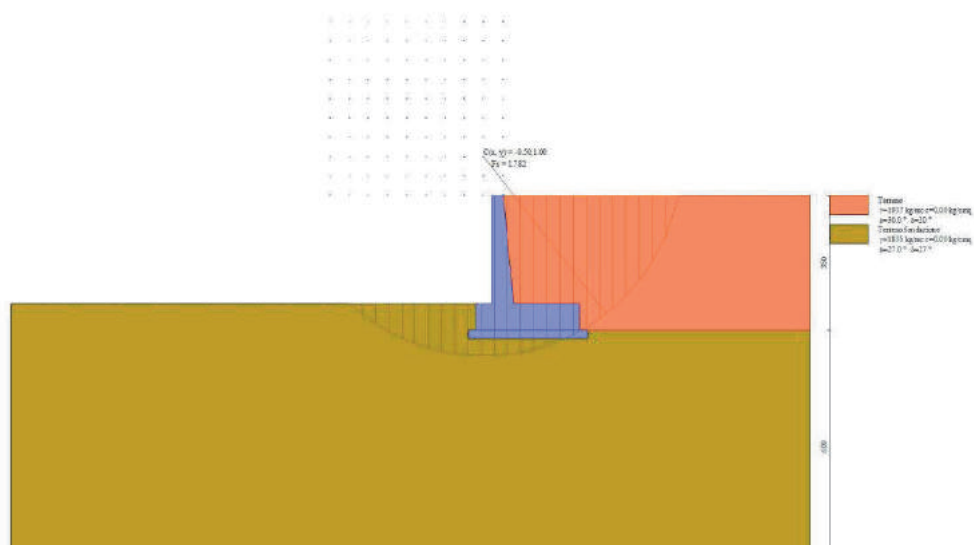
Figura 29 – Stabilità fronte di scavo - Cerchio critico (Combinazione n° 8)
