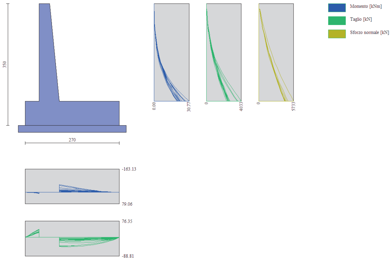
Figura 31 – Inviluppo delle sollecitazioni
