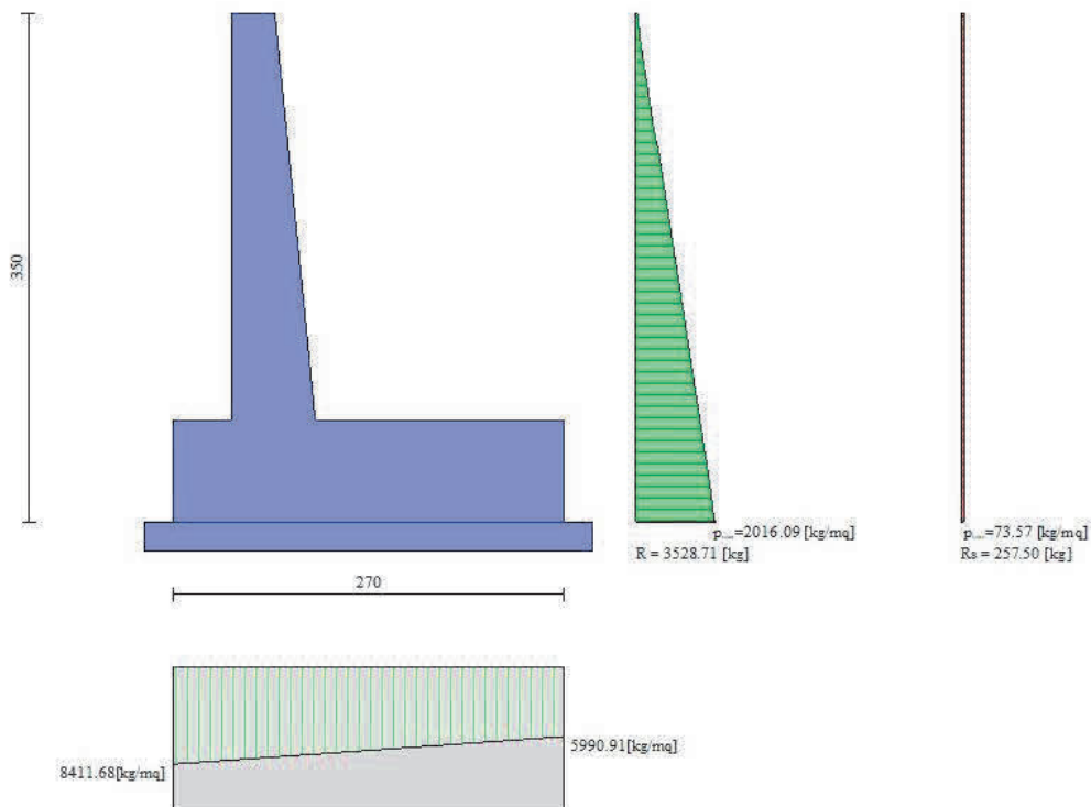
Figura 27 – Diagramma delle pressioni agenti sull'opera (combinazione sismica) (Combinazione n° 2)
