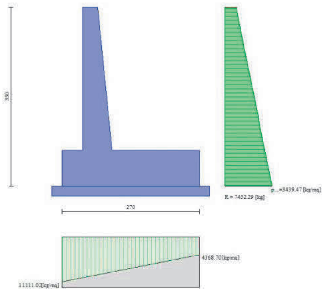
Figura 26 – Diagramma delle pressioni agenti sull'opera (combinazione statica) (Combinazione n° 1)
