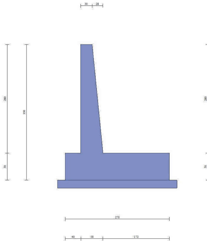
Figura 20 – Geometria del muro d'ala
