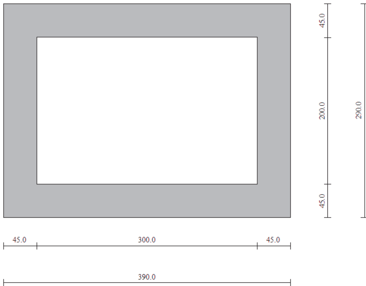
Figura 1 – Sezione trasversale del tombino
