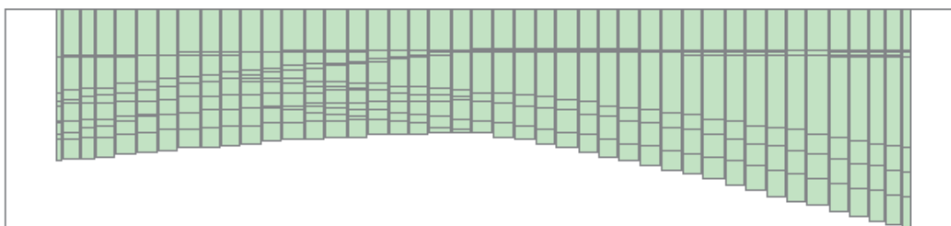
Figura 18 – Involuppo delle pressioni sul terreno di fondazione
