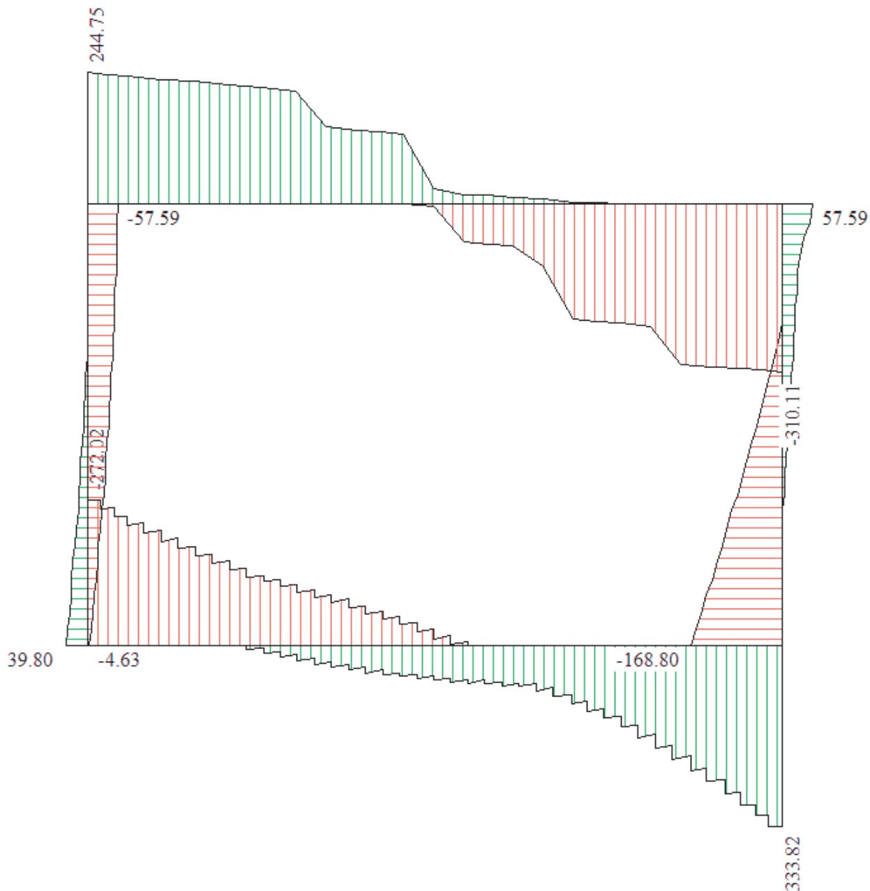
Figura 16 – Involuppo del diagramma del taglio
