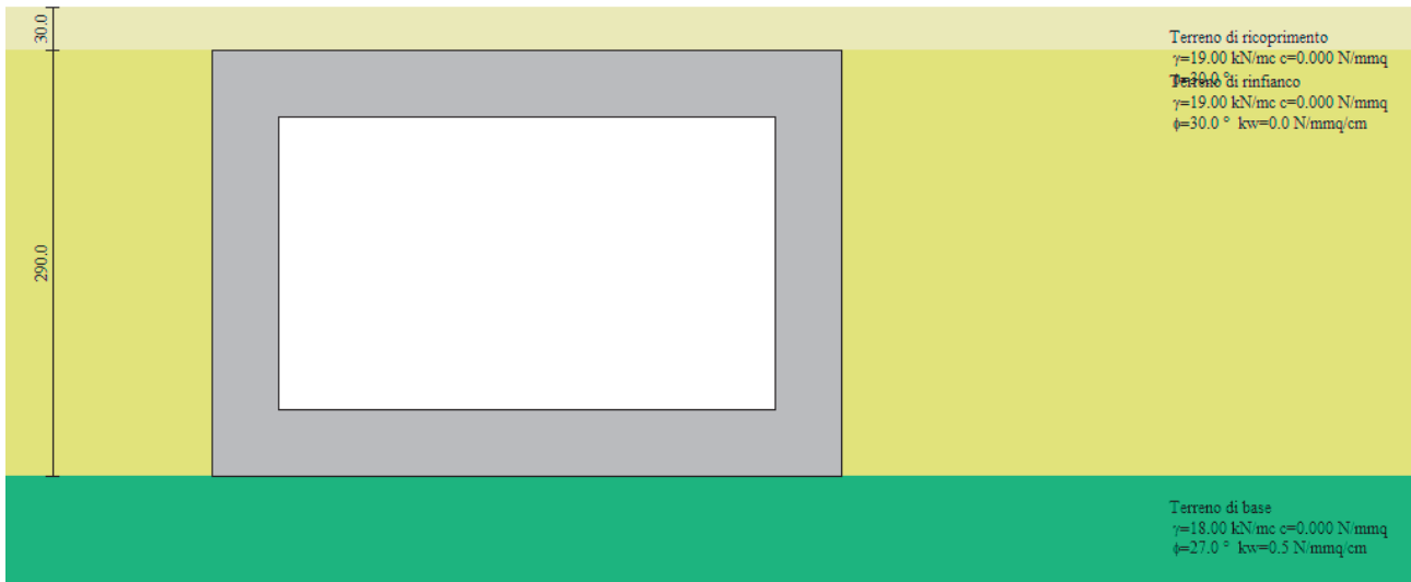
Figura 2 – Stratigrafia e caratteristiche del terreno
