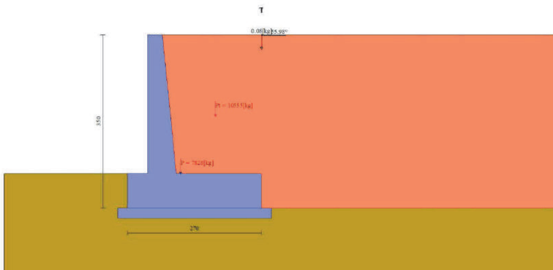
Figura 24 – Cuneo di spinta statico (Combinazione n° 1)
