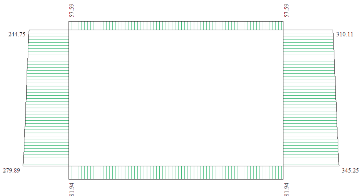
Figura 17 – Involuppo del diagramma dello sforzo normale
