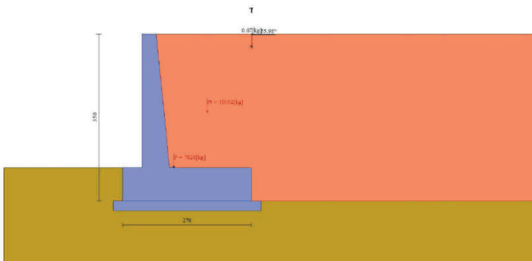
Figura 25 – Cuneo di spinta sismico (Combinazione n° 2)
