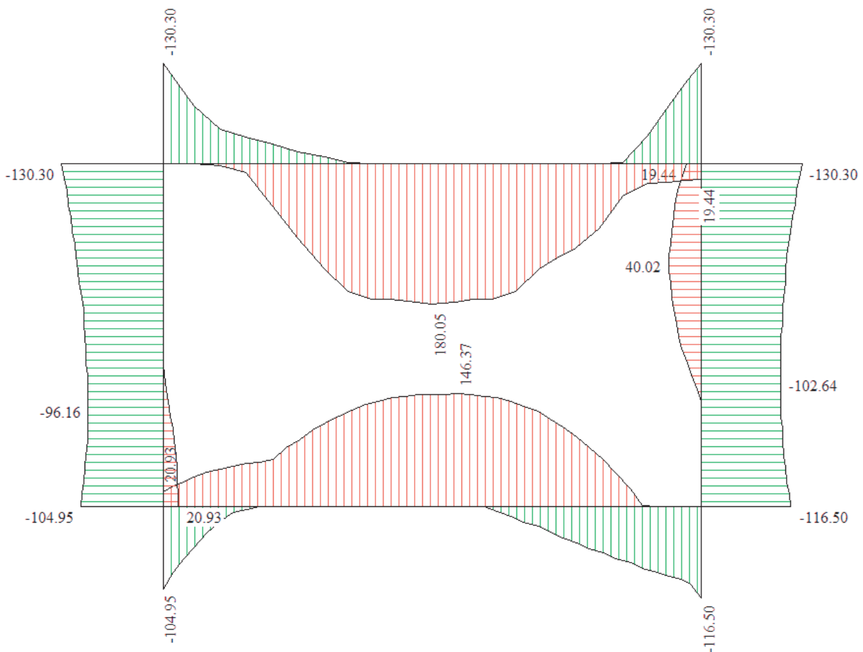
Figura 15 – Involuppo del diagramma del momento
