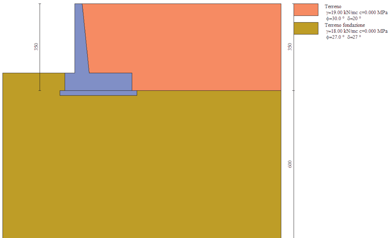
Figura 21 – Profilo del terreno
