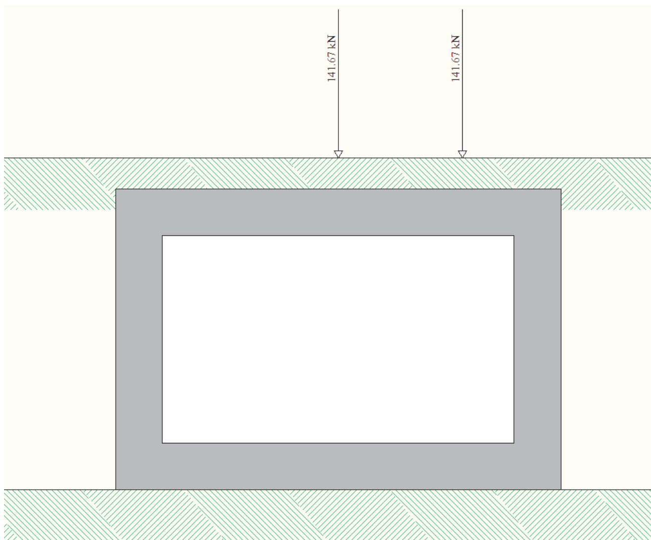
Figura 11 – Gruppo 2 – carico tandem (condizione di carico n°9)
