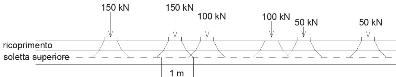
Figura 7 – Diffusione trasversale dei carichi tandem
