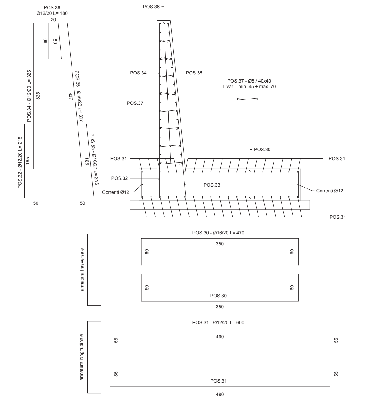
SEZIONE TRASVERSALE MURI SCALA 1:50
