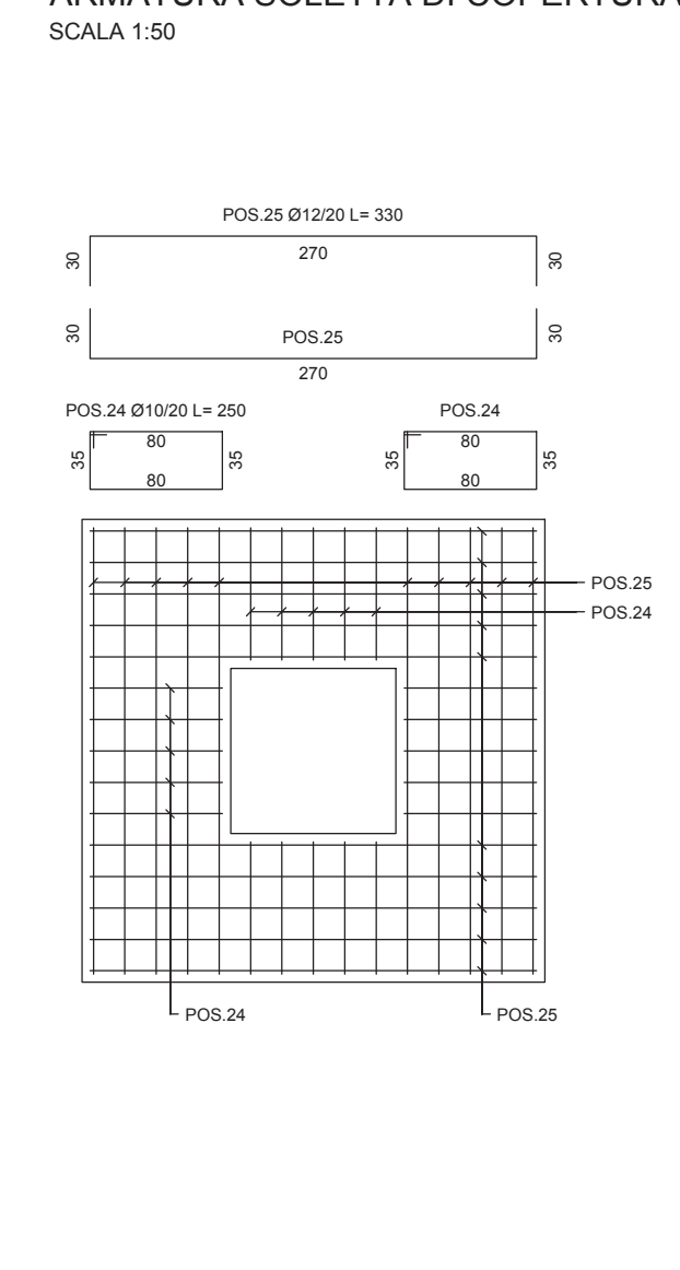
ARMATURA SOLETTA DI COPERTURA SCALA 1:50
