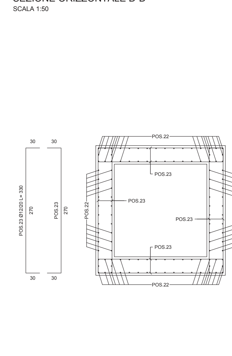
SEZIONE ORIZZONTALE D-D SCALA 1:50
