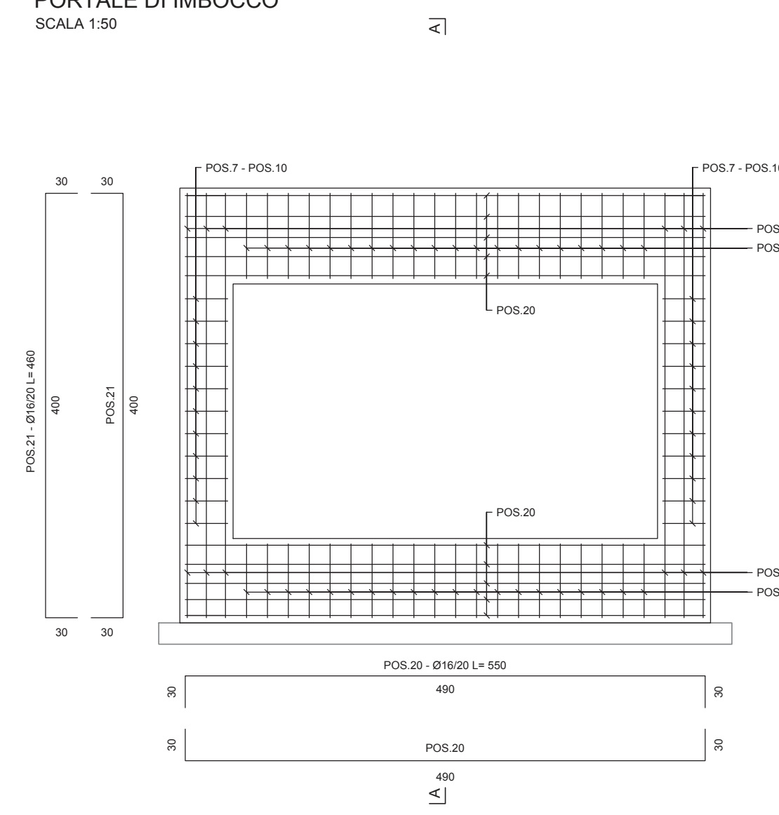
PORTALE DI IMBOCCO SCALA 1:50
