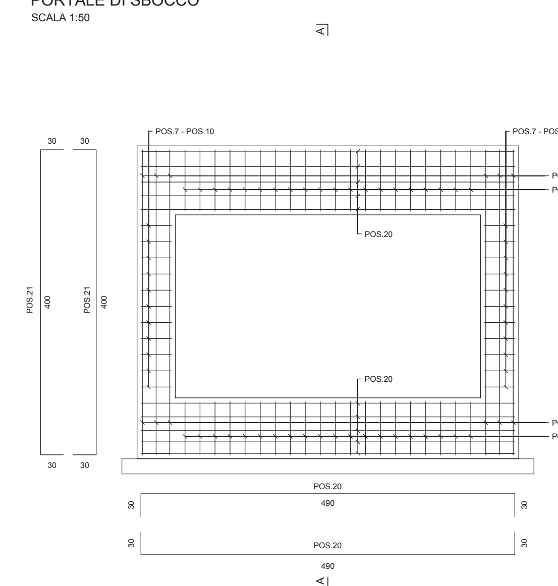
PORTALE DI SBocco SCALA 1:50
