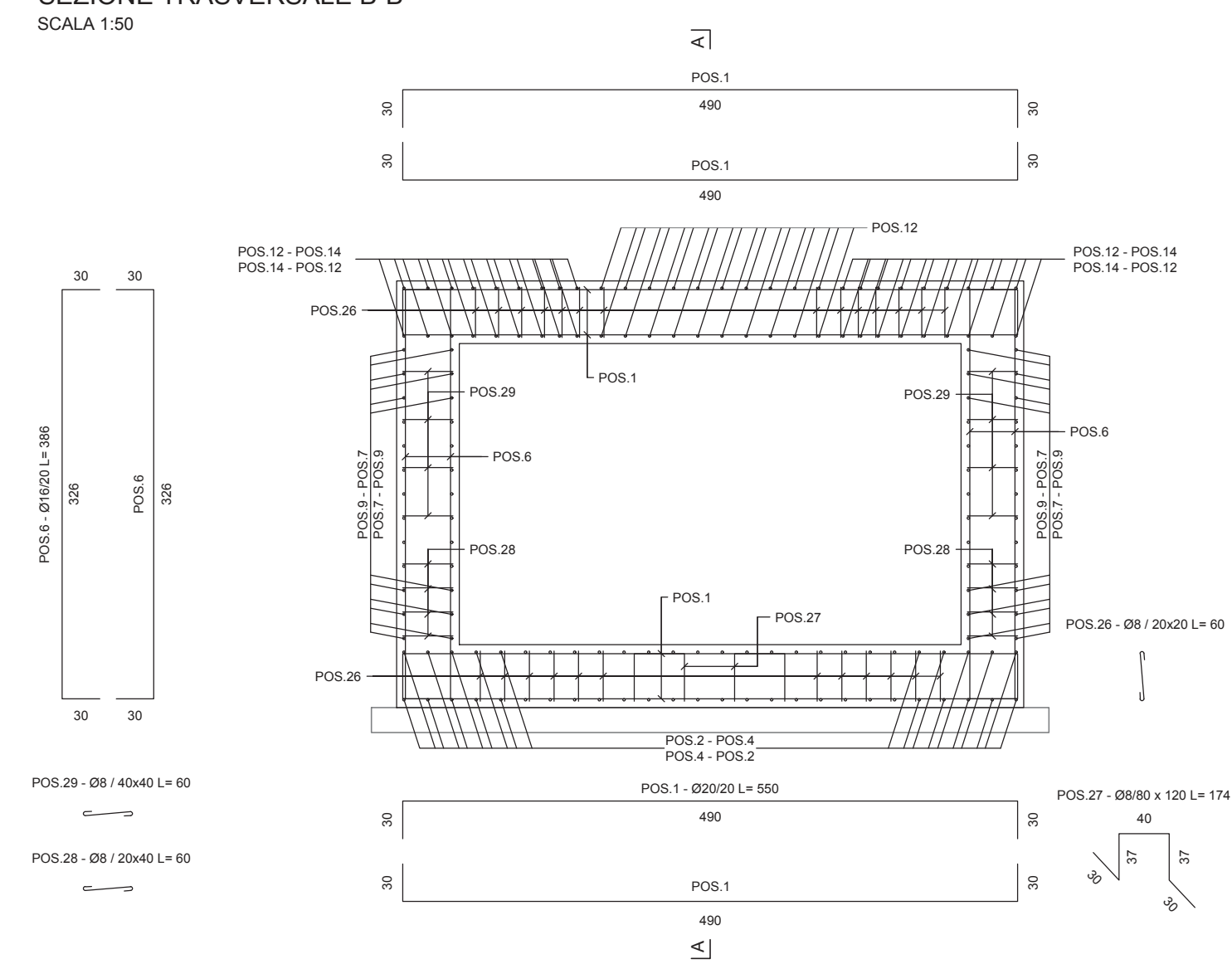
SEZIONE TRASVERSALE B-B SCALA 1:50
