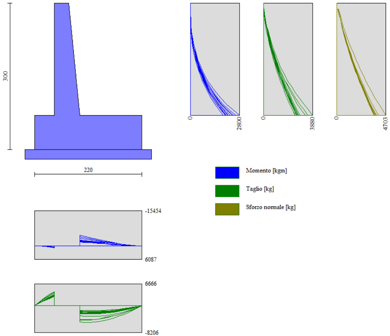
Figura 29 – Inviluppo delle sollecitazioni
