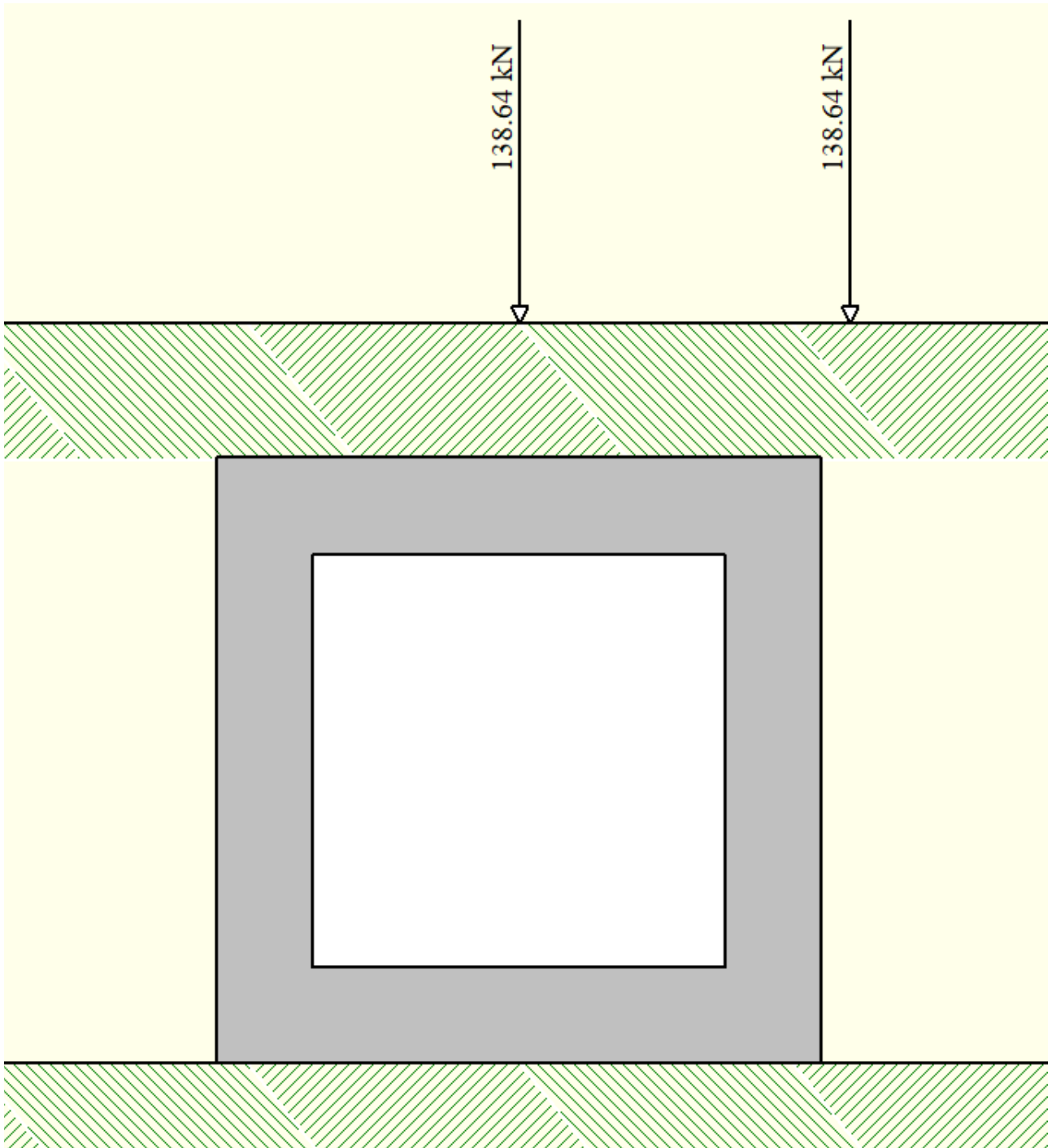
Figura 11 – Gruppo 2 – carico tandem (condizione di carico n°9)
