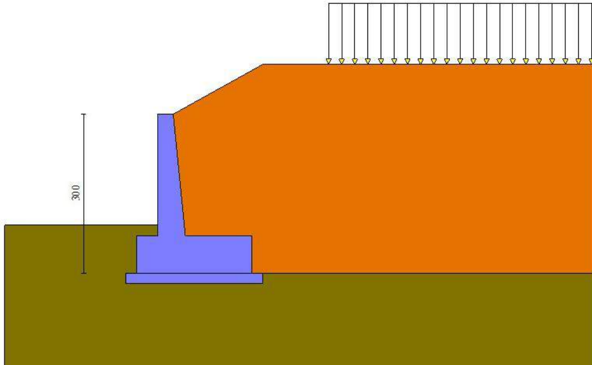
Figura 22 – Carico variabile
