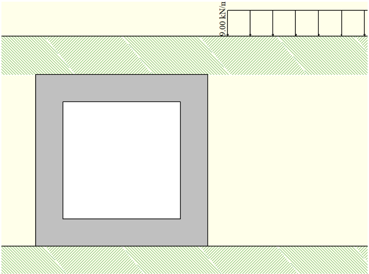
Figura 12 – Gruppo 3 – carico distribuito (condizione di carico n°13)
