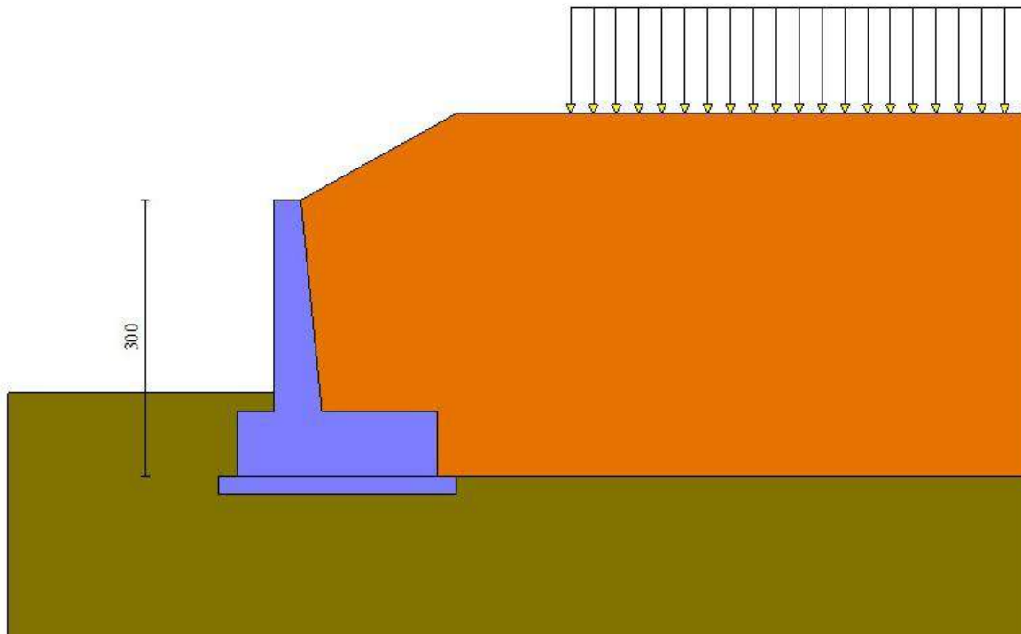
Figura 22 – Carico variabile
