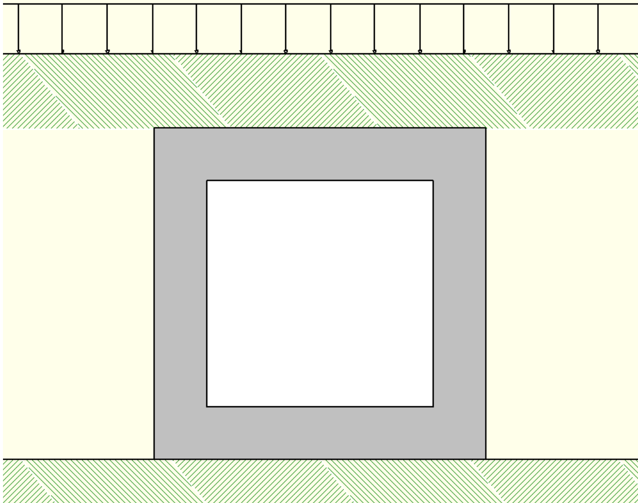
Figura 8 – Gruppo 1 – carico distribuito (condizione di carico n°7)
