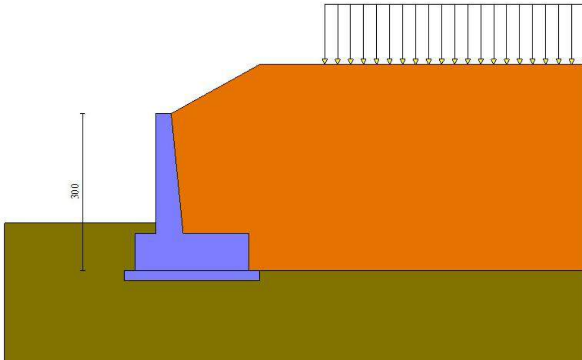
Figura 22 – Carico variabile
