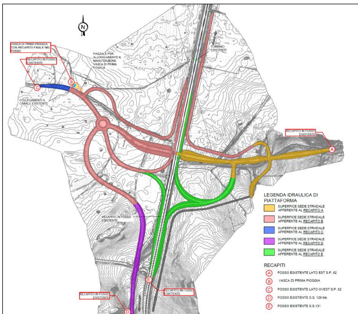
Figura 23 – Alternativa 2 – Individuazione recapiti acque di piattaforma e relative superfici afferenti
