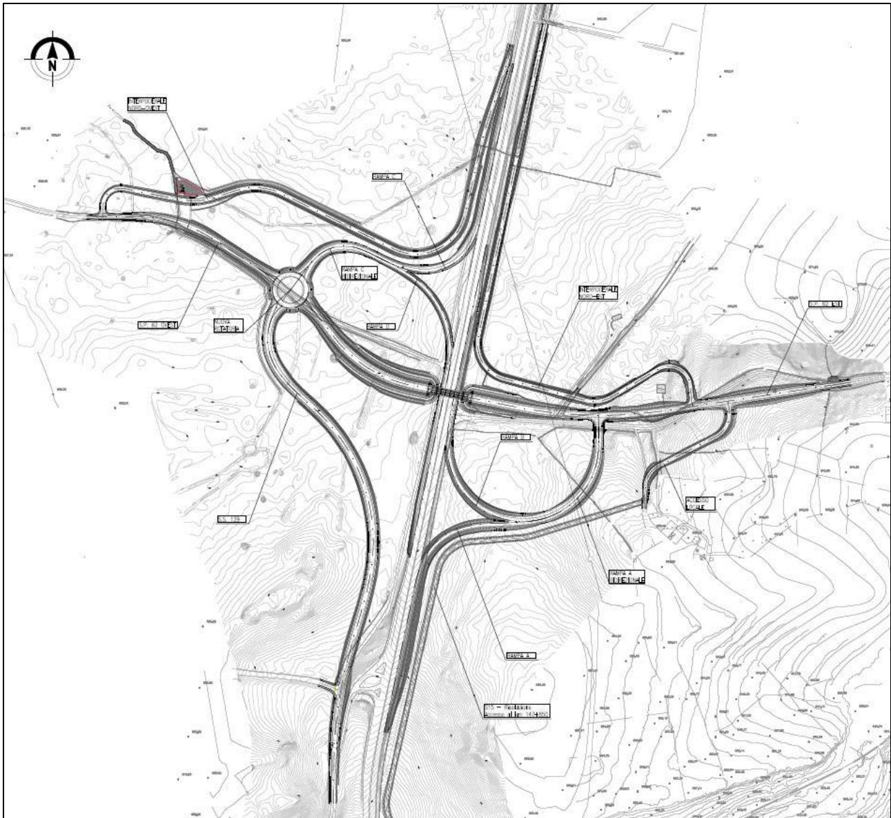
Figura 3 – Svincolo di Mulargia-Macomer Soluzione da Progetto Definitivo
