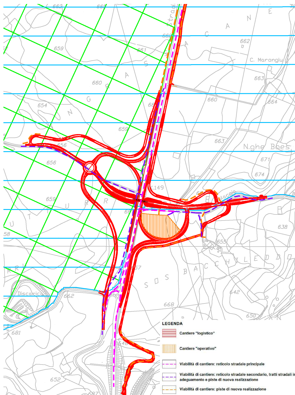
Figura 15 – Soluzione P.D. – Aree di cantiere e viabilità di servizio
