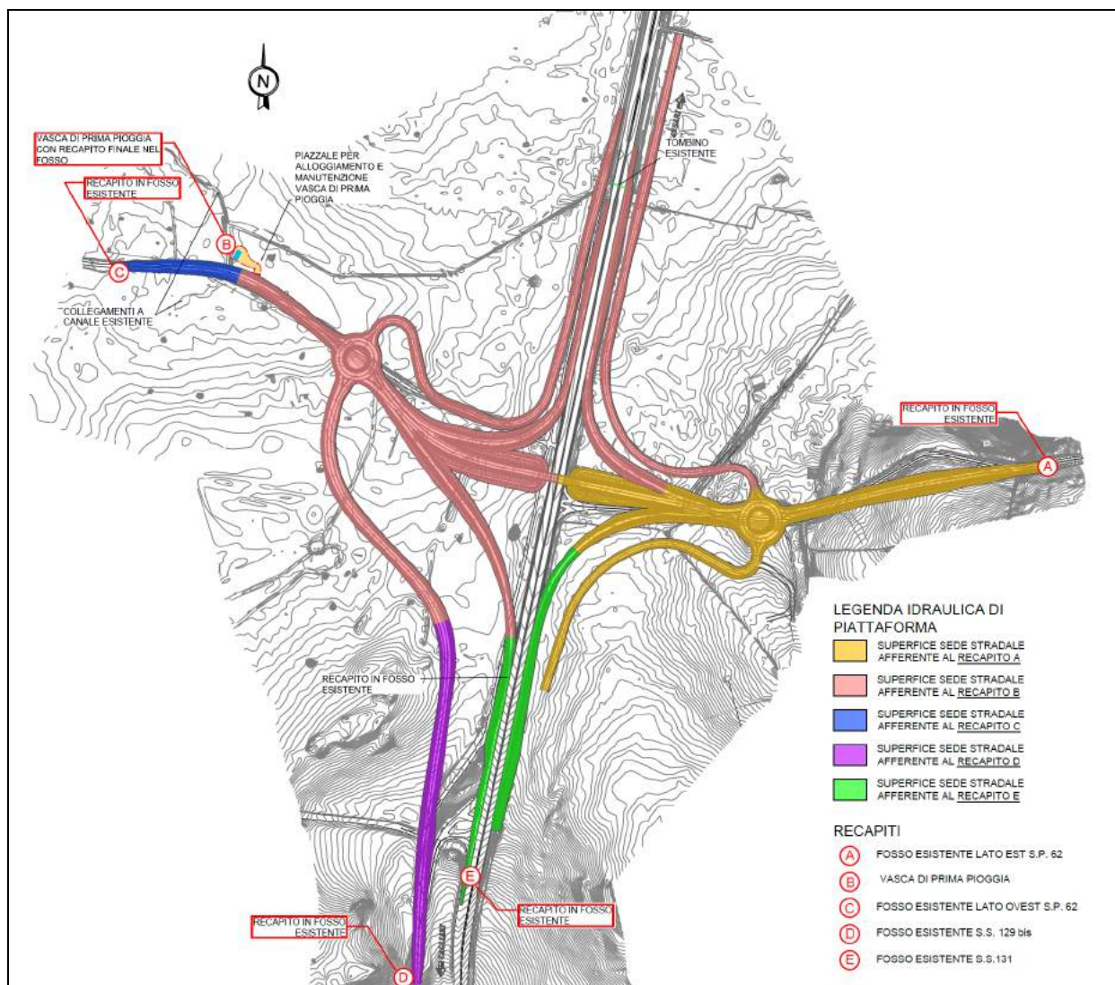
Figura 22 – Alternativa 1 – Individuazione recapiti acque di piattaforma e relative superfici afferenti
