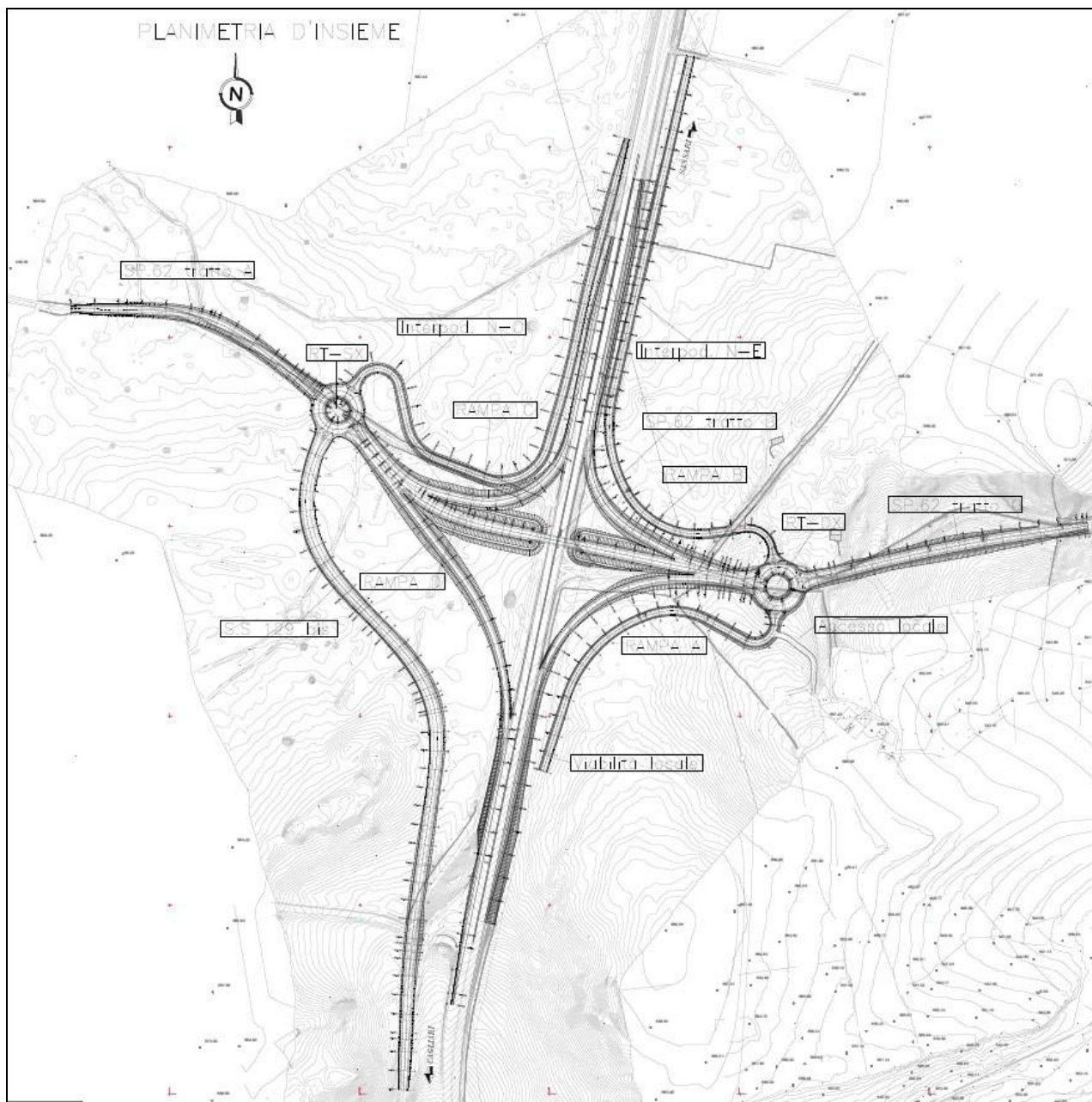
Figura 4 – Svincolo di Mulargia-Macomer Alternativa 1
