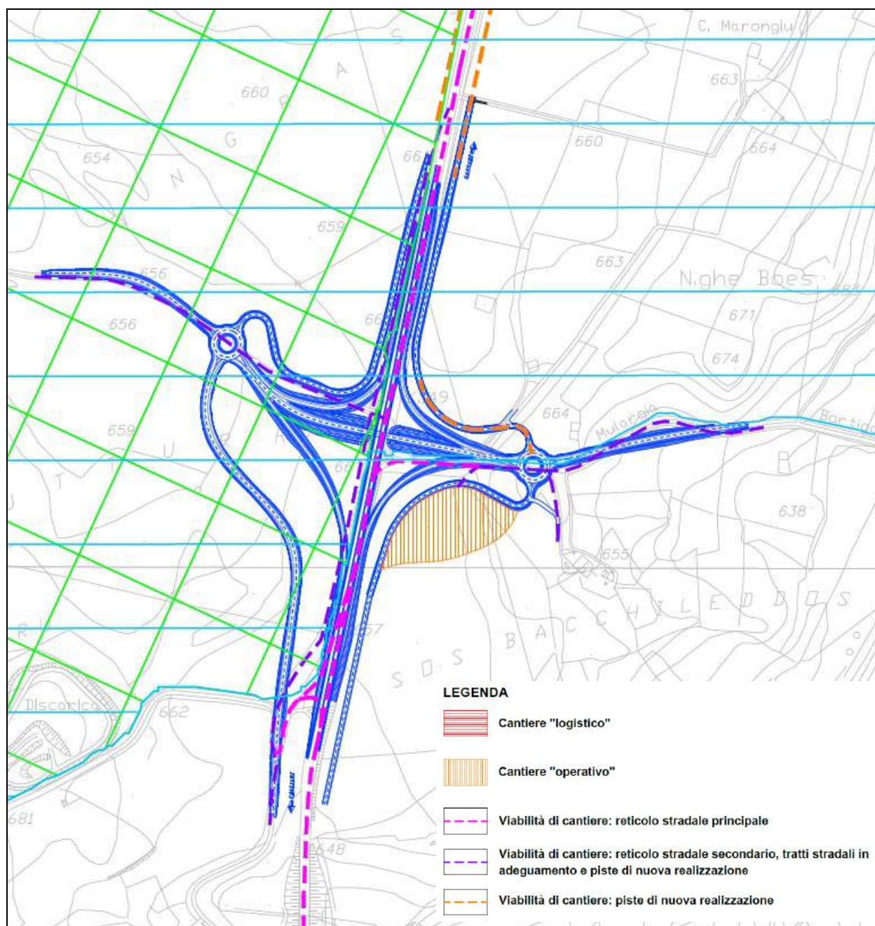
Figura 16 – Alternativa 1 – Aree di cantiere e viabilità di servizio
