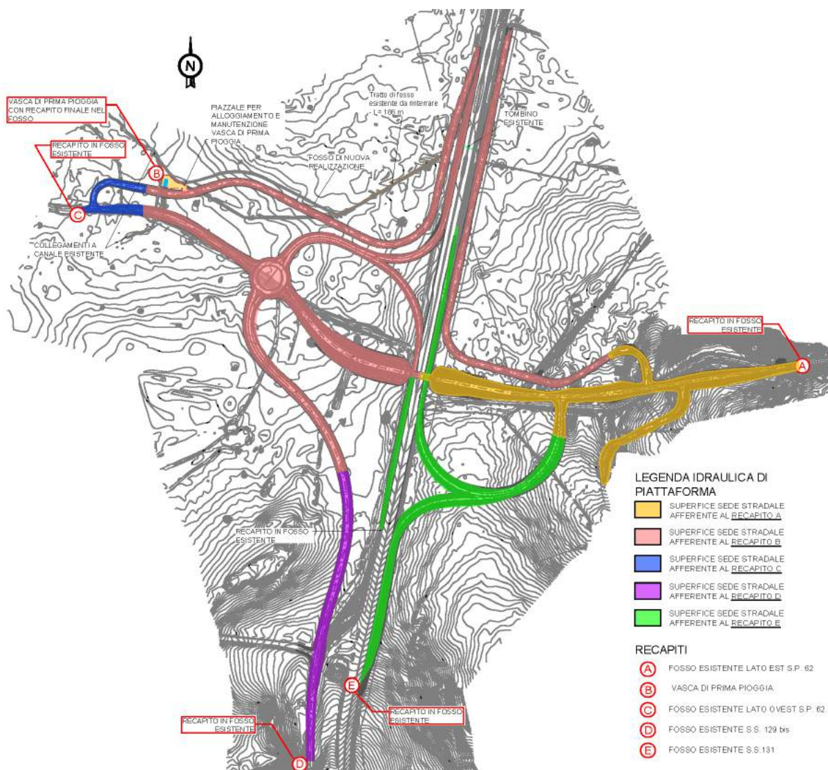
Figura 21 – Soluzione P.D. – Individuazione recapiti acque di piattaforma e relative superfici afferenti
