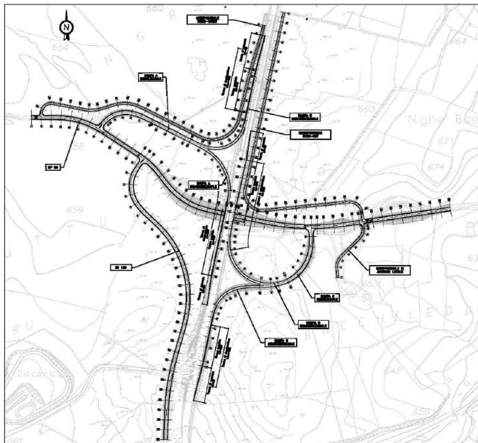
Figura 2 – Svincolo di Mulargia-Macomer da PD
