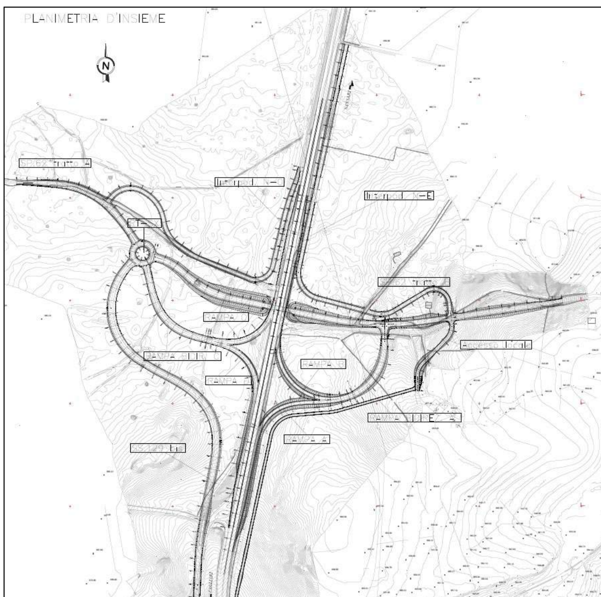
Figura 5 – Svincolo di Mulargia-Macomer Alternativa 2
