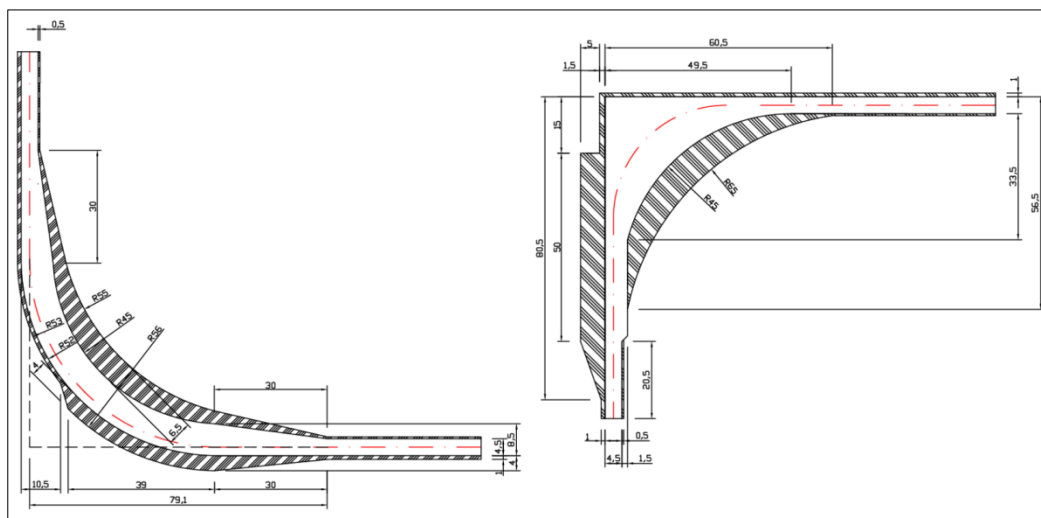
Figura 13 - Particolare realizzazione raccordo strade
