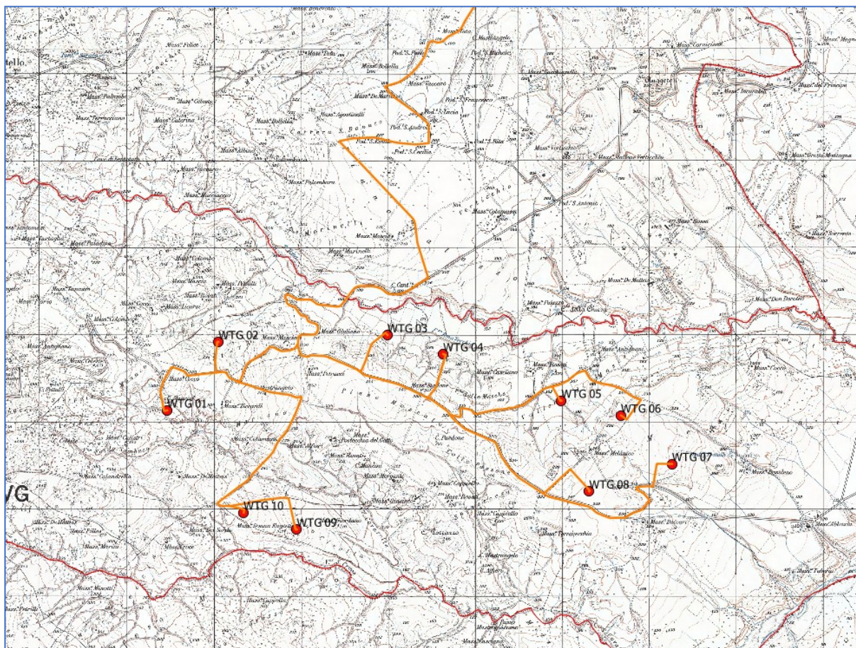
Figura 7 - layout impianto a n.10 aerogeneratori
