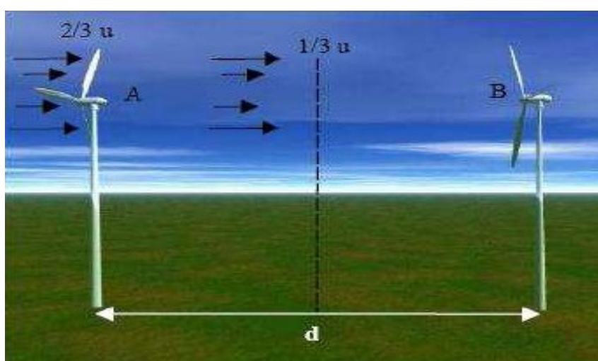
Figura 10 - Effetto di schiera
