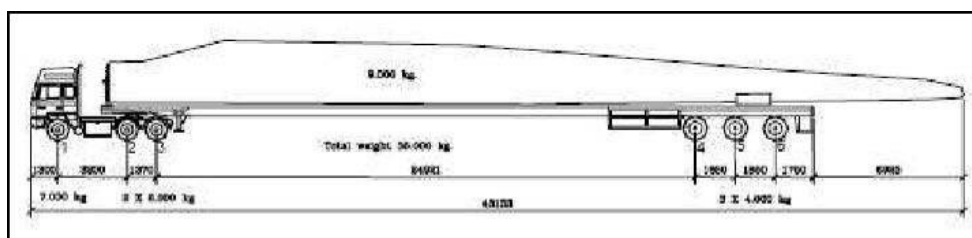
Dimensioni autoarticolato
