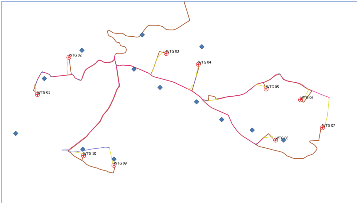
Figura 5 - Sovrapposizione schema layout di partenza a 13 WTG (in blu) e schema definitivo a 10 WTG (in rosso).
