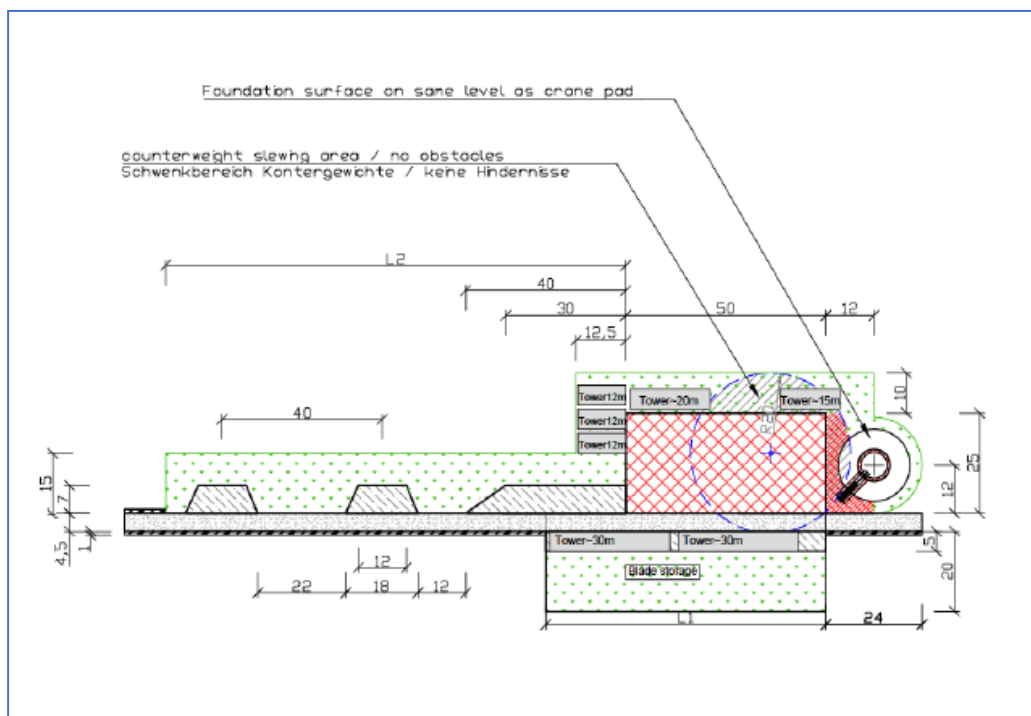
Figura 14 - Piazzola di montaggio
