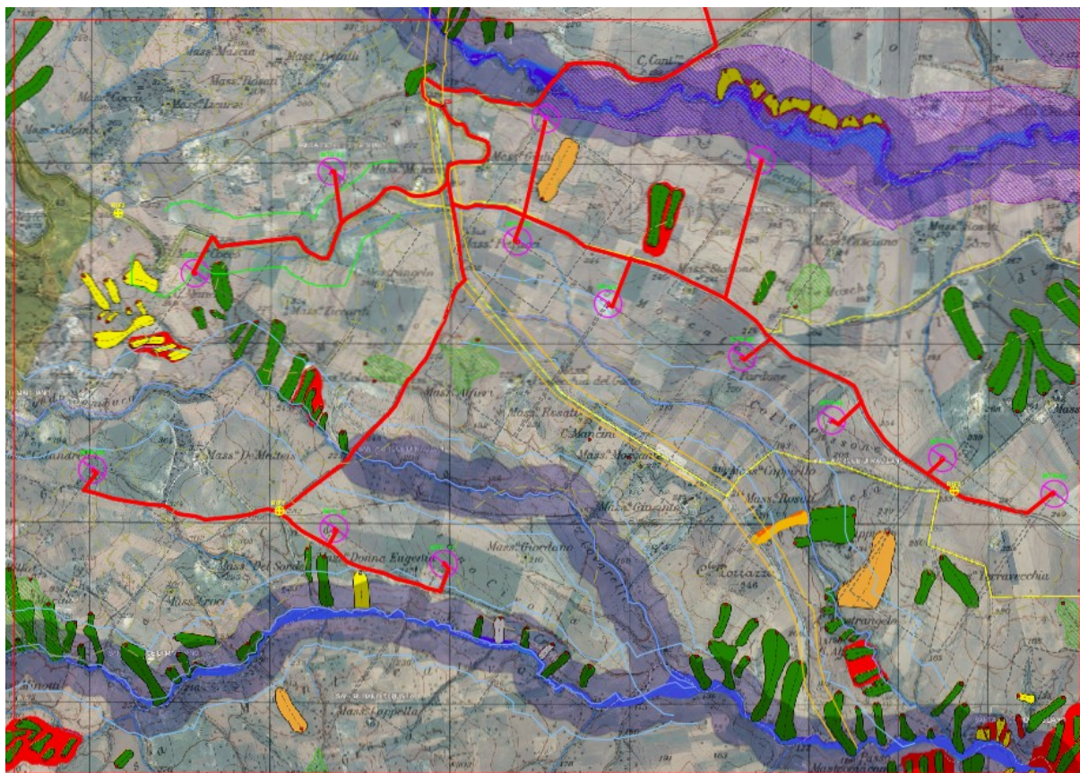
Figura 4 - Ipotesi di layout a 13 aerogeneratori - analisi vincolistica
