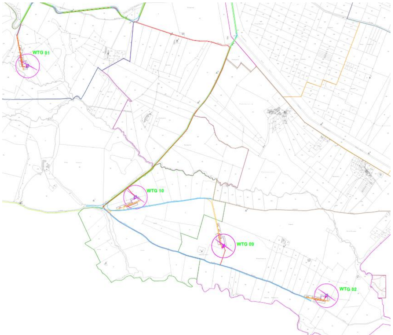
Stralcio Catastale con ubicazione torri eoliche
