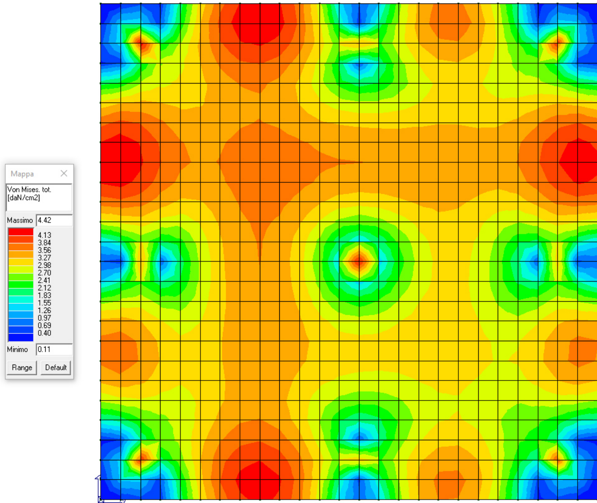
Figura 7 – Von Mises (daN/cm 2 )
