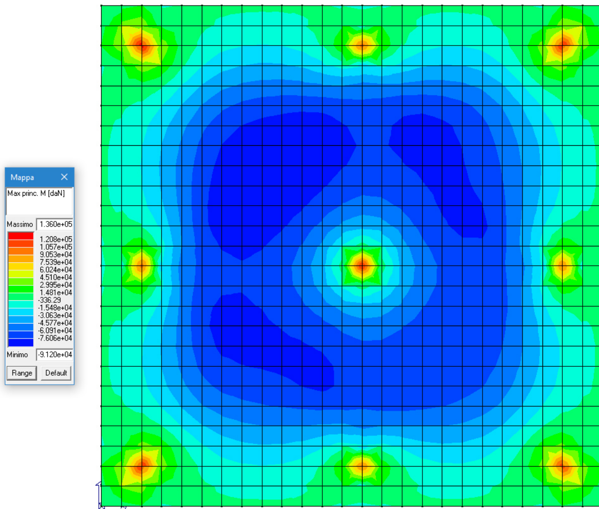
Figura 6 – Von Mises: Max princ. M (daN)
