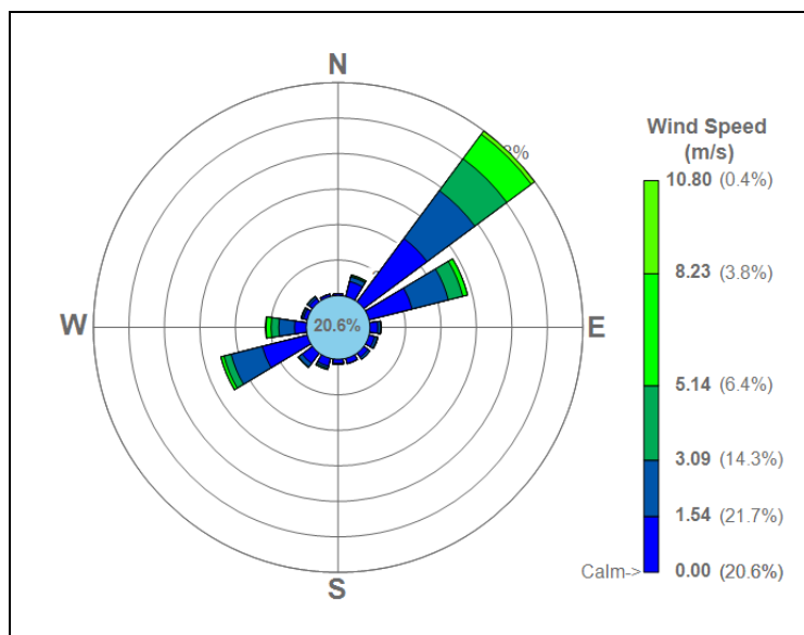
Figura 4-3 Rosa dei venti – 01/01 – 30/06/2021
