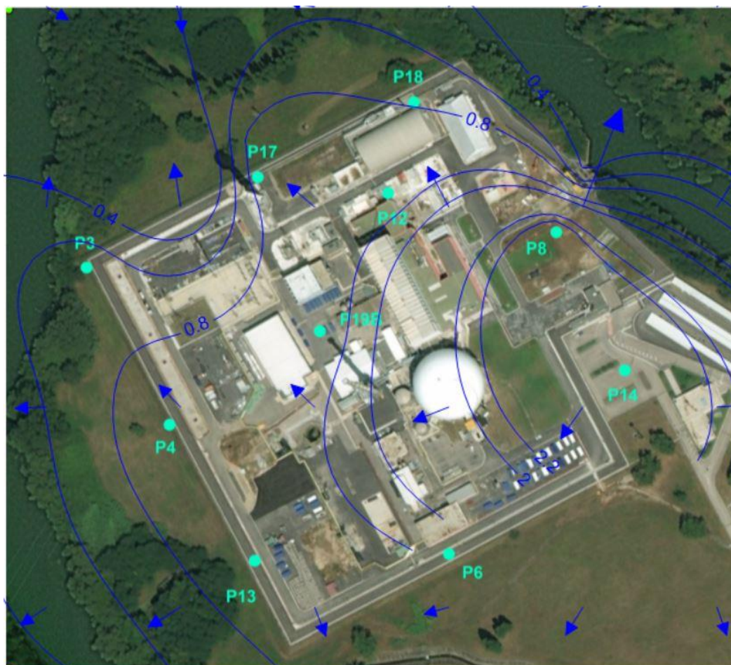
Figura 5-7 - Ubicazione dei punti di monitoraggio acque sotterranee – isofreatiche di maggio 2021
