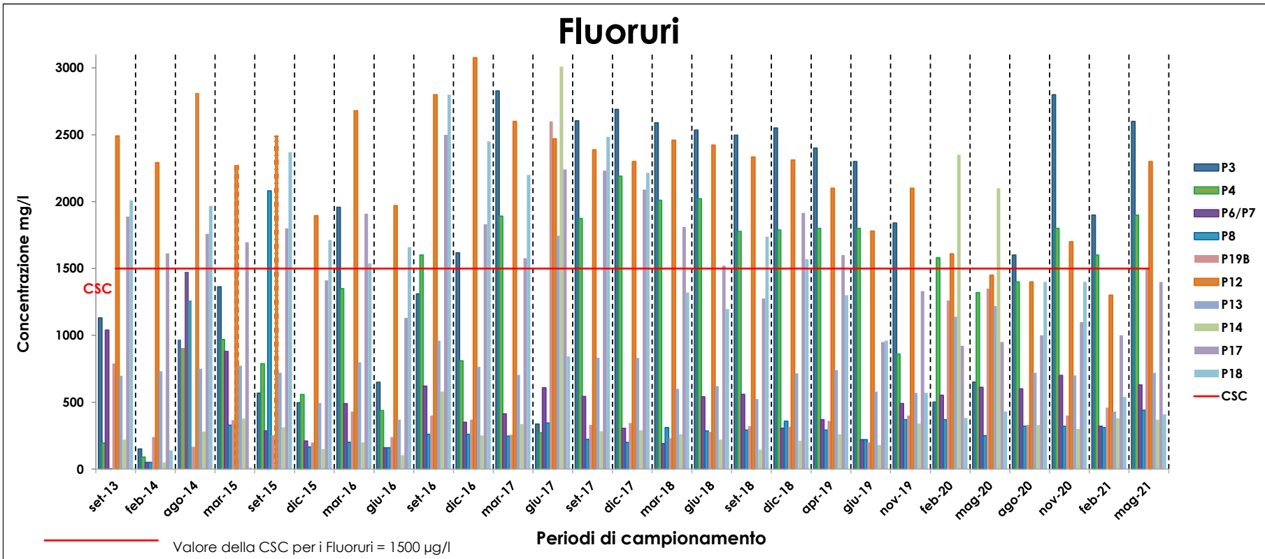
Figura 5-8 - Andamento nel tempo del parametro fluoruri nelle acque sotterranee
