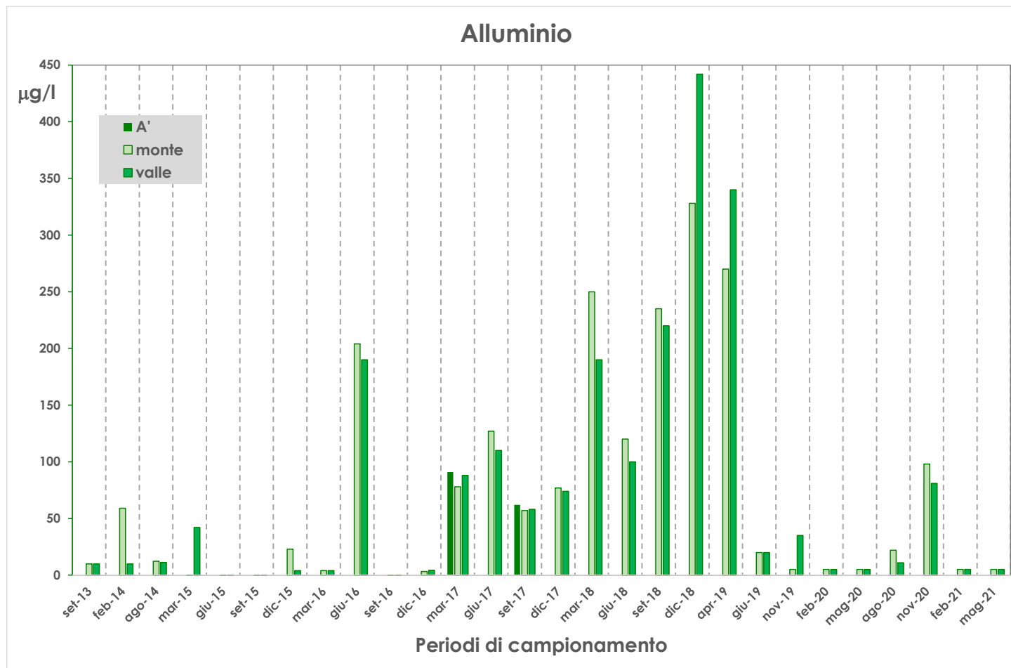
Figura 5-3 – Acque superficiali: confronto tra i valori di monte e valle da settembre 2013 fino a maggio 2021 - alluminio
