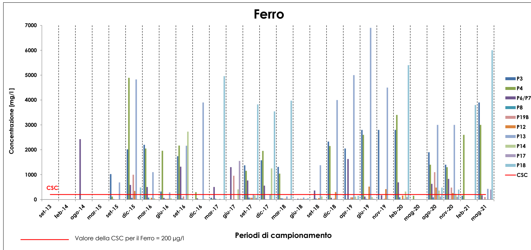
Figura 5-10 - andamento del parametro ferro nelle acque sotterranee
