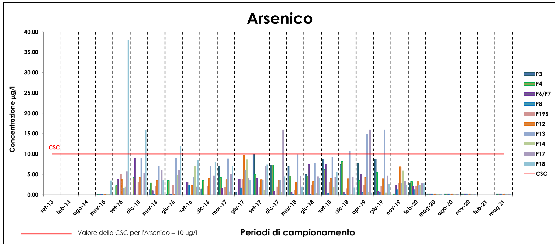
Figura 5-9 - andamento nel tempo del parametro arsenico nelle acque sotterranee
