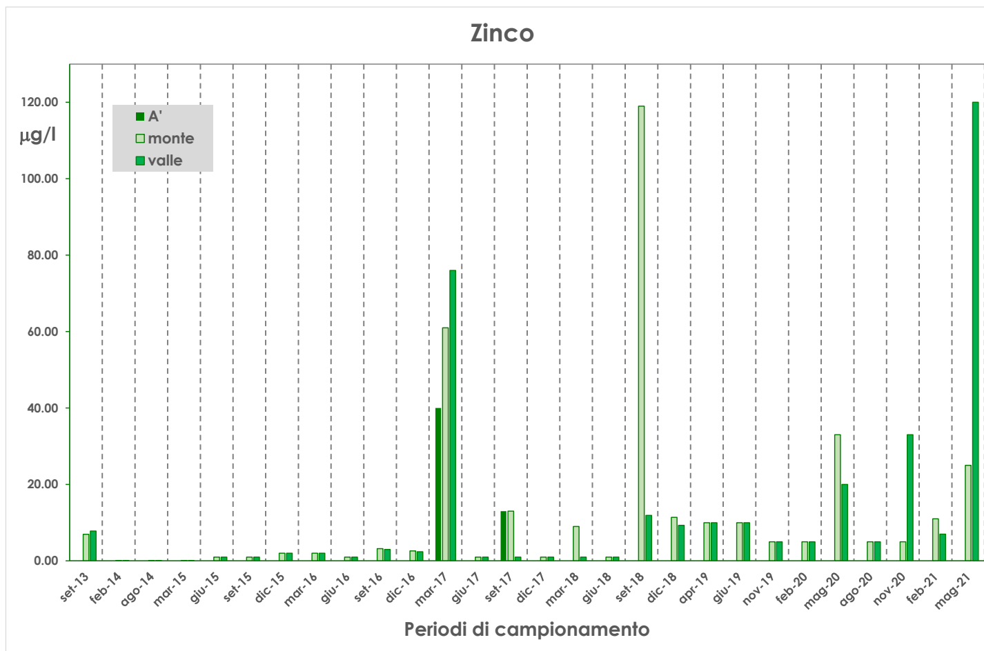
Figura 5-4 - Acque superficiali: confronto tra i valori di monte e valle da settembre 2013 fino a maggio 2021 - zinco
