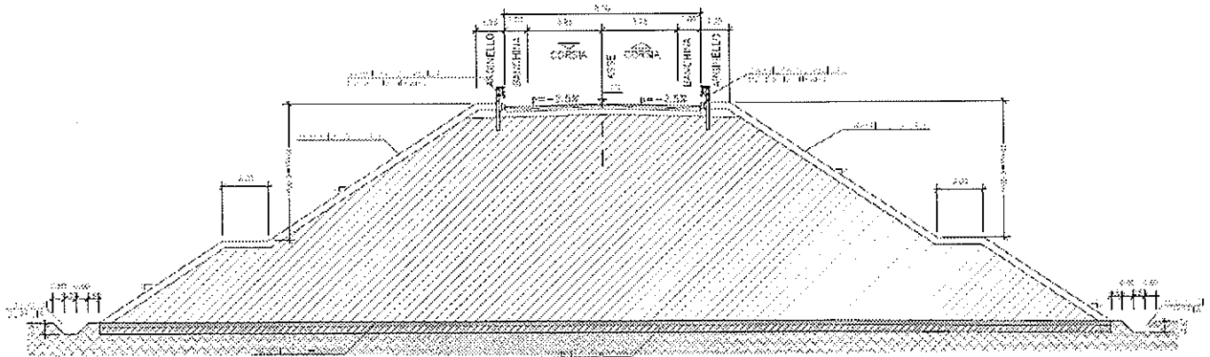
Figura 1 – Sezione tipo cat. F2 (D.M. 5/11/2001) per H>6.00m
