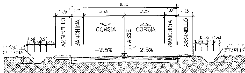
Figura 2– Sezione tipo cat. F2 (D.M. 5/11/2001) per H≤6.00m
