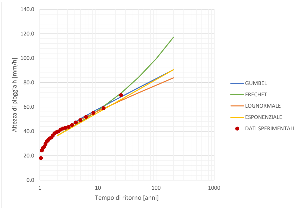
Figura 9: Confronto delle curve di possibilità pluviometriche con i dati sperimentali osservati, stazione di Gragnano.
