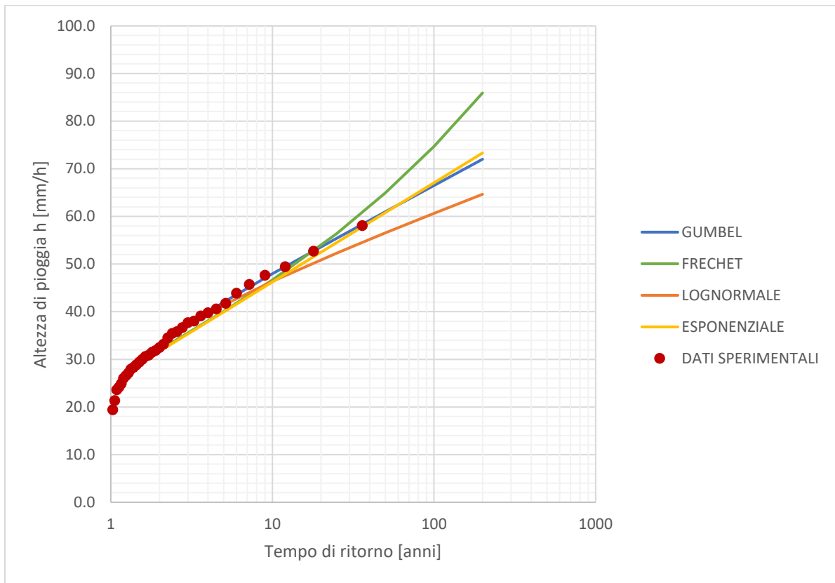
Figura 10: Confronto delle curve di possibilità pluviometriche con i dati sperimentali osservati, stazione di Mercato San Severino.
