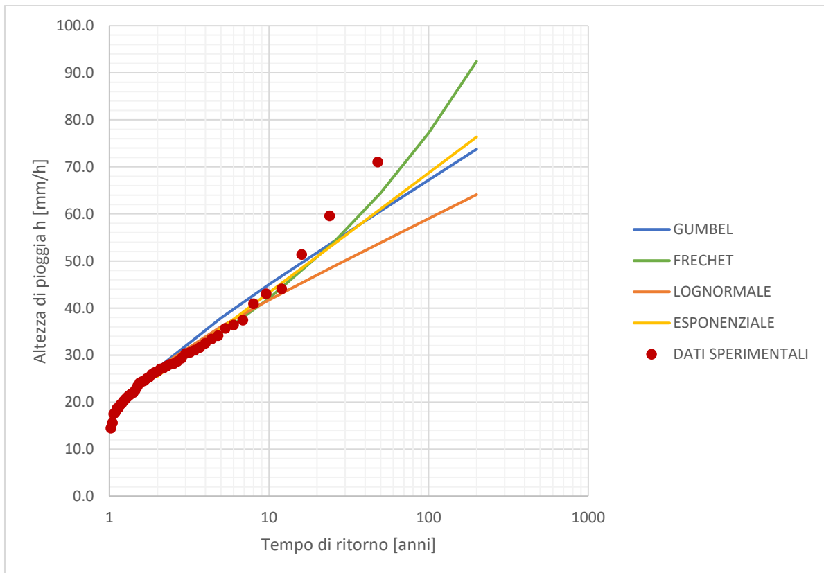
Figura 11: Confronto delle curve di possibilità pluviometriche con i dati sperimentali osservati, stazione di Sarno.
