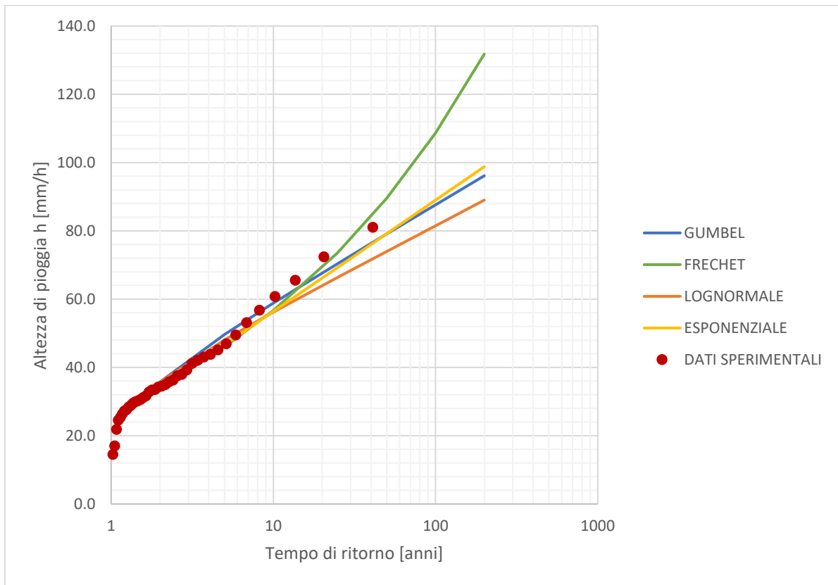
Figura 8: Confronto delle curve di possibilità pluviometriche con i dati sperimentali osservati, stazione di Cava dei Tirreni.
