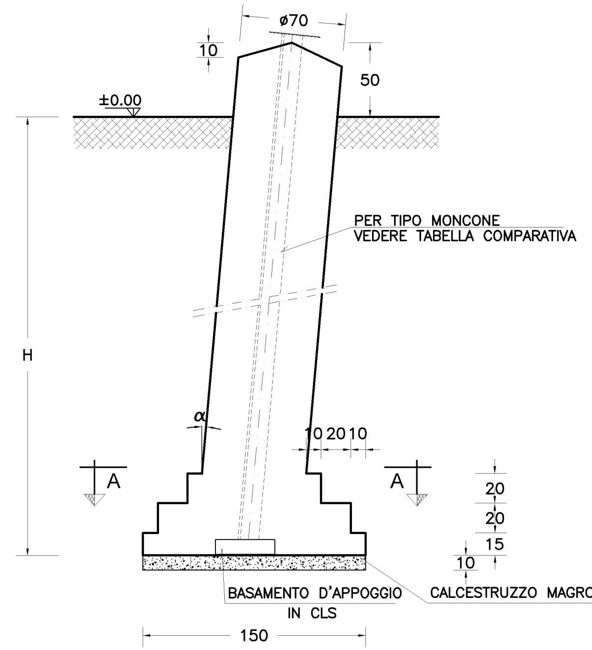
SEZIONE B-B 1:25
