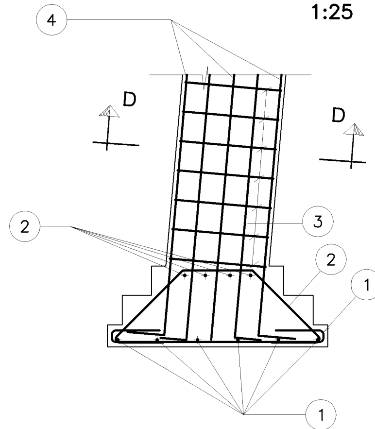
SEZIONE C-C 1:25
