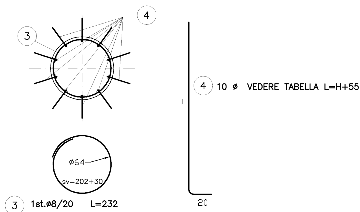
SEZIONE D-D 1:25
