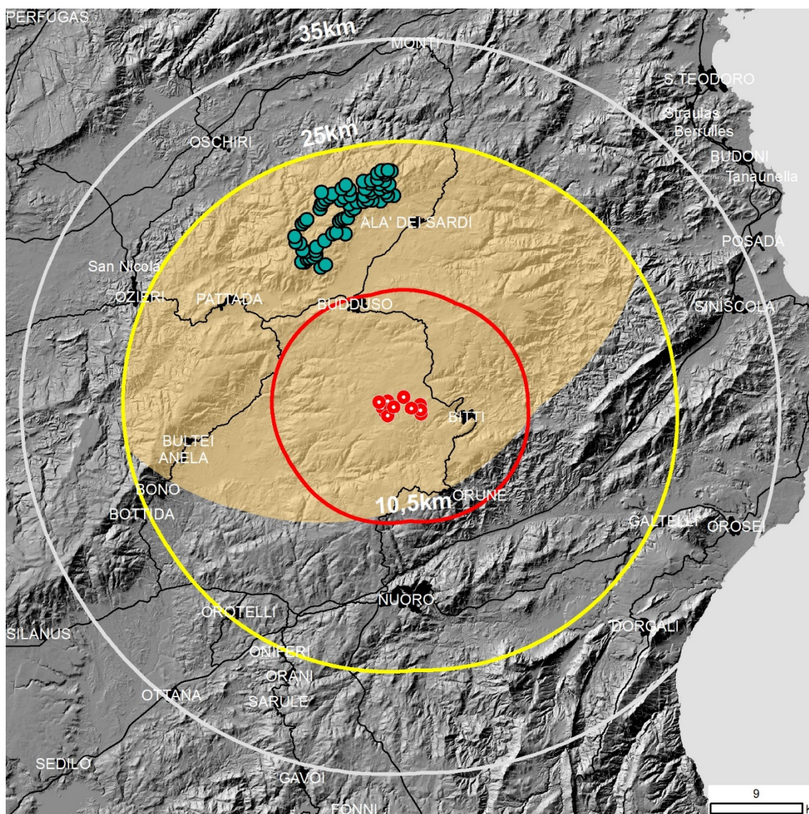
Figura 7 – In ocra sono rappresentate le aree ricomprese nel calcolo dell’ICS secondo l’assunto 3 (in rosso l’impianto in progetto in verde l’impianto esistente in relazione visiva)
