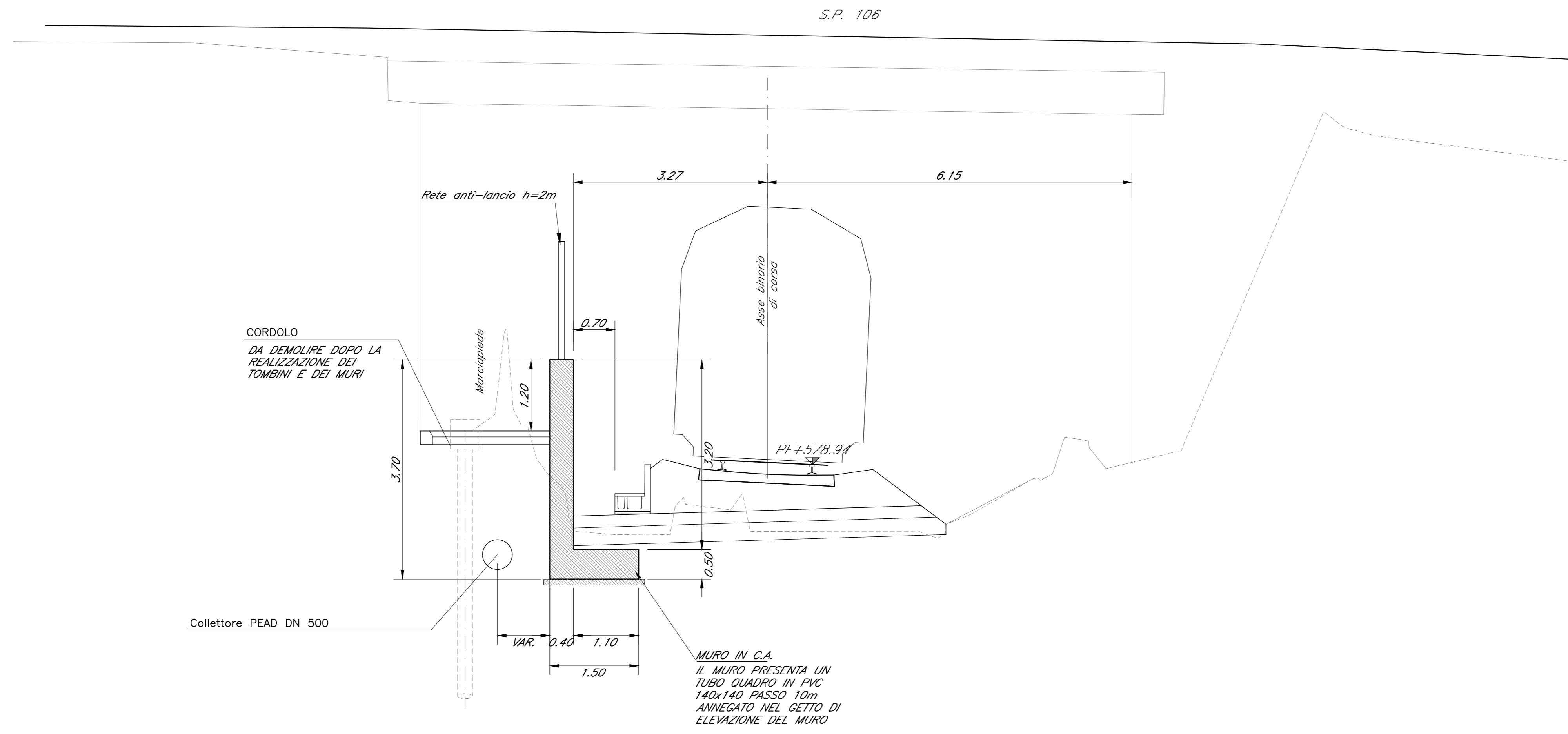
PROSPETTO MURO B-B SCALA 1:50
