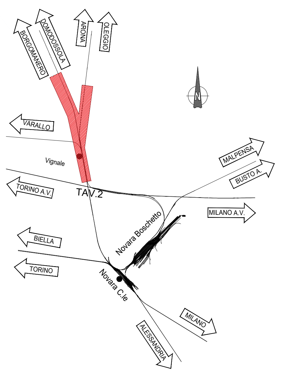
Piantina chiave
