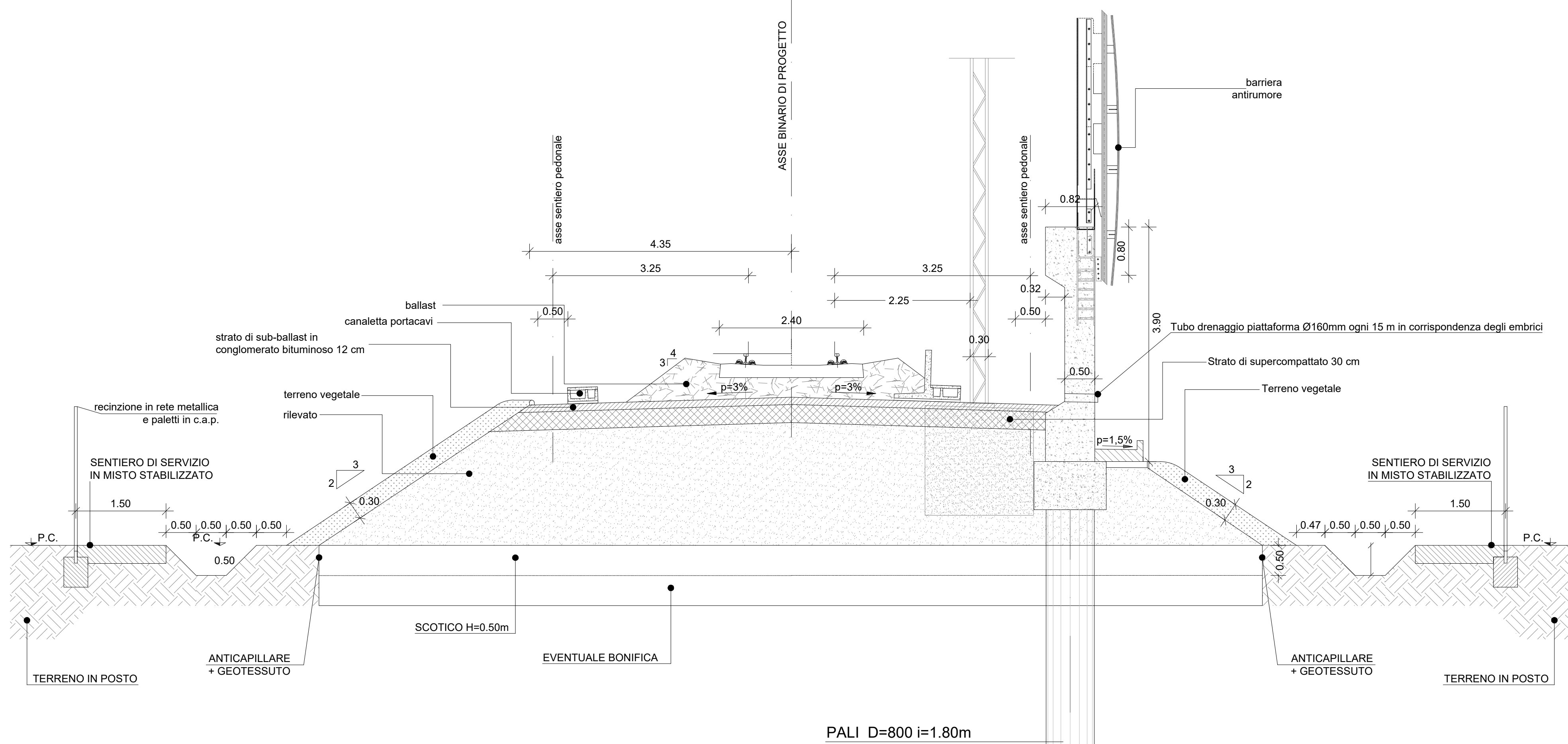
SEZIONE TIPO SINGOLO BINARIO NUOVO PIATTAFORMA CON BARRIERA ANTIRUMORE E MURI DI RECINZIONE IN RILEVATO scala 1:50
